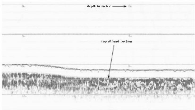
Figuur D-22 Locatie D5 – Dichtheidsprofiel (linker bovenhoek), radiografie (rechter bovenhoek), in situ foto van het staal (linker benedenhoek) en echogram (rechter benedenhoek) voor kern D5-B-6, opgenomen bij volle vloedstroom.
