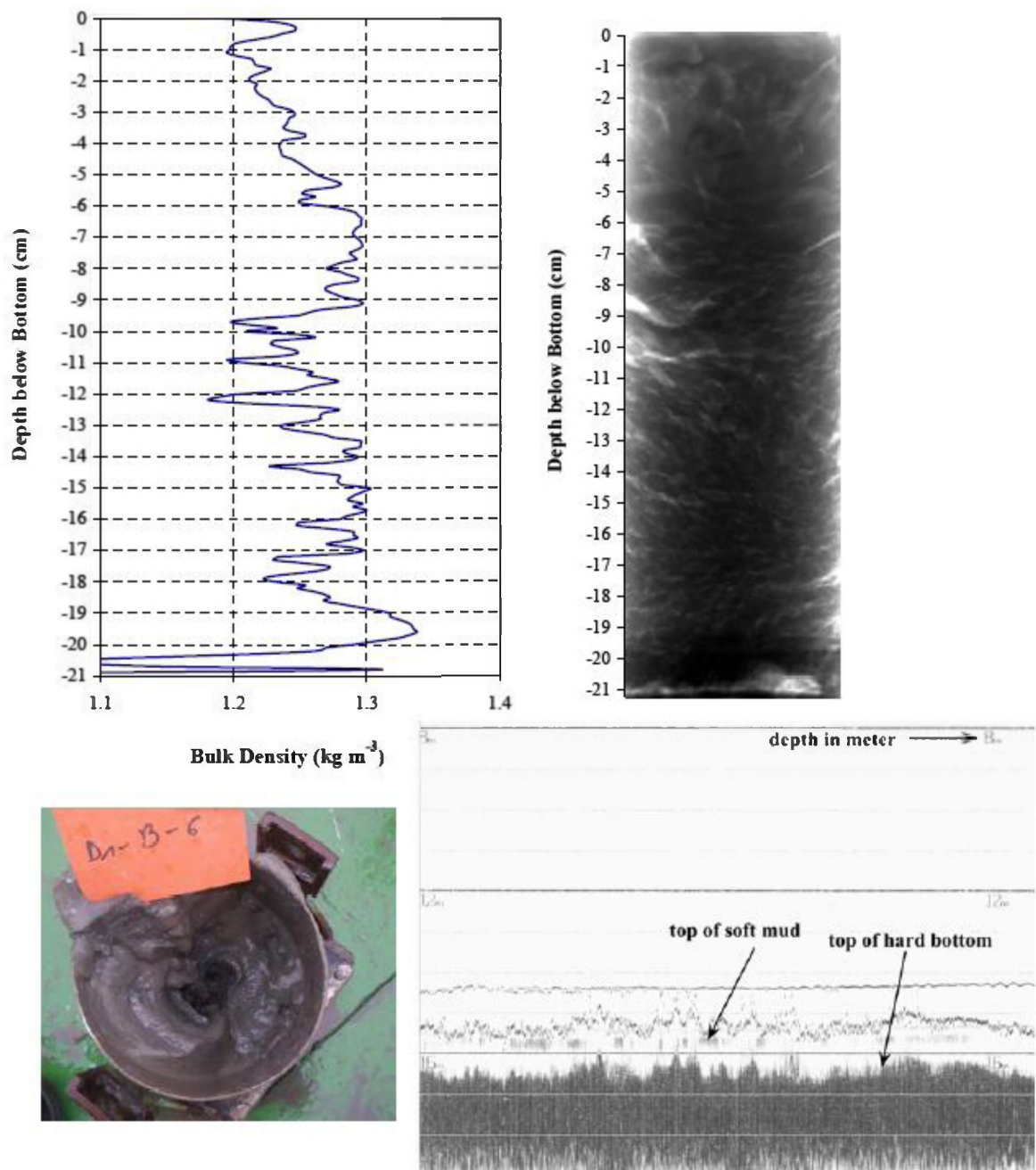
Figuur D-6 Locatie D1 – Dichtheidsprofiel (linker bovenhoek), radiografie (rechter bovenhoek), in situ foto van het staal (linker benedenhoek) en echogram (rechter benedenhoek) voor kern D1-B-6, opgenomen bij volle ebstroom.
