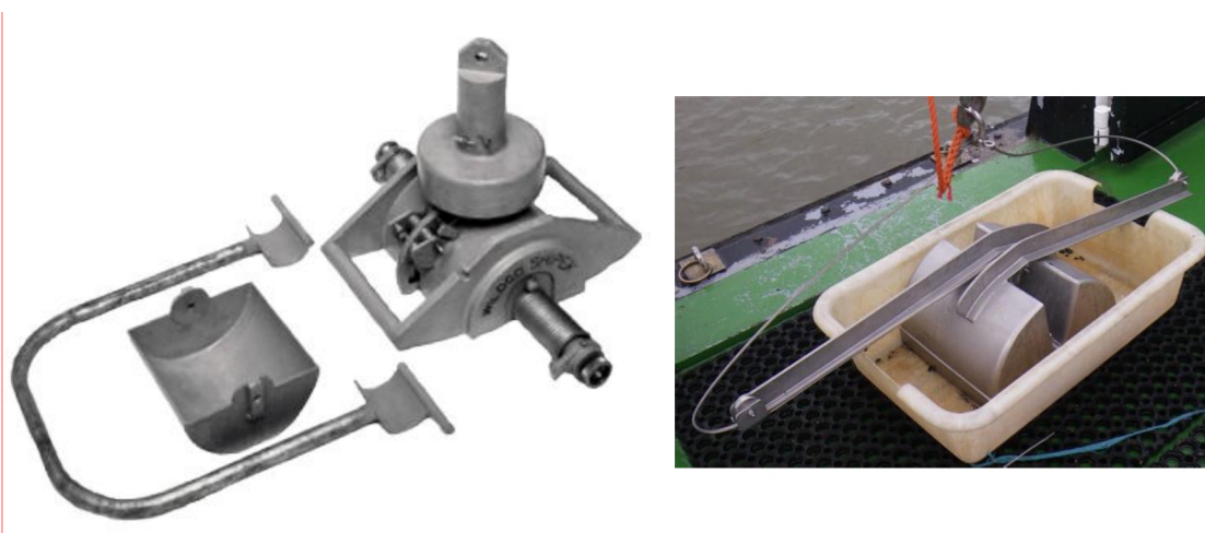
Figuur 2-1 Links: Shipek bodemgrijper; rechts: Van Veen grijper
