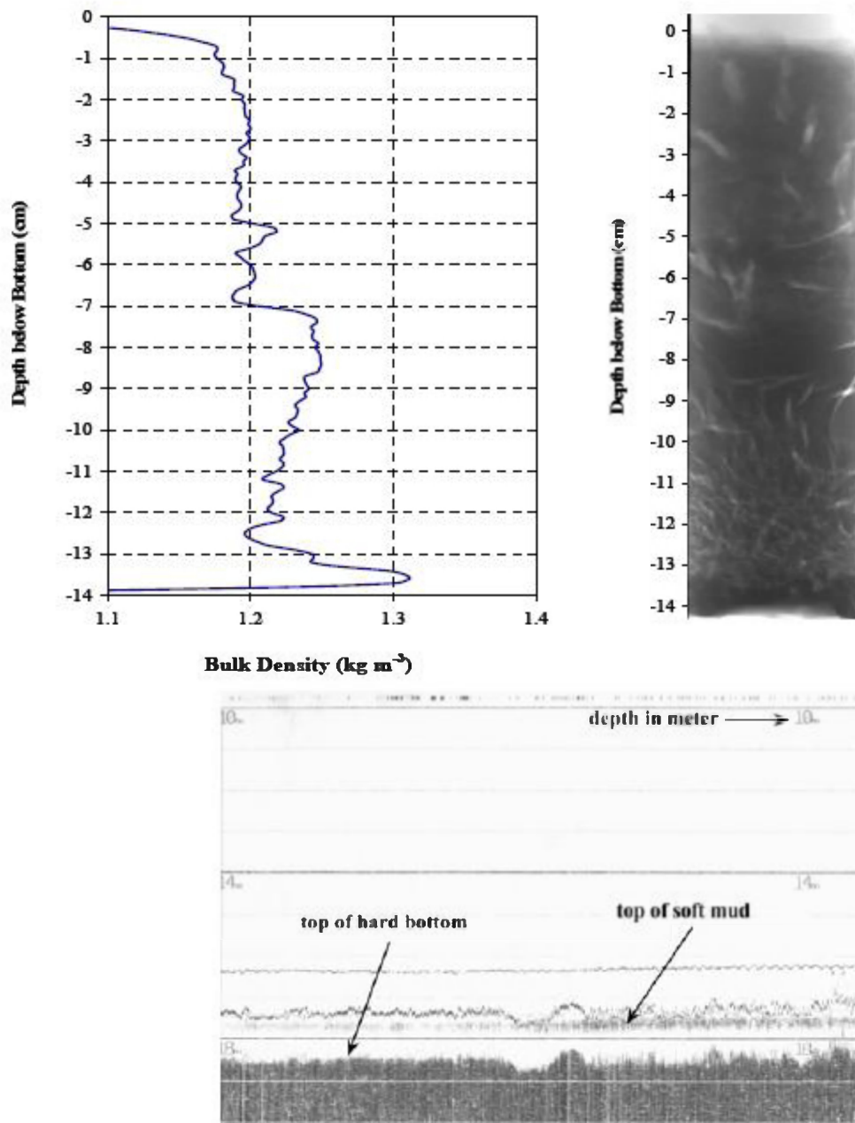
Figuur D-3 Locatie D1 – Dichtheidsprofiel (linker bovenhoek), radiografie (rechter bovenhoek), en echogram (beneden midden) voor kern D1-B-3, opgenomen bij stroomstilstand na vloed
