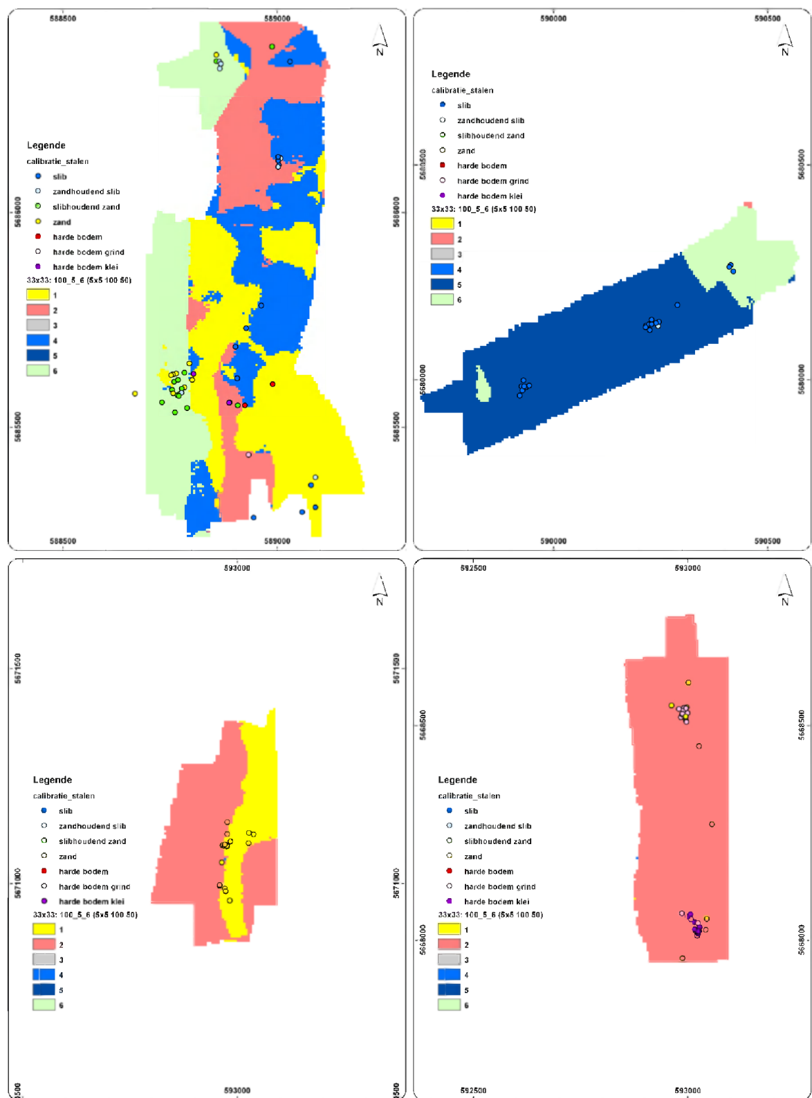
Figuur F-4 Vergelijking calibratiekaart 33x33_6 klassen en calibratiestalen. Linksboven: referentiezones D3 (zandhoudend slib) en D4 (slibhoudend zand), rechtsboven: referentiezone D1 (slib), linksonder: referentiezone D5 (zand), rechtsonder referentiezone D2 (harde bodem).
