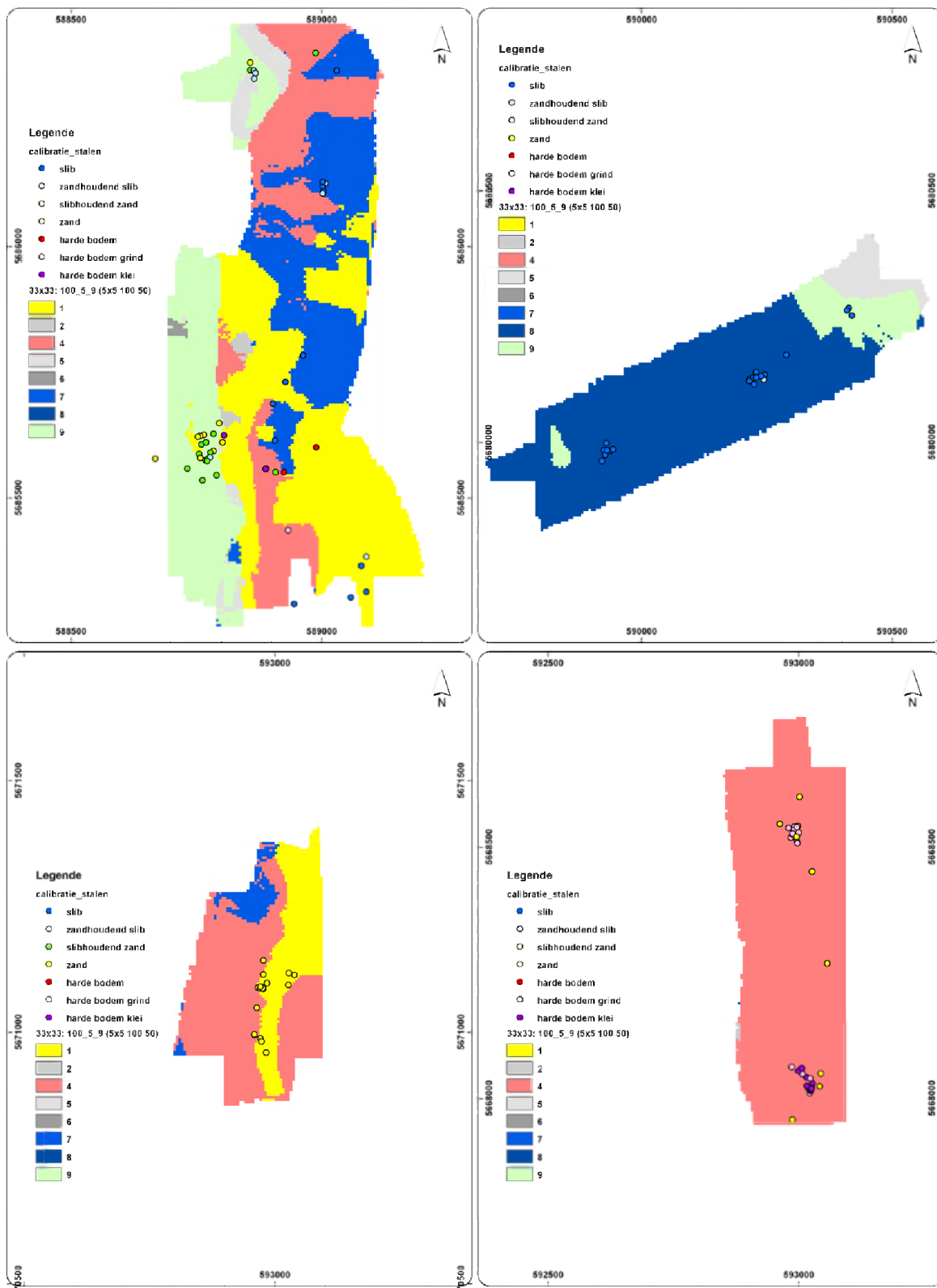
Figuur F-6 Vergelijking calibratiekaart 33x33_9 klassen en calibratiestalen. Linksboven: referentiezones D3 (zandhoudend slib) en D4 (slibhoudend zand), rechtsboven: referentiezone D1 (slib), linksonder: referentiezone D5 (zand), rechtsonder referentiezone D2 (harde bodem).
