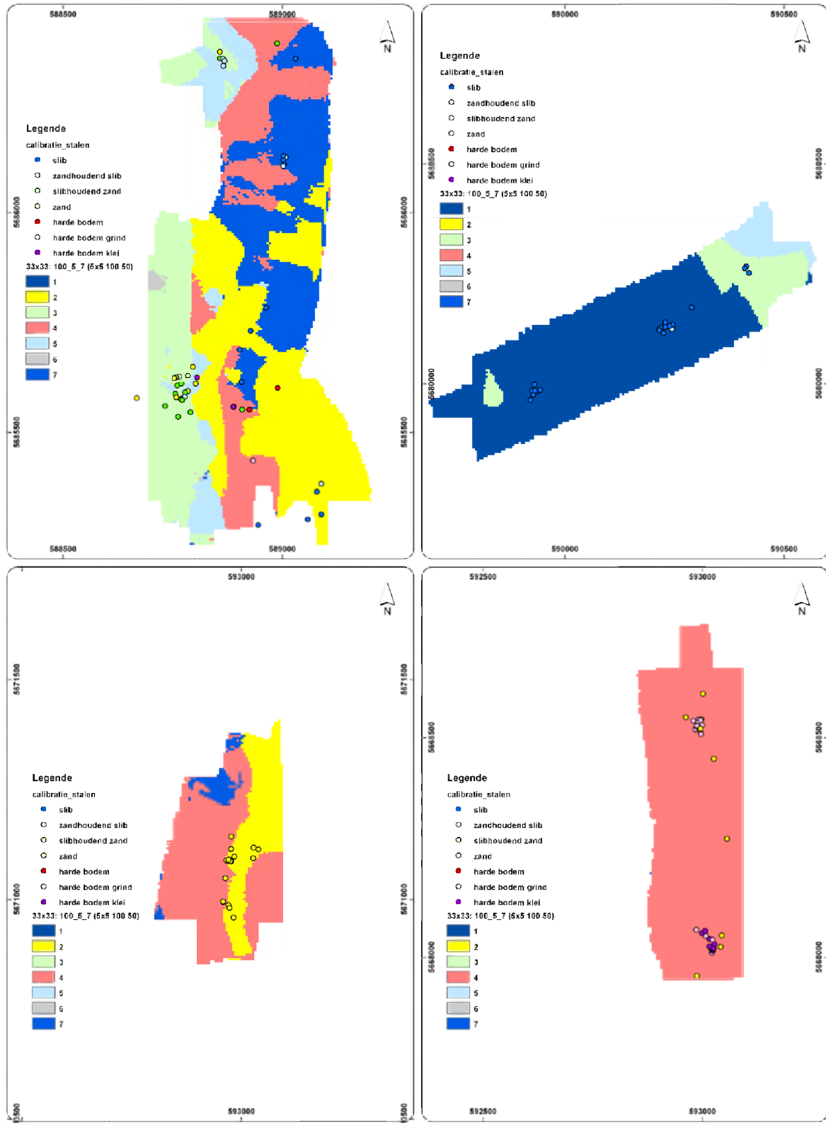
Figuur F-5 Vergelijking calibratiekaart 33x33_7 klassen en calibratiestalen. Linksboven: referentiezones D3 (zandhoudend slib) en D4 (slibhoudend zand), rechtsboven: referentiezona D1 (slib), linksonder: referentiezona D5 (zand), rechtsonder referentiezona D2 (harde bodem).
