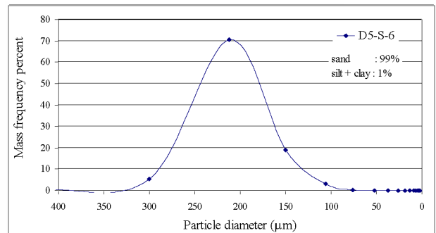
Figuur C-22 Referentiezone D5: sediment korrelgrootteverdeling van de Shipek samples bij laagwaterkentering
