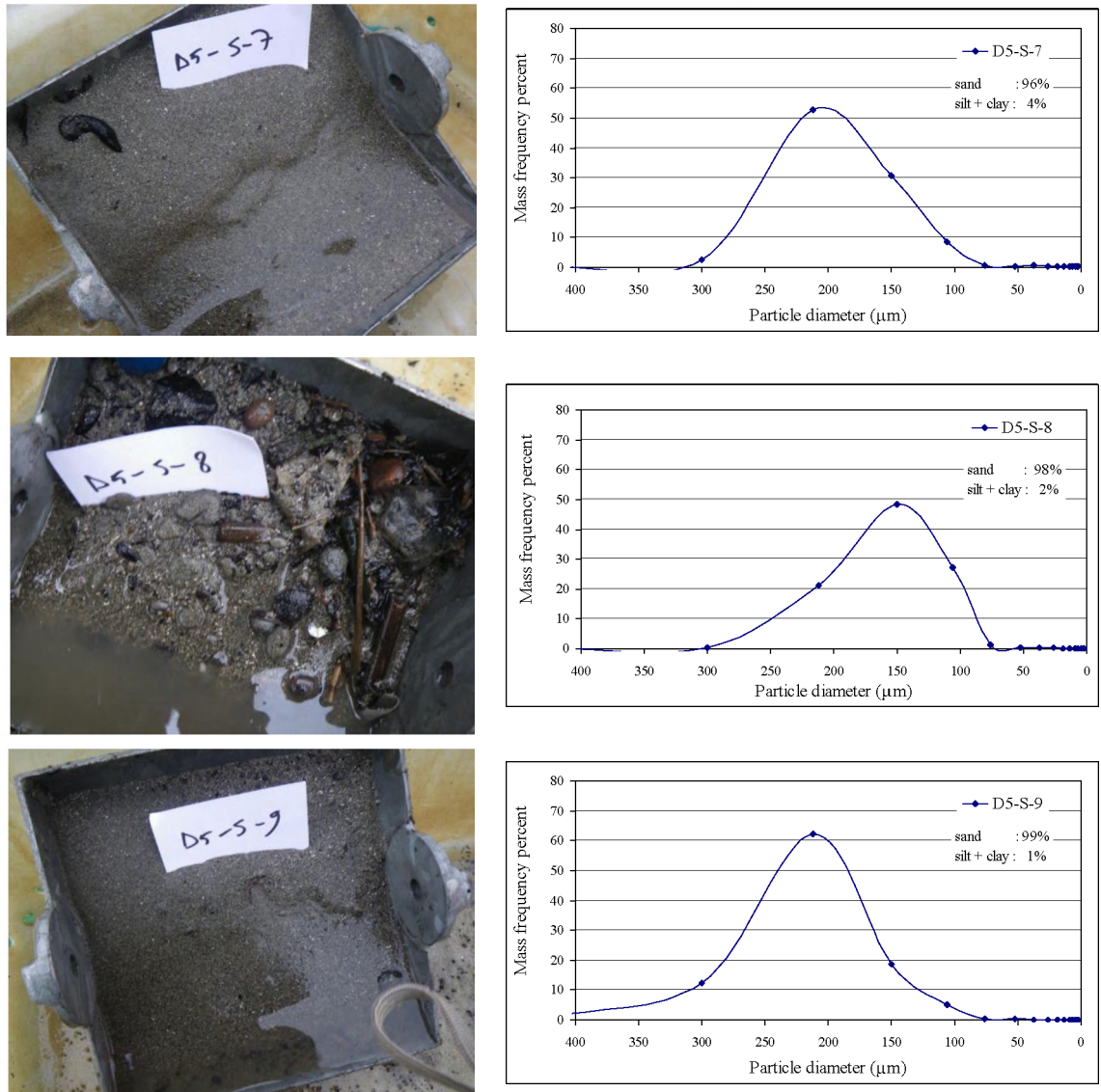
Figuur C-23 Referentiezone D5: sediment korrelgrootteverdeling van de Shipek samples bij volle vloed
