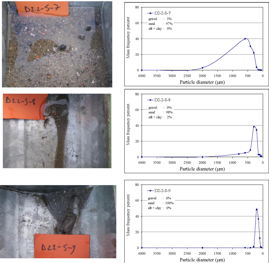
Figuur C-12 Referentiezone D2.2: sediment korrelgrootteverdeling van de Shipex samples bij volle eb
