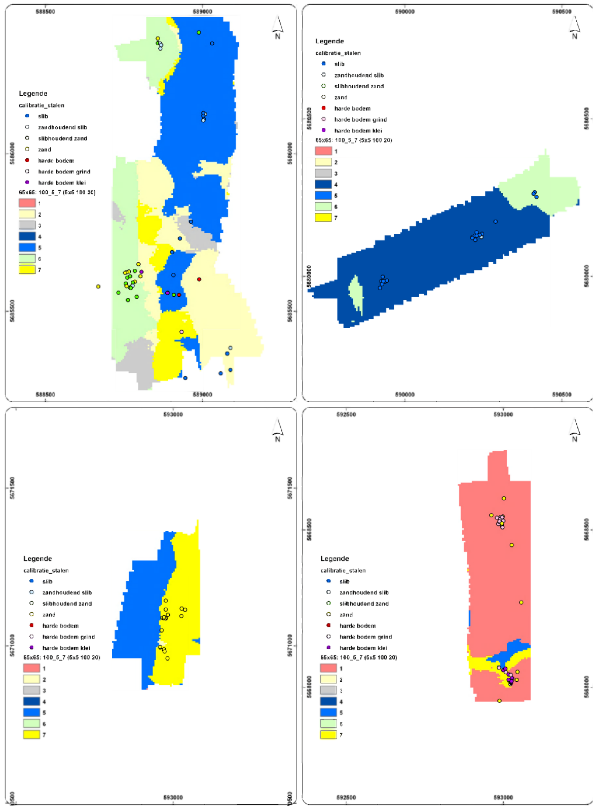
Figuur F-2 Vergelijking calibratiekaart 65x65_7 klassen en calibratiestalen. Linksboven: referentiezones D3 (zandhoudend slib) en D4 (slibhoudend zand), rechtsboven: referentietone D1 (slib), linksonder: referentietone D5 (zand), rechtsonder referentietone D2 (harde bodem).
