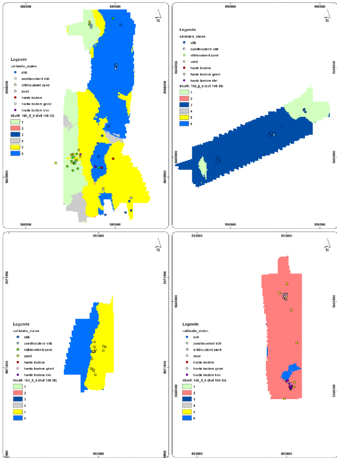
Figuur F-1 Vergelijking calibratiekaart 65x65_6 klassen en calibratiestalen. Linksboven: referentiezones D3 (zandhoudend slib) en D4 (slibhoudend zand), rechtsboven: referentiezone D1 (slib), linksonder: referentiezone D5 (zand), rechtsonder referentiezone D2 (harde bodem).
