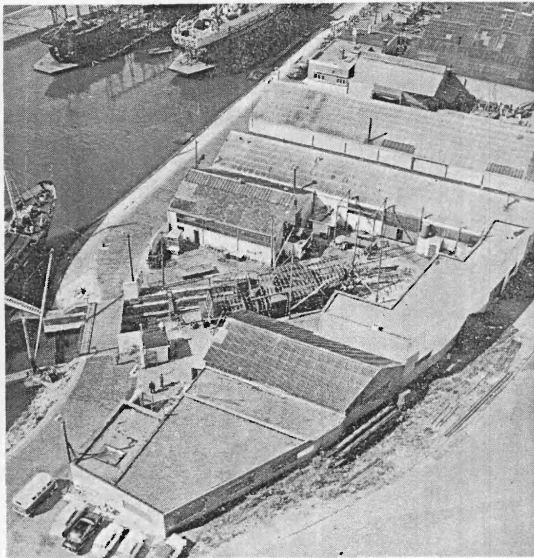
Zicht op de werf Seghers. Een stalen vaartuig is in opbouw. Bovenaan een gedeelte van de sloopways. Foto genomen vanuit de vuurtoren. ( cliché Seghers)
