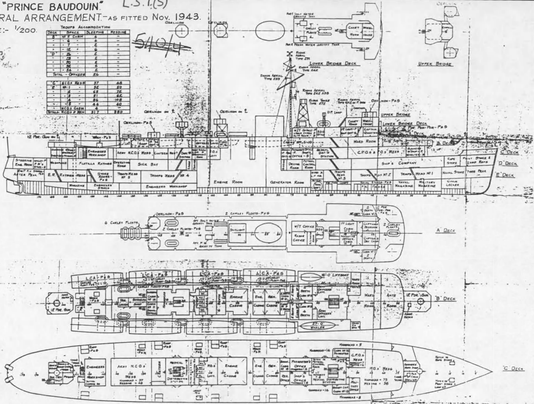
H.M.S. Prince Baudouin. Algemeen plan, bovenste dekken, gemaakt door Green & Sillyweir in november 1943
