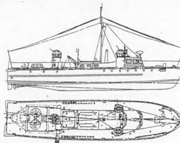
Figuur nr. 40: Thornycroft 67 ft High Speed Launch. Ontworpen door John I. Thornycroft & Co. Ltd., Hampton. Afmetingen : l.o.a. 20,44 m x br. 4,58 m x dpg. 1,22 m 2 motoren van 650 pk, snelheid 24,7 knoop. Autonomie : 600 mijl. Bewapening : 3 koepels met 2 m.g. .303 duim.
