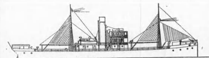
Fig. nr. 66. Tilburylijn. Lijntekening van het s.s. Emeraude, (ex- Rio Prado), aangekocht in 1920. Gebouwd in 1903 door Graig-Taylor te Stockton, Engl. Het schip zonk op 30 juni 1945 in het Kanaal.
