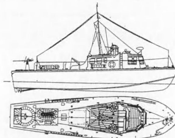
Figuur nr. 41: British Power Boat Co. Type 3, "Hants and Dorset" 68 ft R.A.F. High Speed Launch. Ontworpen door British Power Boat Co., Hythe, 1943. Afmetingen : l.o.a. 20,75 m x br. 5,04 m x dpg. 1,22 m 3 motoren van 500 pk, snelheid 28 knoop, autonomie 580 mijl Bewapening : 1 x 20 mm, 2 koepels met 2 m.g.'s .303 inch.
