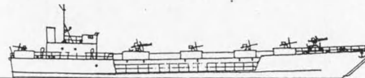
Figuur nr.35 LCF(4). Landing Craft Anti-Aircraft, Type 4. Omgebouwde LCT(4), bewapend met luchtdoelkanonnen voor verdediging tegen luchtaanvallen van de troepen op de stranden en ontschepingsvloot. Bewapening : 4 x 1 2-pond en 8 x 1 20 mm A.A. kanonnen. Bemanning : 66. Achterveertig vaartuigen in dienst genomen door de R.N.
