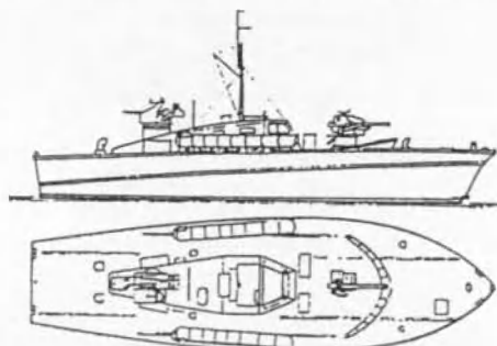
Figuur nr. 39: British Power Boat Motor Torpedoboot. Ontworpen door British Power Boat Co., Hythe. Afmetingen : l.o.a. 21,88 m x br. 6,28 m x dpg. achter 1,68 m. Waterverplaatsing 51,6 ton. 3 motoren Packard van 1200 pk. Snelheid 39 knoop, autonomie 600 mijl bij 15 knoop. Bewapening : 1 x 6 pond kanon, 1 x 20 mm kanonnen in aangedreven koepels. 2 x 18" torpedo's Bemanning : 17. Gebouwd 1942-45, aantal 80.
