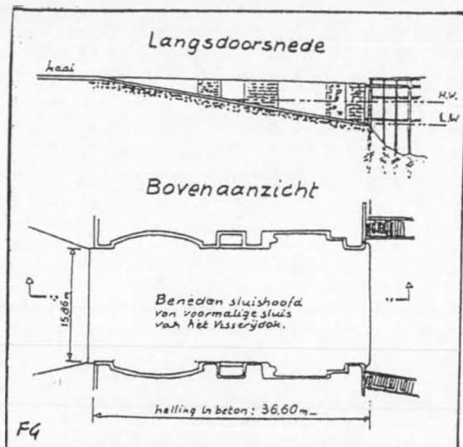
Fig. nr. 26. Oostende 1944, LST-helling nr. 1 (LST ramp no. 1). Inplanting, bovenaanzicht en langsdoorsnede van de door de Britten gebouwde landingsinstallatie tussen de beneden sluishoofden van de voormalige Visserijsluis. De helling bestaat ten heden dagen nog, (december 2005).
