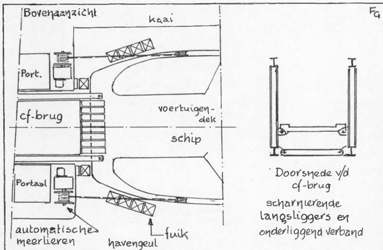
Figuur nr. 60. Haven Oostende, in- en ontschepingsbrug nr. I. Concept principes. Fuik, oplegging brug op schip en meren.
