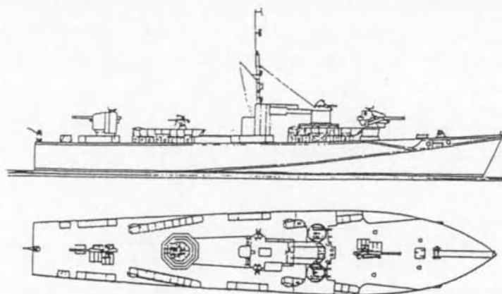
Figuur nr. 38: Fairmile Type D Motor Torpedoboot. Ontworpen door de Britse Admiraliteit, constructie in hout. Afmetingen : l.o.a. 30,08 m x br. 6,48 m x dpg. achter 1,56 m. Waterverplaatsing 105 ton. Vier motoren Packard van 1250 pk. Snelheid 31 knoop, autonomie 1200 zeemijl bij 10 knoop. Bewapening : 2 x 16 pond kanon, 1 x 20 mm kanon, 2 x 2 m.g.'s .50" in aangedreven koepels. 4 x 18" torpedo's, 2 dieptebommen. Bemanning : 30. Gebouwd : 1942-44, aantal : 210 boten.
