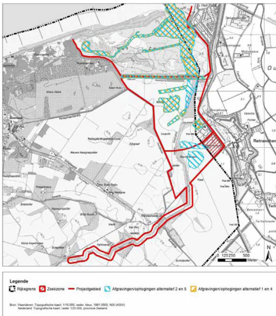
Figuur 4-1: Geplande afgravingen en ophogingen in het bestaande en uitgebreide Zwin
