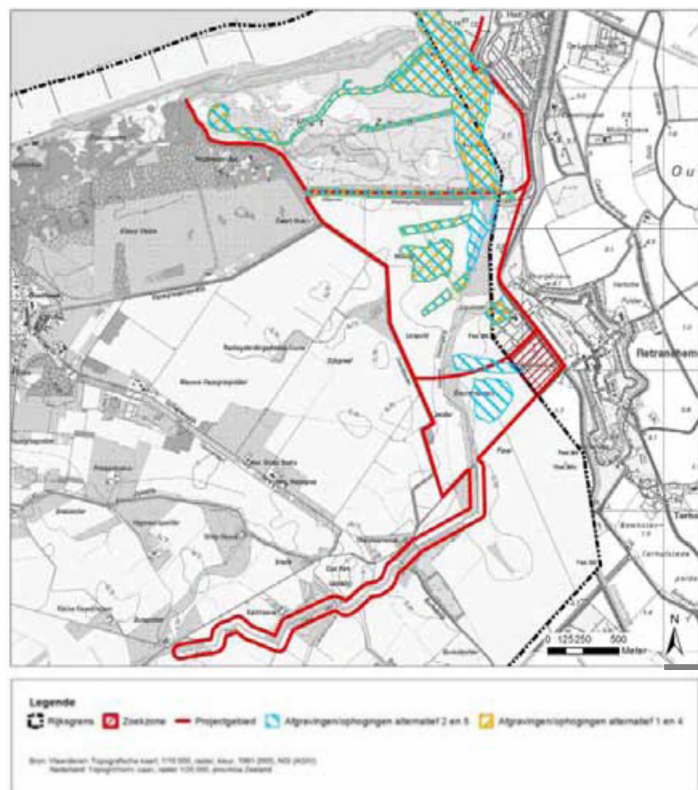
Figuur 5-1: Overzicht van de af te graven en op te hogen zones in het huidige Zwin en de Willem-Leopoldpolder
