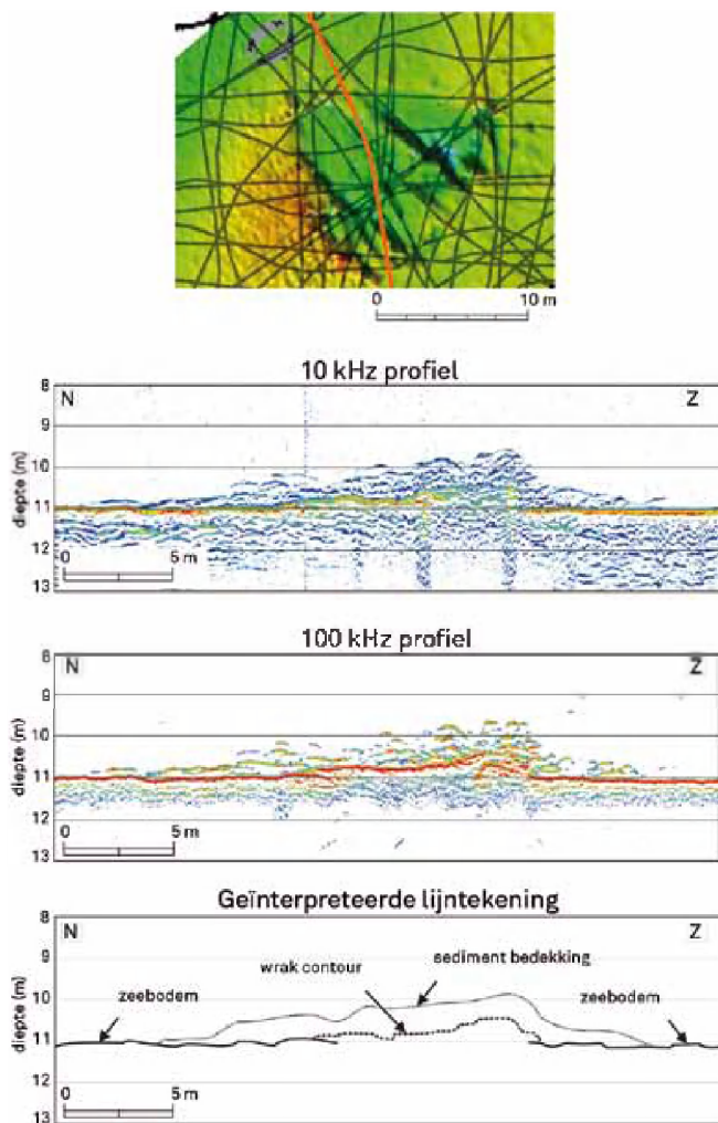
FIG. 12. Locatie van het profiel (in oranje aangegeven) en seismisch profiel 7 (diepte onder wateroppervlak in meter). Location of profile (in orange) and seismic profile 7 (depth under water in meters).
