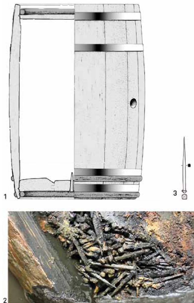
FIG. 51 1: reconstructietekening van de ton. Schaal 1:10, 2: detailopname van de inhoud, 3: nagel. Schaal 1:3.
