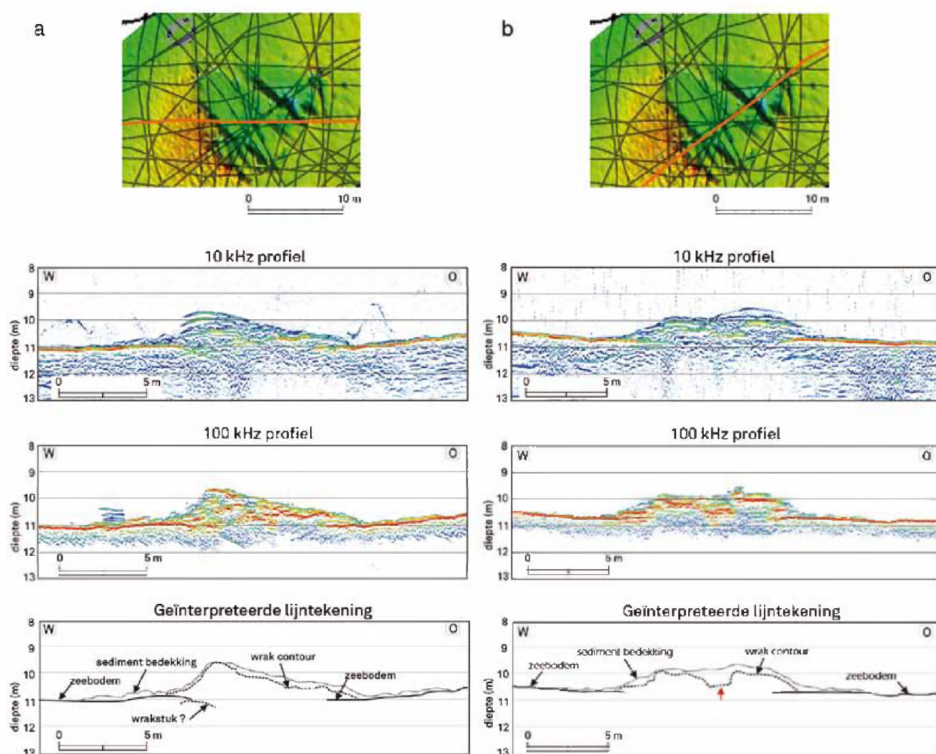
FIG. 13 a: Locatie van het profiel (in oranje aangegeven) en seismisch profiel 30 (diepte onder wateroppervlak in meter). b: Locatie van het profiel (in oranje aangegeven) en seismisch profiel 42 (diepte onder wateroppervlak in meter).
