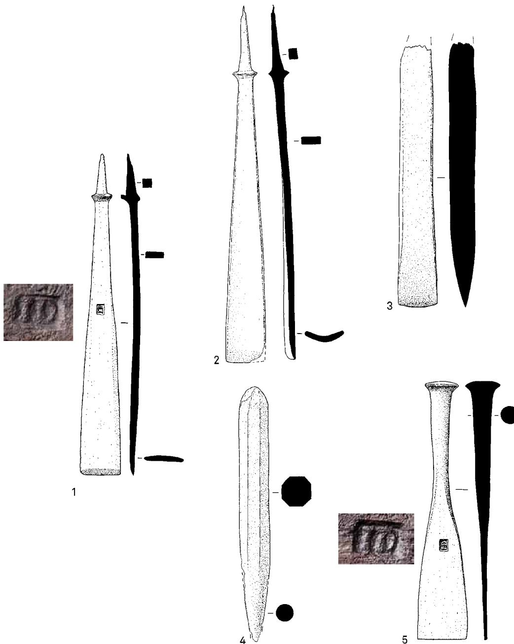
FIG. 60 1: hakbeitel, 2: schrijnwerkersguts, 3: koubeitel, 4: doorslag, 5: breeuwbeitel. Schaal 1:3. 1: mortise chisel, 2: carpenter's gouge, 3: cold chisel, 4: pointed chisel, 5: caulking iron. Scale 1:3.
