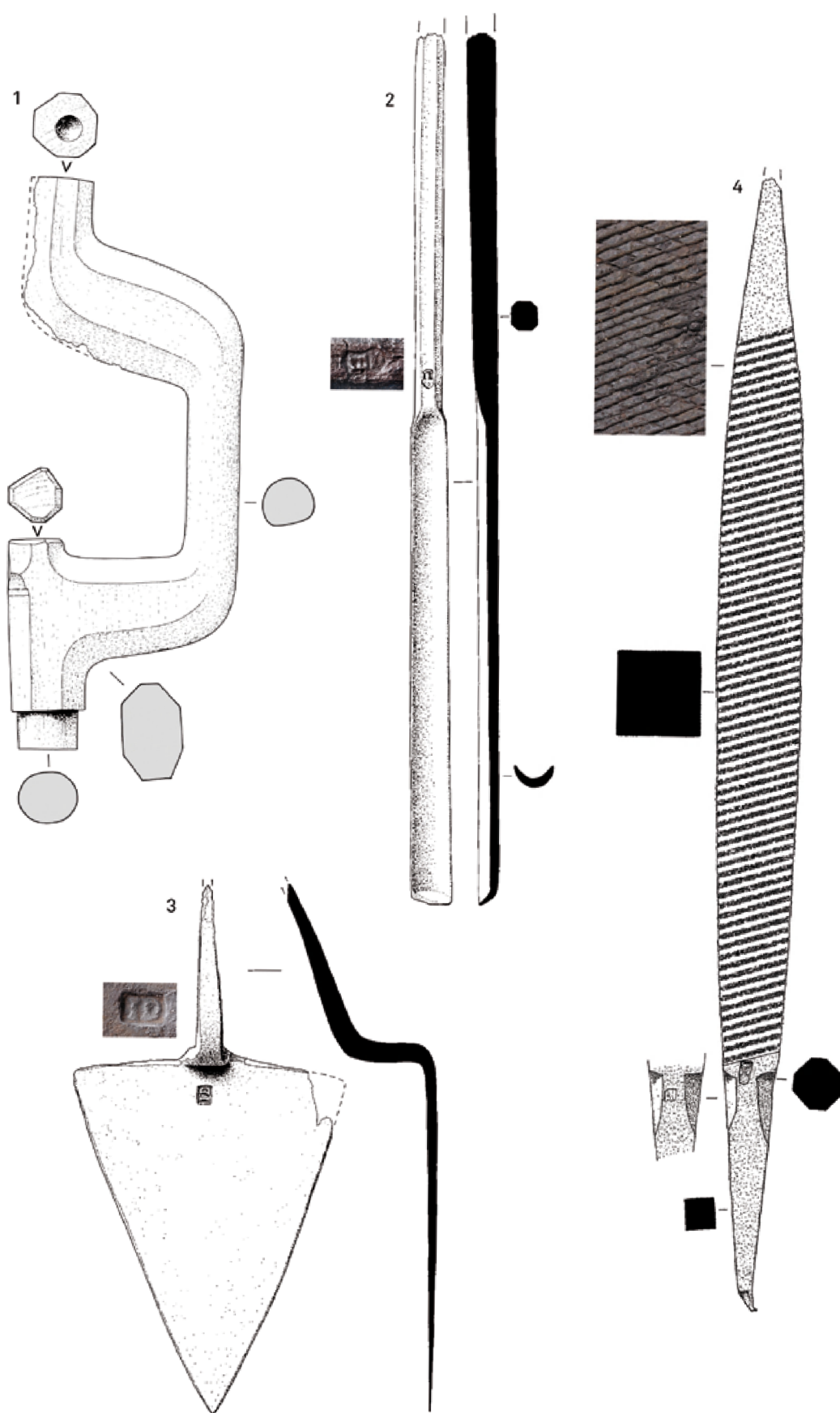
FIG. 63 1: booromslag, 2: boorijzer, 3: troffel, 4: vijl. Schaal 1:3. 1: brace, 2: bit, 3: trowel, 4: file. Scale 1:3.
