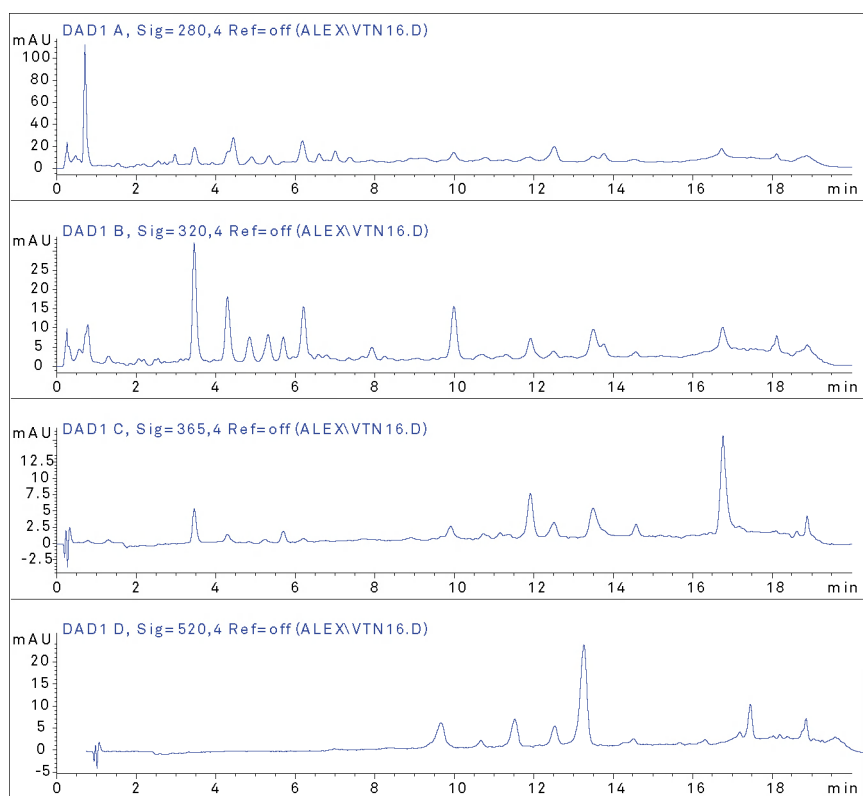
FIG. 83 Cromatograma del vino tinto DO Penedès. Compuestos y sus correspondientes picos. Ácido gálico (1), ácido protocateico (2), tirosol (3), catequina (4), epicatequina (5), t -ácido caftarico (6), t -ácido cafeico (7), t -ácido cutárico (8), ácido 2-S-glutathionil caftarico (9), quercetin-3-glucurónido (10), isoamnetina (11), quercetina (12), delphinidin-3-glucósido (13), petunidin-3-glucósido (14), peonidin-3-glucósido (15), malvidin-3-glucósido (16), malvidin-(6-acetil)-3-glucósido (17), malvidin-(6-cumaril)-3-glucósido (18).
