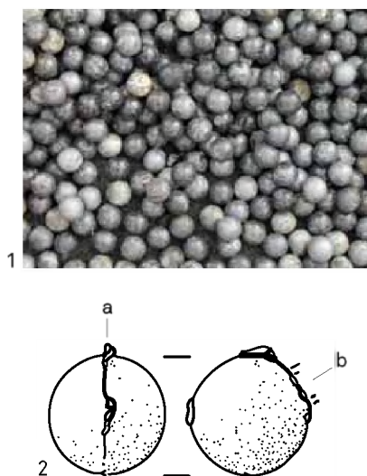
FIG. 41 1: Loden kogels van de Buiten Ratel-wraksite en 2: geweer-kogel met gietnaad (a) en afgeslepen gietprop (b). Schaal 1:1. 1: Lead bullets from the Buiten Ratel site and 2: bullet with casting seam (a) and trimmed sprue (b). Scale 1:1.
