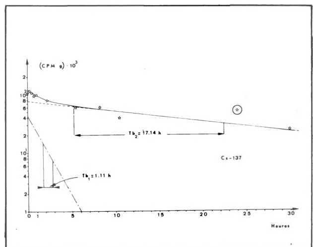
Figure 27 : Cinétique de désorption du ^{137}\text{Cs} chez Scenedesmus acutus , à partir d'une radiocontamination en culture en continu.
