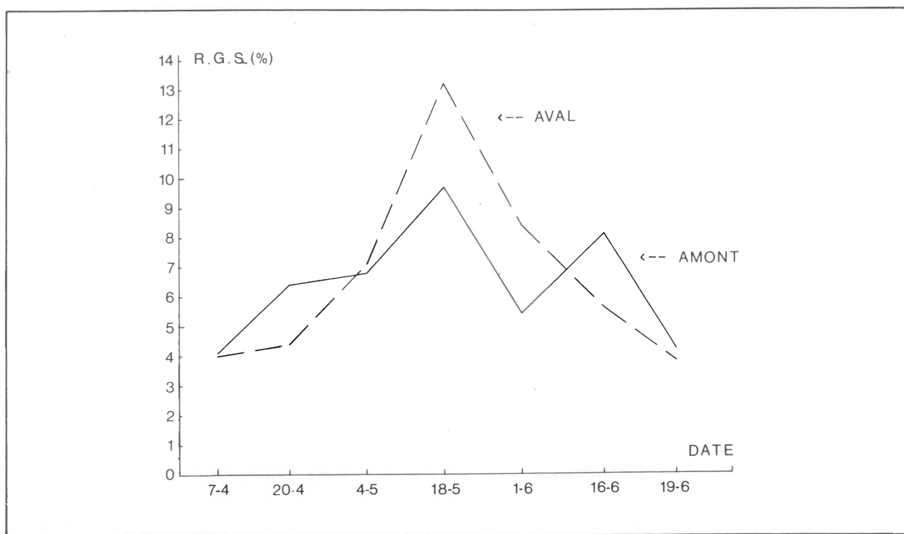
Figure 17 : Evolution des rapports gonado-somatiques moyens (R.G.S.) chez les ablettes femelles de la Meuse, en amont et en aval de la centrale de Tihange, durant le premier semestre de 1982.
