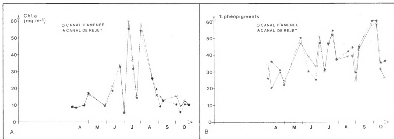
Figure 9 : A. Evolution de la biomasse du phytoplancton, estimée par la concentration en chlorophylle a, dans les canaux d'amenée et de rejet de la centrale de Tihange 1, au cours de l'année 1983.
