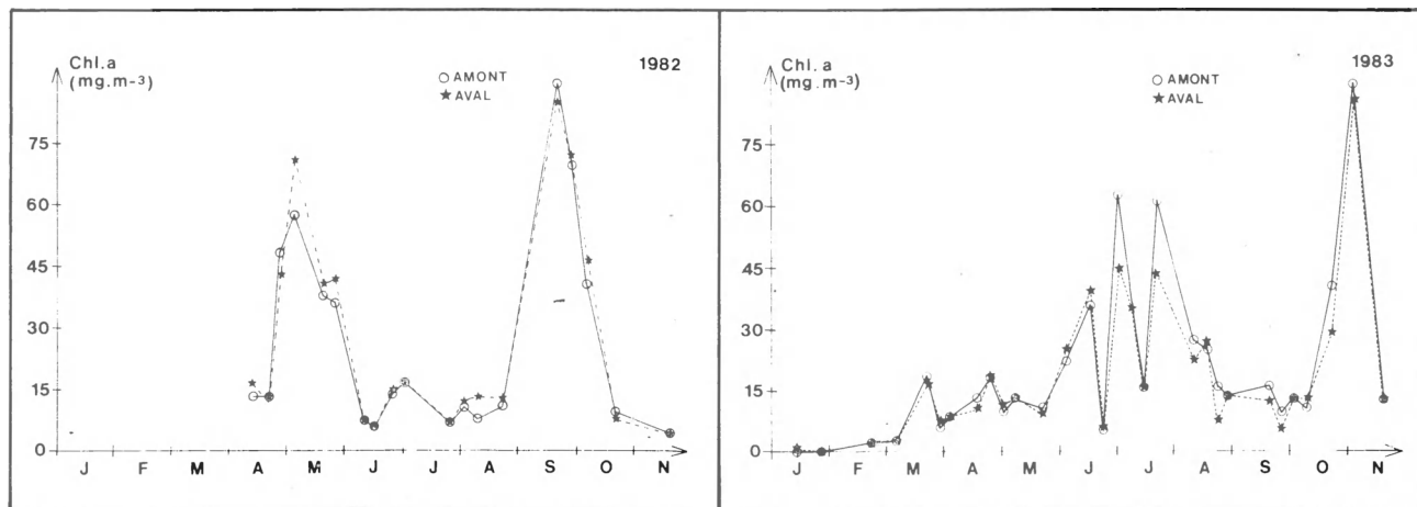
Figure 7 : Evolution de la biomasse du phytoplancton de la Meuse, estimée par la concentration en chlorophylle a , en amont et en aval de la centrale de Tihange, au cours des années 1982 et 1983.
