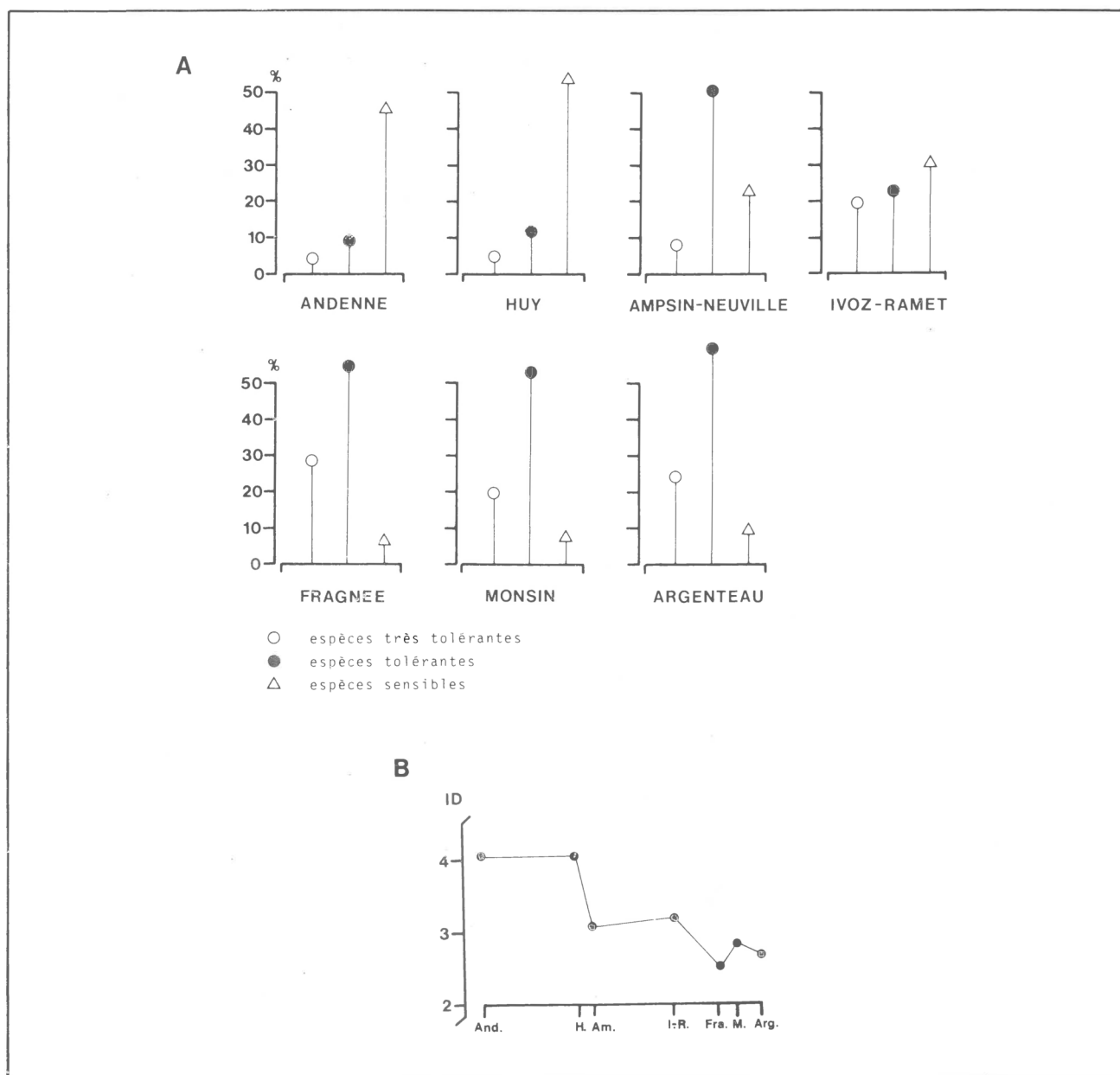
Figure 12 : A. Evolution de la structure des peuplements de diatomées du microphytobenthos dans la Meuse d'Andenne à Argenteau, en septembre 1983, d'après le système de Lange-Bertalot (1979). B. Evolution de l'indice diatomique (Descy, 1979) dans la Meuse, en septembre 1983. And. : Andenne; H. : Huy; Am. : Ampsin; I.-R. : Ivoz-Ramet; Fra. : Fragnée; M. : Monsin; Arg. : Argenteau.
