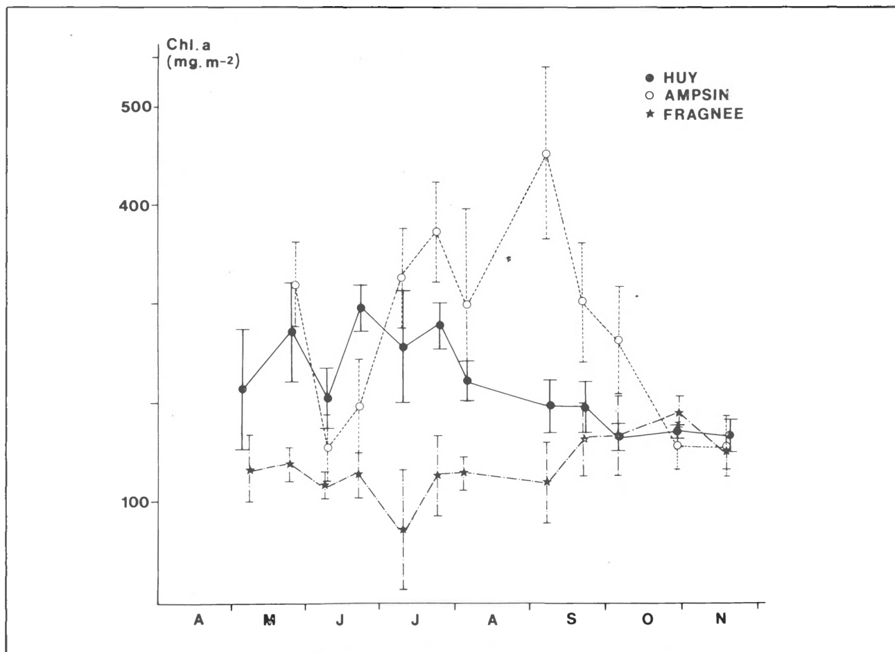
Figure 11 : Evolution de la biomasse du microphytobenthos dans les secteurs situés en amont (Huy) et en aval (Ampsint et Fragnée) de la centrale de Tihange, au cours de l'année 1981 (d'après Descy & Mouvet, 1984).
