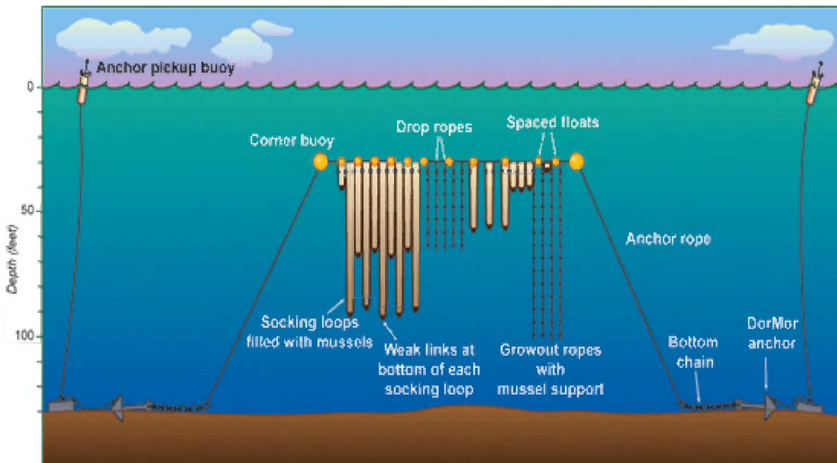
Fig. 10-33 - Het Amerikaanse ondergedompelde langlijnsysteem (SCOMAS).
