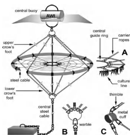
Fig. 10-38 - Overzicht zeewierkweekstelsel voor de Noordzee (Buck & Buchholz, 2004)
