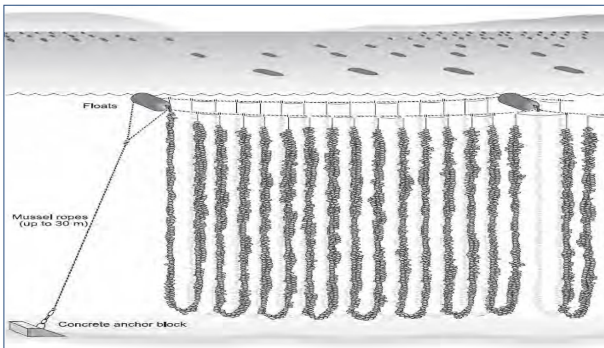
Fig. 10-32 - Het Nieuw-Zeelandse langlijnsysteem.
