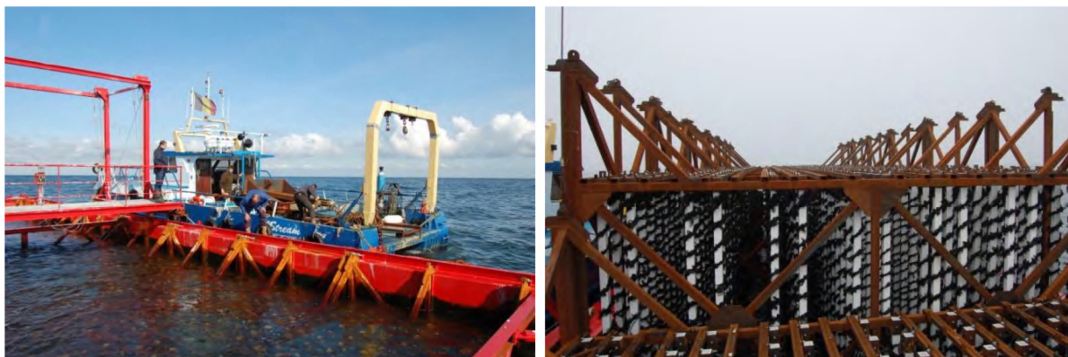
Fig. 10-24 - De mosselkooistructuur met aparte kooien in één grote vlottende kooi Belgische kooisysteem voor de offshore kweek van mosselen gebruikt door Reynaert-Versluys.
