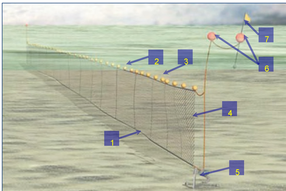
Fig. 9-7 – Staand want vistuig
