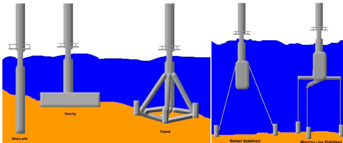
Fig. 2-1 – Verschillende types funderingen voor windmolens op zee ( http://offshorewind.net/Other_Pages/Turbine-Foundations.html )
