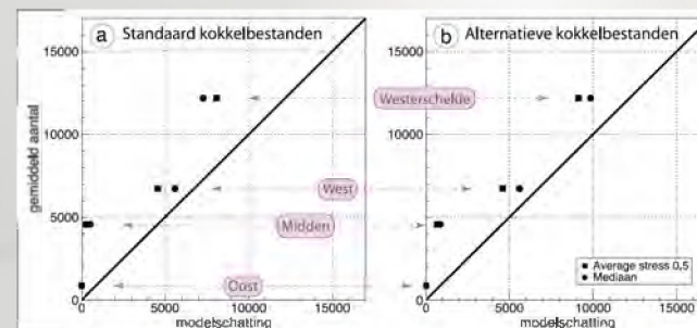
Figuur 1: WEBTICS modelschatting vergeleken met waargenomen aantallen scholeksters. A: uitgaande van standaard kokkelbestanden en b: uitgaande van kokkelbestanden gecorrigeerd voor verlies door vissen
