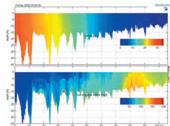
Figuur 2: Berekend zoutgehalte (ppt) en slibconcentratie (mg/L) langs de hoofdgeul van de Schelde voor hoog rivierafvoer ( 283 \text{ m}^3/\text{s} ). Vliissingen = 0 km, Antwerpen = 90 km. Het troebelingsmaximum bij Antwerpen is duidelijk zichtbaar.
