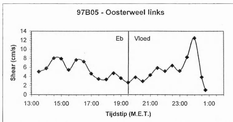
Figuur 13: wrijvingssnelheid te Oosterweel links (voorjaar 1997)
