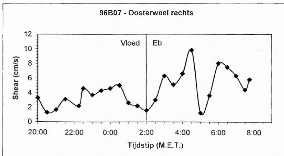
Figuur 10: de wrijvingssnelheid in Oosterweel rechts in het voorjaar van 1996.
