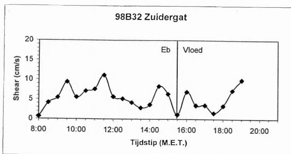
Figuur 6: wrijvingssnelheid ter hoogte van het Zuidergat
