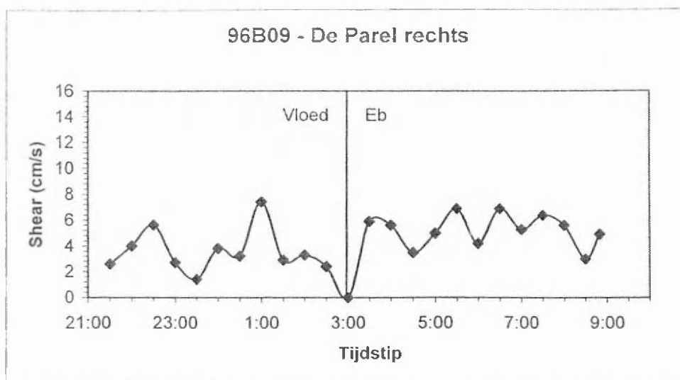
Figuur 17: overzicht wrijvingssnelheid op station De Parel rechts.
