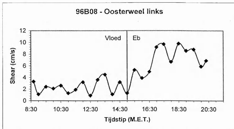
Figuur 11: de wrijvingssnelheid in Oosterweel links (voorjaar 1996).
