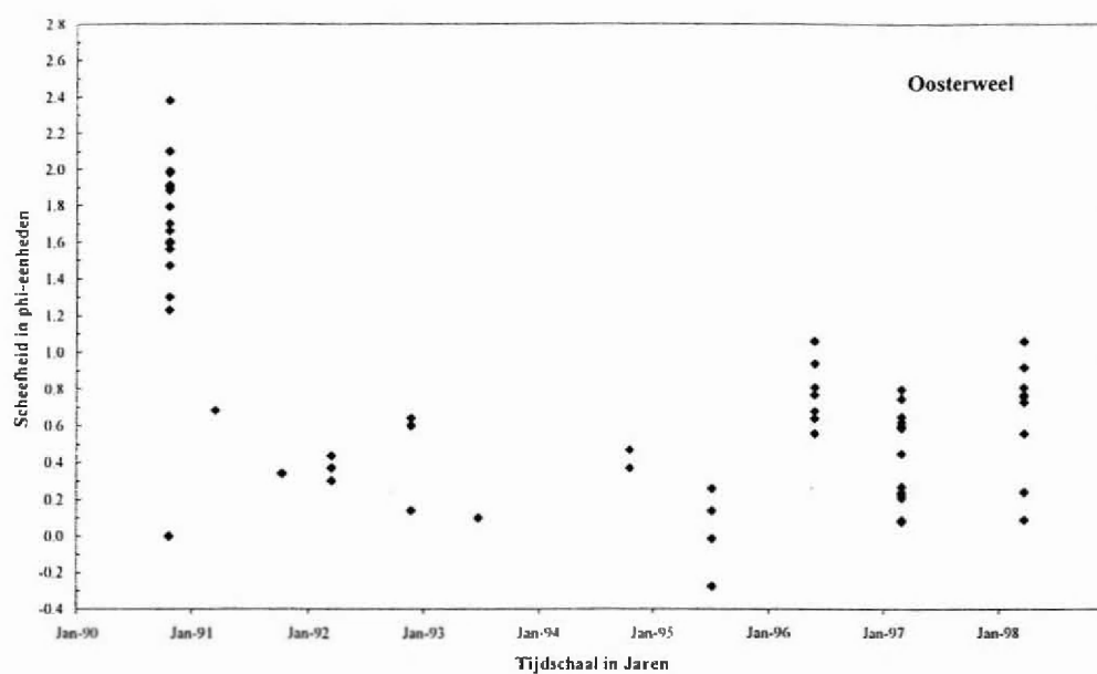
Figuur 71: scheefheid van de korrelgrootteverdeling van het suspensiesediment voor de periode 1990-1998.
