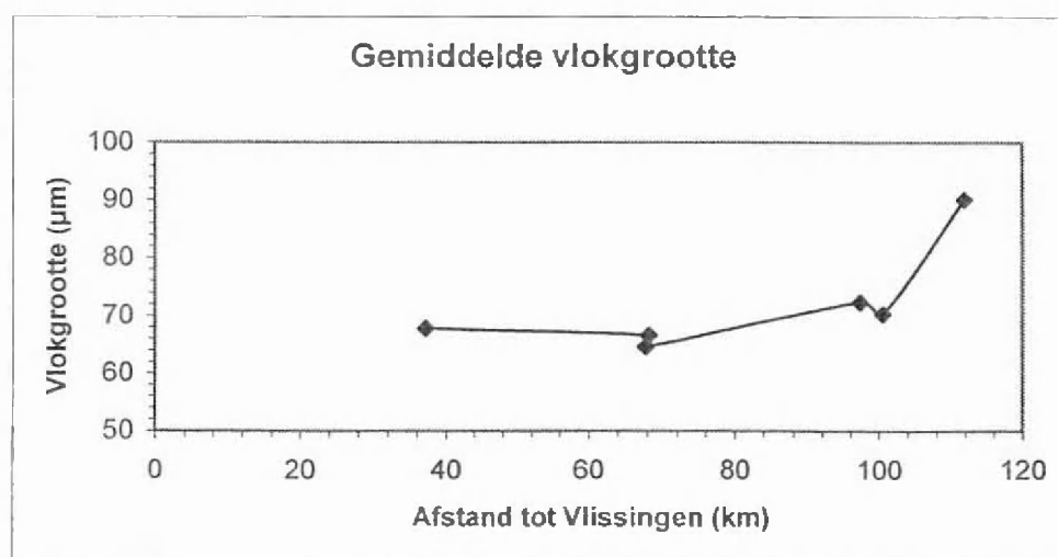
Figuur 55: de gemiddelde vlokgrootte in functie van de afstand tot Vlissingen
