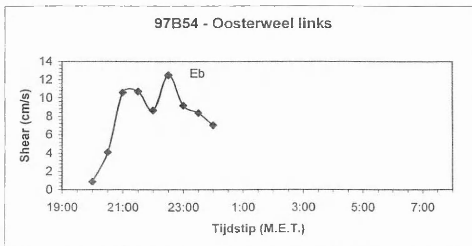
Figuur 15: wrijvingssnelheid ter hoogte van Oosterweel links (najaar 1997)
