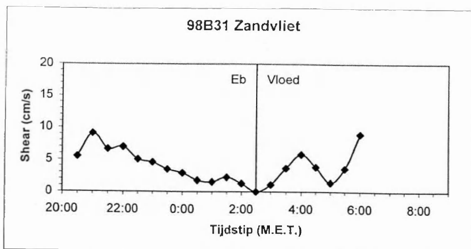
Figuur 5: variatie in de wrijvingssnelheid ter hoogte van Zandvliet
