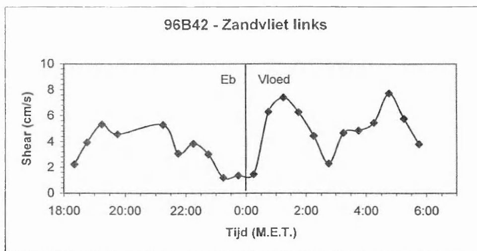
Figuur 19: verloop van de wrijvingssnelheid ter hoogte van Zandvliet links.
