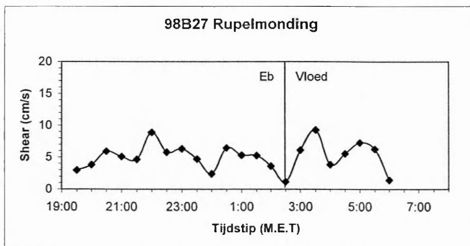
Figuur 1: variatie in de wrijvingssnelheid (shear) in de tijd ter hoogte van de Rupelmonding.
