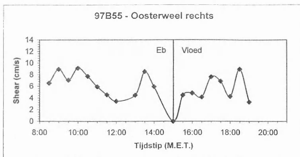
Figuur 14: wrijvingssnelheid te Oosterweel rechts (najaar 1997)
