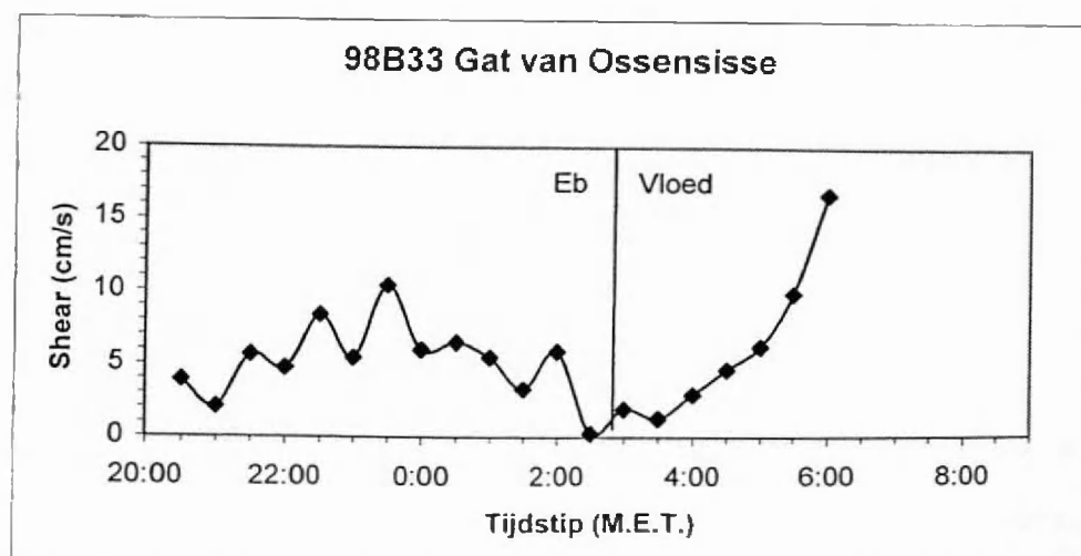
Figuur 7: variatie van de wrijvingssnelheid te Ossensisse
