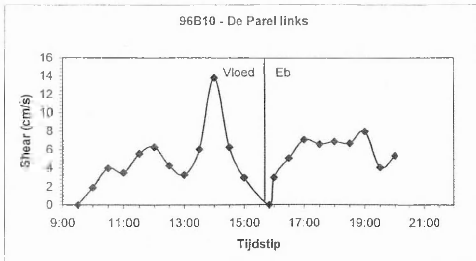
Figuur 16: de wrijvingssnelheid ter hoogte van De Parel links.
