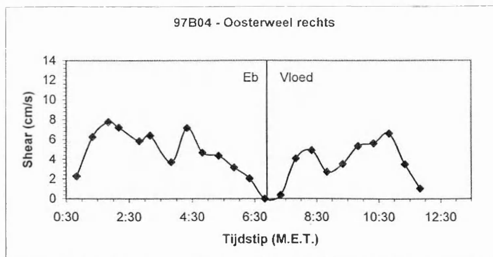
Figuur 12: wrijvingssnelheid te Oosterweel rechts (voorjaar 1997).
