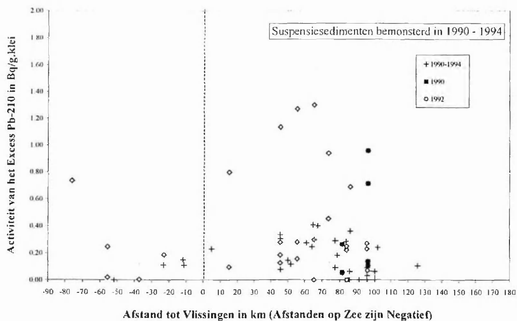
Figuur 63: exces activiteit van het ^{210}\text{Pb} in Bq/g.klei voor suspensiesedimenten uit de periode 1990-1994
