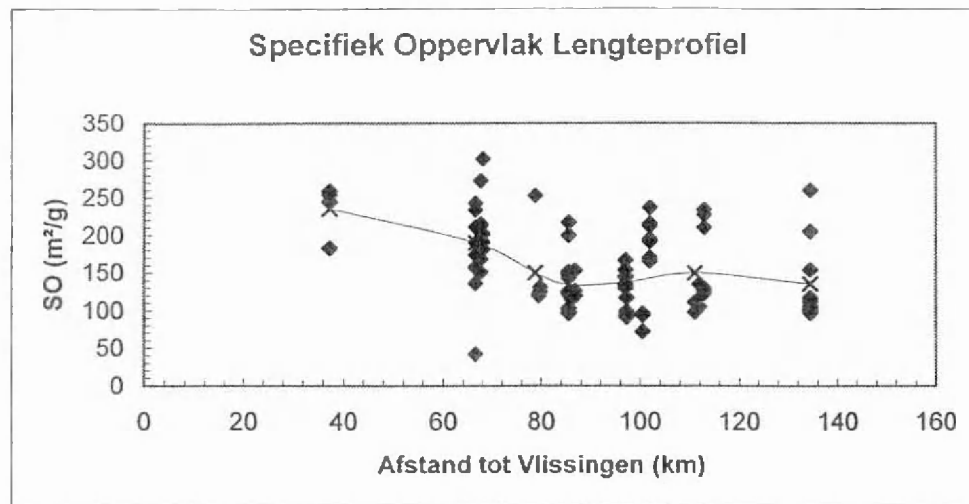
Figuur 56: variatie van het specifiek oppervlak van suspensiesedimenten over het Schelde-estuarium.
