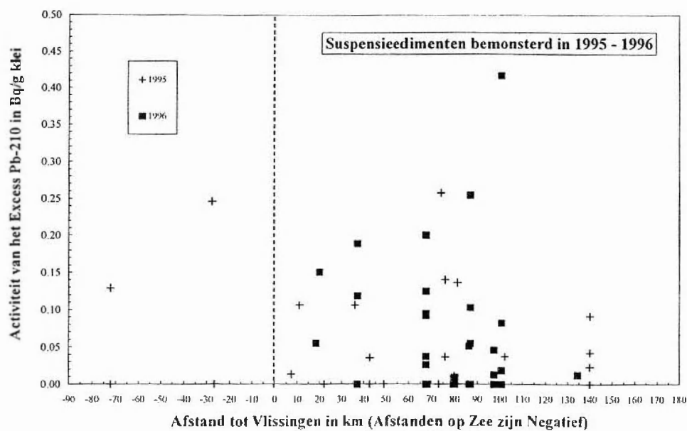
Figuur 64: exces activiteit van het ^{210}\text{Pb} in Bq/g.klei voor suspensiesedimenten uit de periode 1995-1996
