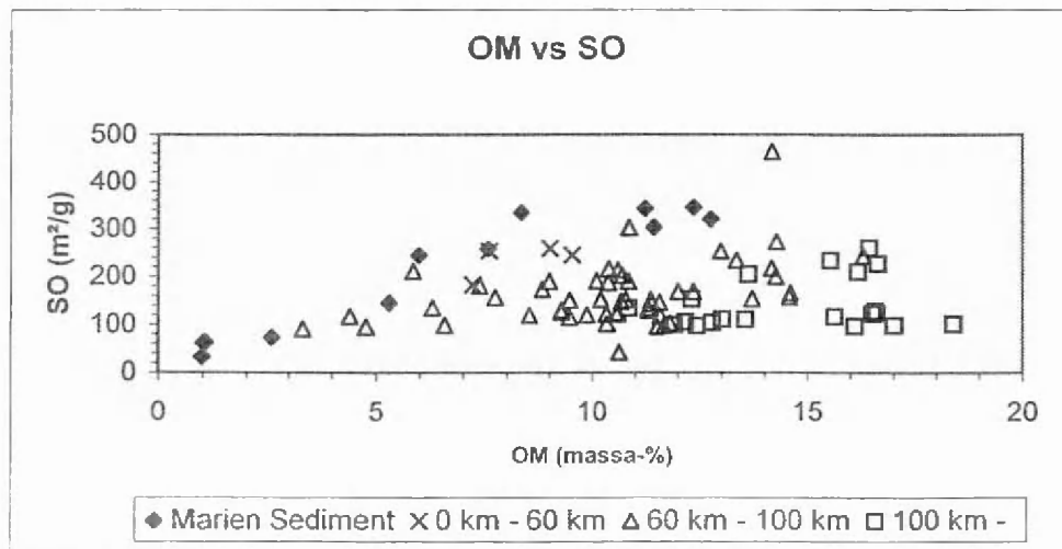
Figuur 57: relatie organisch materiaal – specifiek oppervlak voor Schelde-suspensiesedimenten.
