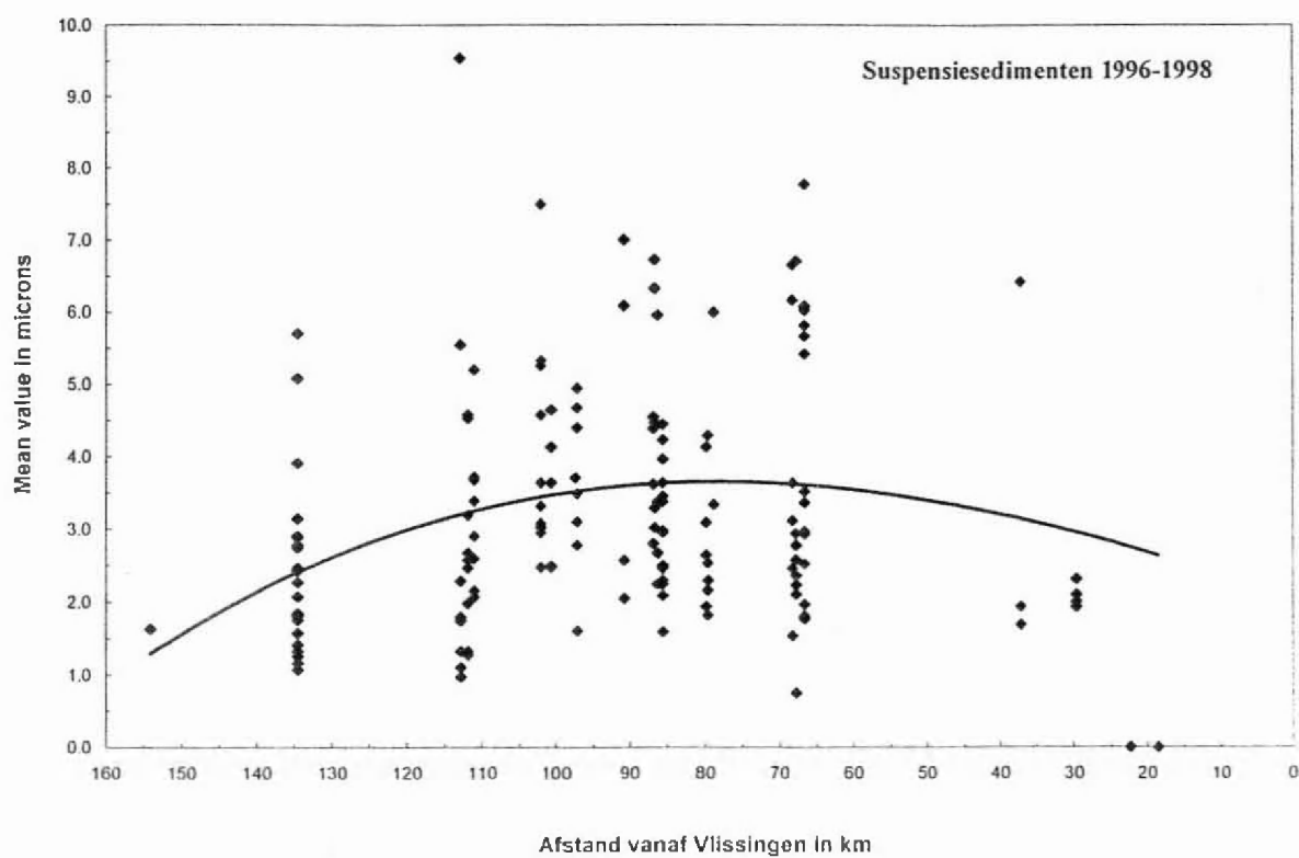
Figuur 53: gemiddelde korrelgrootte van suspensiesedimenten 1996-1998
