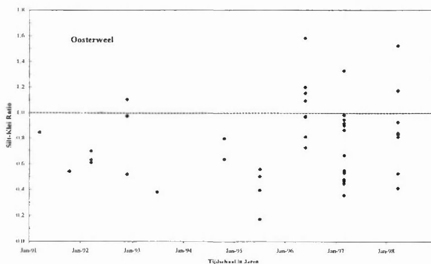
Figuur 70: silt-klei verhouding van het suspensiesediment voor de periode 1990-1998.
