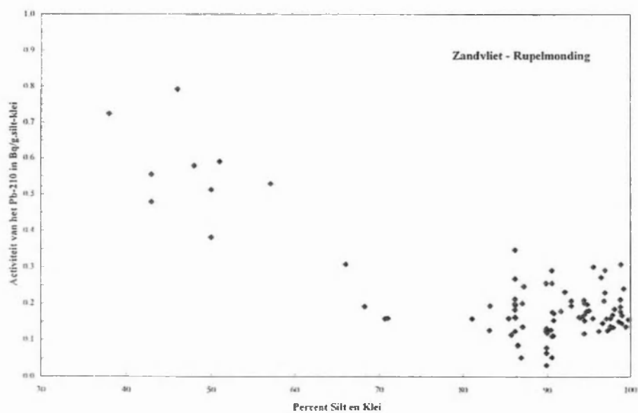
Figuur 68: activiteit van het ^{210}\text{Pb} in Bq/g.silt-klei ten opzichte van percentage silt-klei in het supsiesediment.
