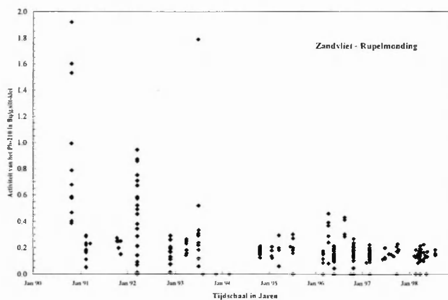
Figuur 66: activiteit van het ^{210}\text{Pb} in Bq/g.silt-klei voor sedimenten bemonsterd in de periode 1990-1998.
