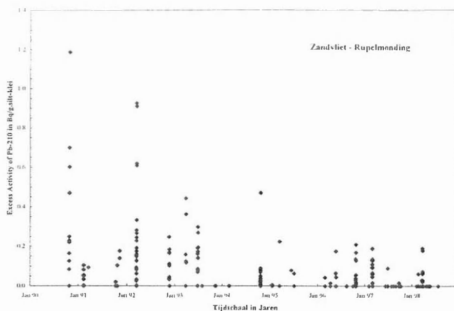
Figuur 67: exces-activiteit van het ^{210}\text{Pb} in Bq/g.silt-klei voor sedimenten bemonsterd in de periode 1990-1998.
