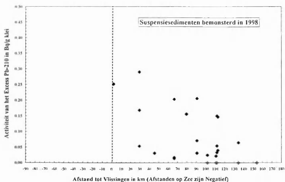
Figuur 65: exces activiteit van het ^{210}\text{Pb} in Bq/g.klei voor suspensiesedimenten uit de periode 1998
