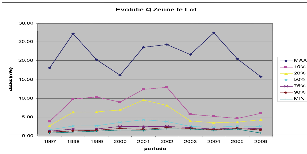
Figuur 35: Waterkwantiteitsmetingen op Zenne te Lot
