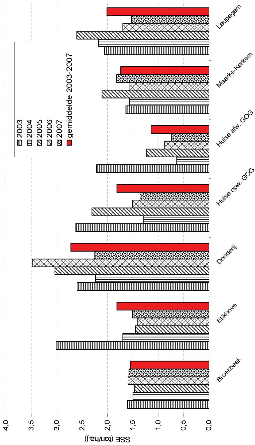
Figuur 47: Onbevaarbare sedimentmeetnet Bovenschelde: overzicht van de SSE-waarden over de periode 2003 - 2007; afgebeeld van links naar rechts volgens stroomgebiedsgrootte (223 ha - 4947 ha)
