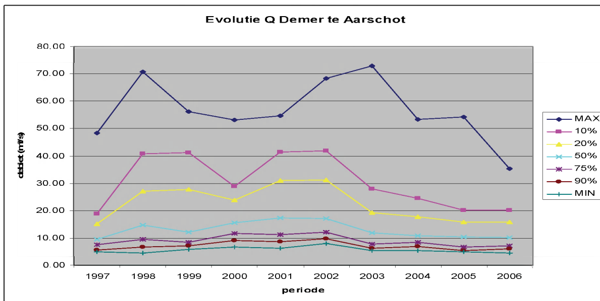
Figuur 34: Waterkwantiteitsmetingen op Demer te Aarschot
