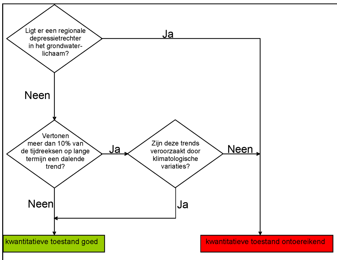
Figuur 43: Schema voor de test waterbalans voor de kwantitatieve beoordeling
