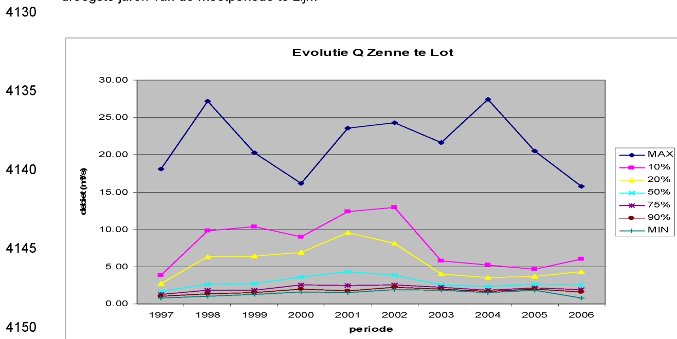
Figuur 34: Waterkwantiteitsmetingen op Zenne te Lot
