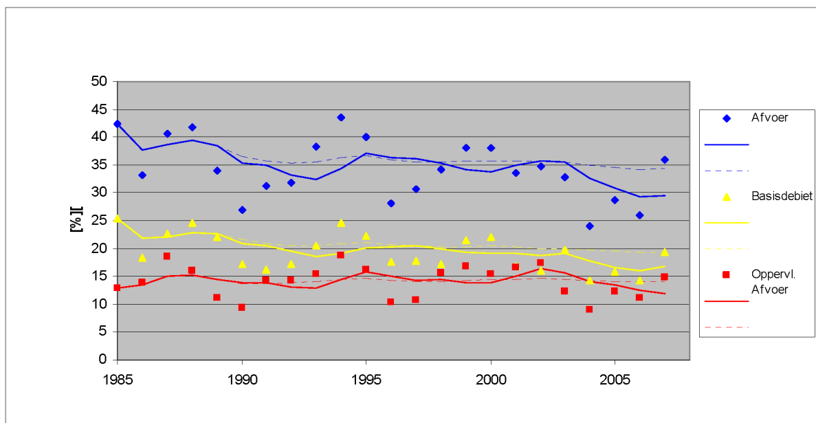
Figuur 40: De gemiddelde afvoer uitgedrukt als percentage van de gemiddelde gebiedsneerslag [%] van 5 meetlocaties. Volle lijn: 5-jaargemiddelde; stippellijn: voortschrijdend gemiddelde.
