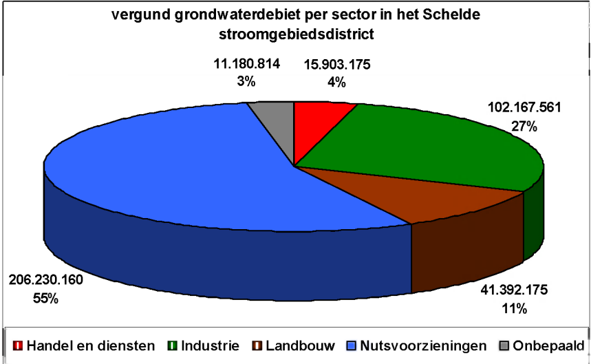
1690 Figuur 25: Vergunde hoeveelheid grondwater en percentages per sector in het SGD Schelde
