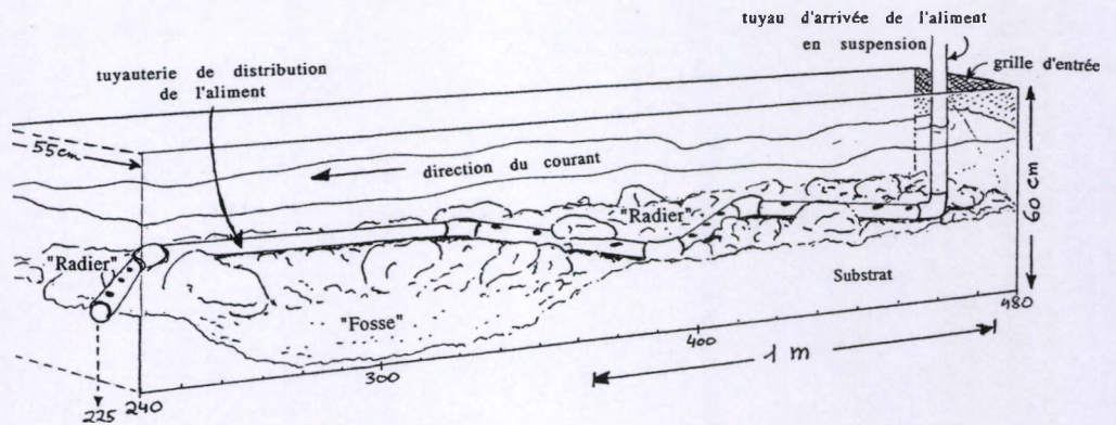
Figure 6.7 : Dessin schématique de la partie amont de la rivière artificielle. La tuyauterie d'alimentation, composée d'une série articulée de 5 tuyaux en PVC, est légèrement enfoncée dans le substrat.
