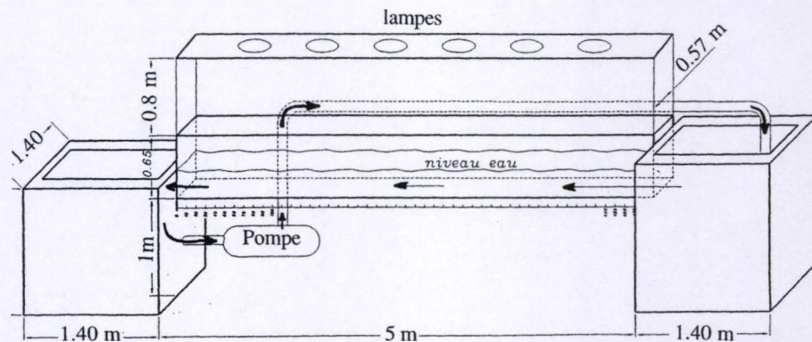
Figure 6.1 : Schéma général de la rivière artificielle.
