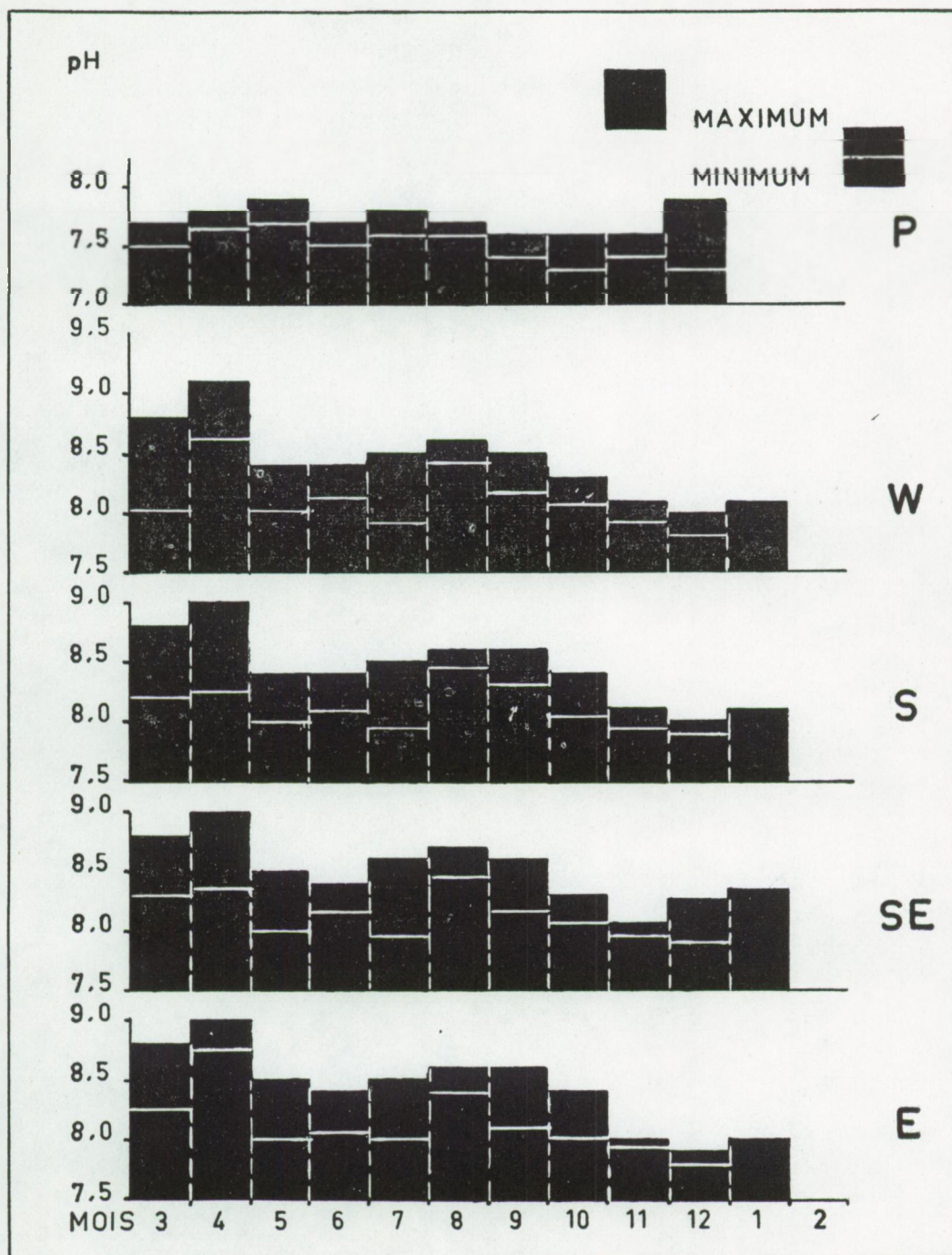
Fig. 20. Maximale en minimale waargenomen waarden van de pH in de haven van Oostende en in vier verschillende biotopen in de Spuikom gedurende het jaar 1960.
