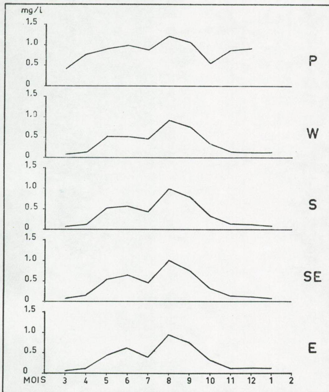
Fig. 28. Fosphaatgehalte van het water in de haven van Oostende en in vier onderzochte biotopen in de Spuikom, uitgedrukt in mg/l.
