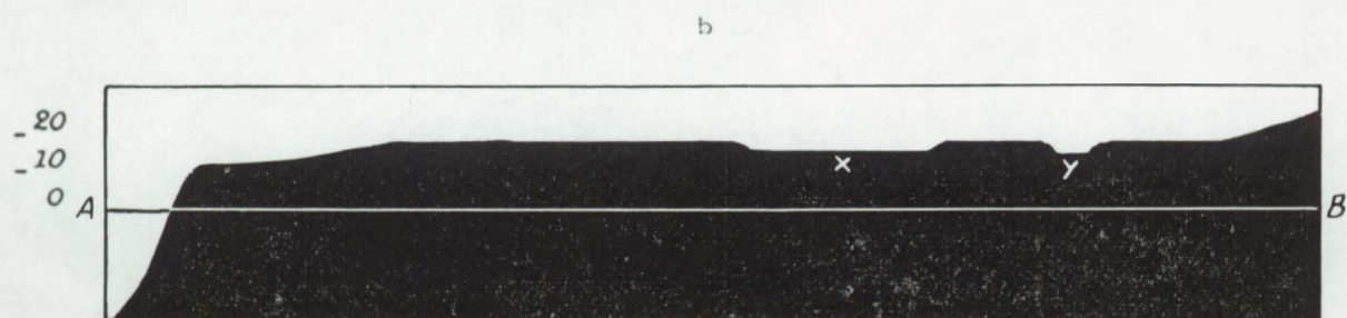
II'' Fig. 5. Verloop der diepte in de Spuikom volgens de lijn AB (Fig. 3) in 1959.
