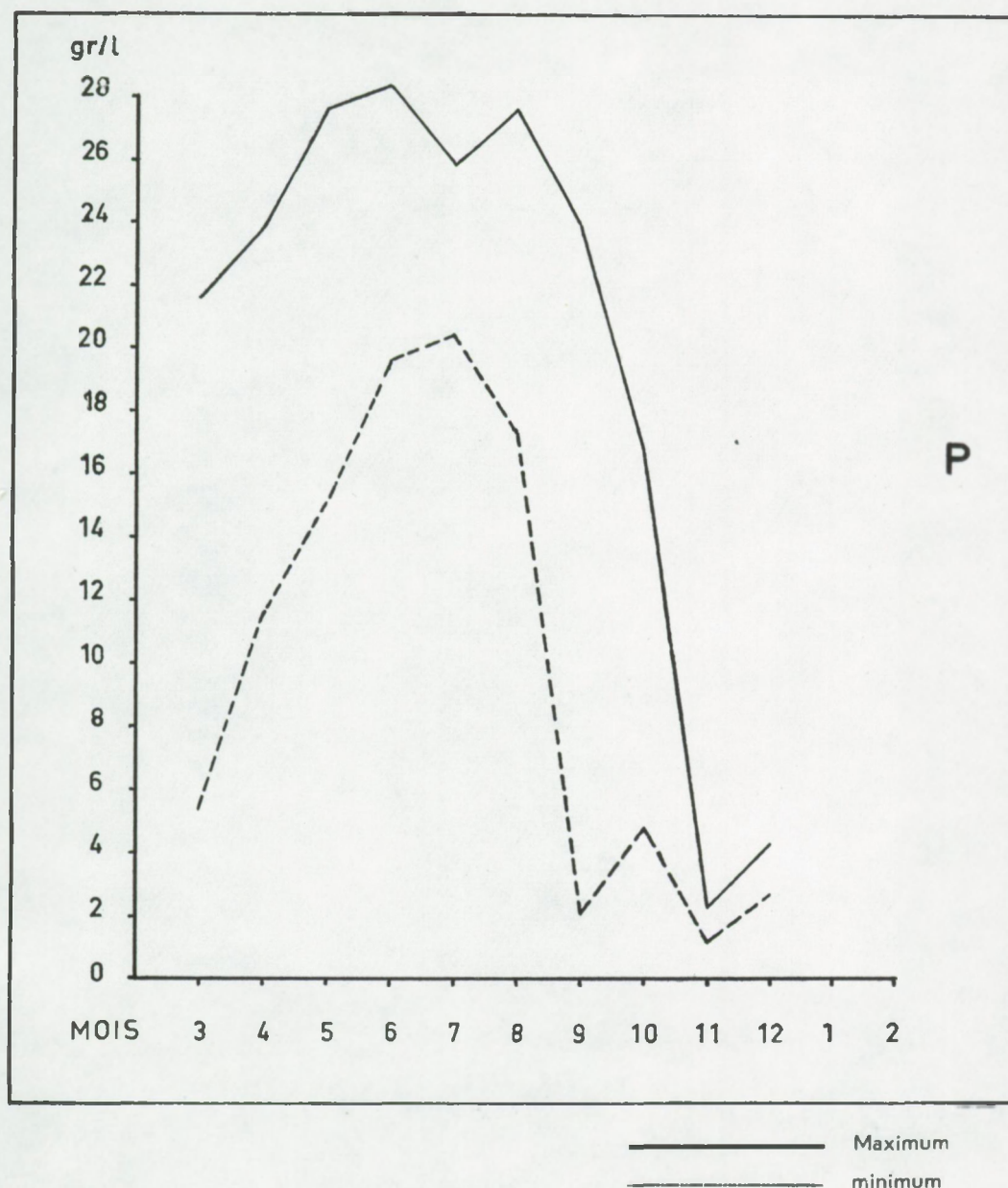
Fig. 17. Maximale en minimale waargenomen waarden van het zoutgehalte in de haven van Oostende.
