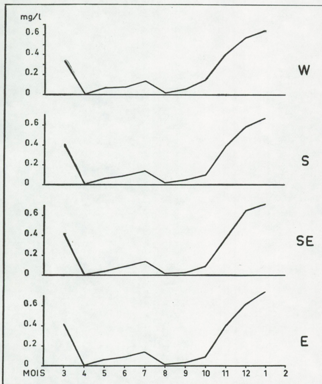
Fig. 27. Nitrietgehalte van vier onderzochte biotopen in de Spuikom te Oostende, uitgedrukt in mg/l.
