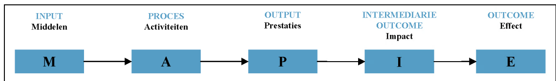
Figuur 4: MAPIE-keten
