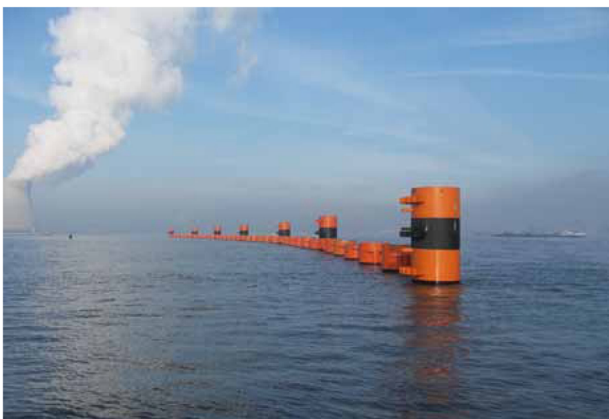
Het ontwerp van de Current Deflecting Wall werd uitgedokterd door experts
