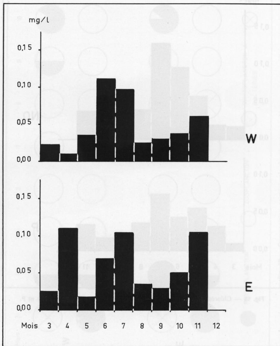
Fig. 15 — Chlorophylle en mg/litre — Moyennes mensuelles, points W et E.
