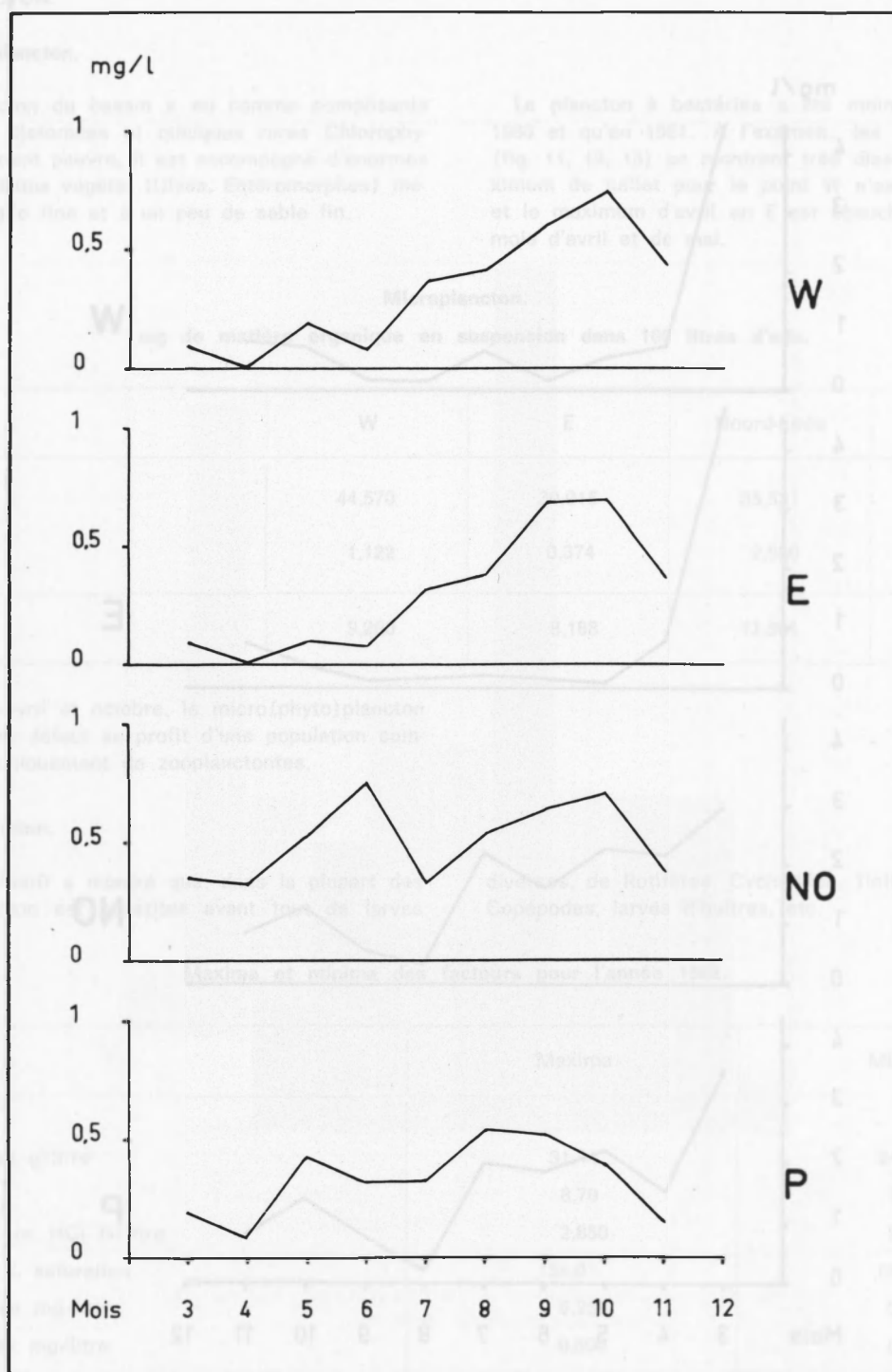
Fig. 9 — Phosphates PO 4 mg/litre — Moyennes mensuelles.
