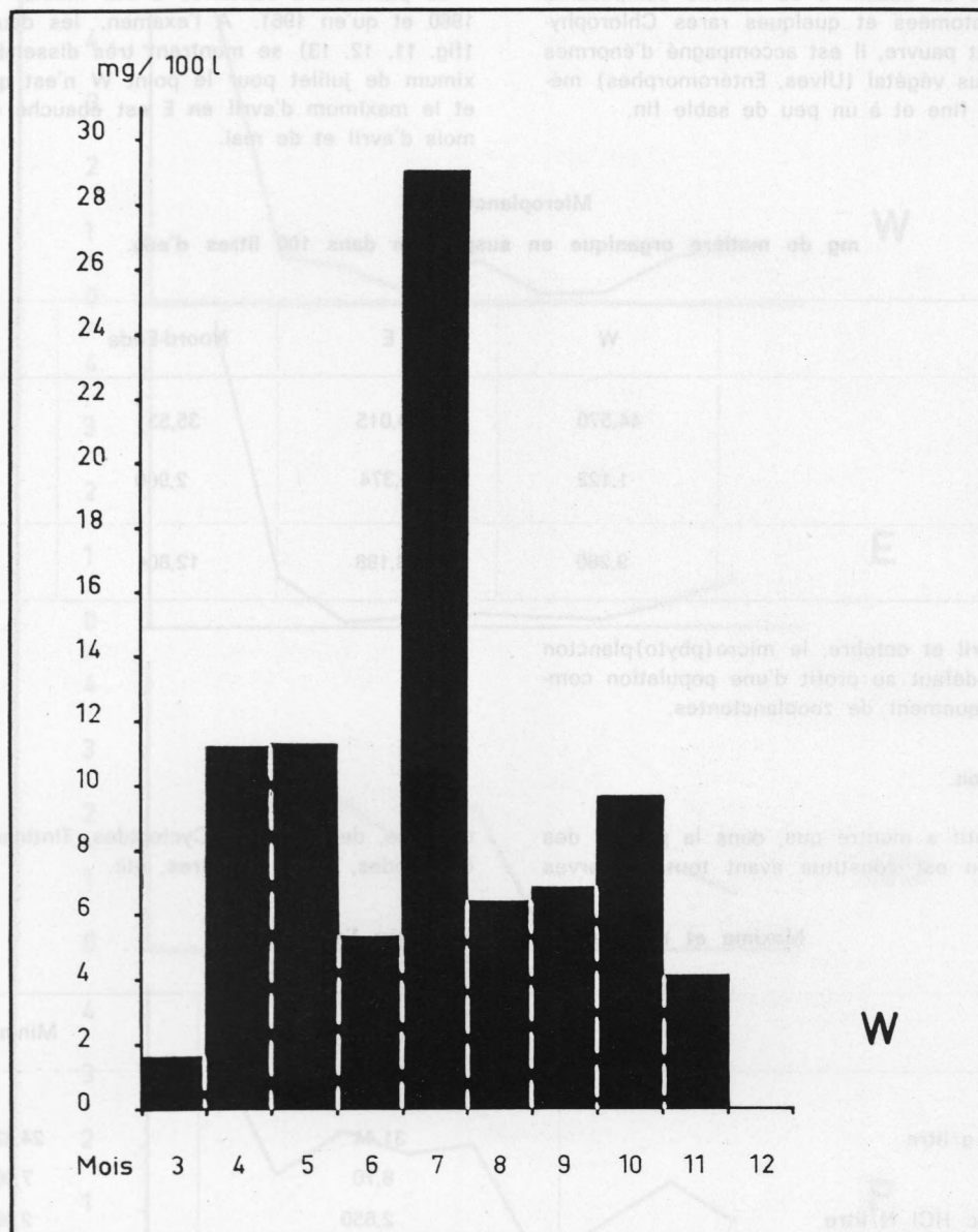
Fig. 11 — Microplankton — Matières organiques en mg 100 l : Moyennes mensuelles, point W.
