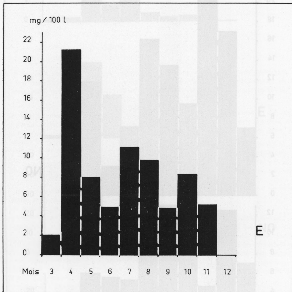
Fig. 12 — Microplancton — Matières organiques en mg/100 l : Moyennes mensuelles, point E.
