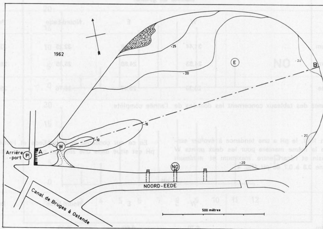
Fig. 1 — Topographie du bassin de chasse d'Ostende, 1962.
