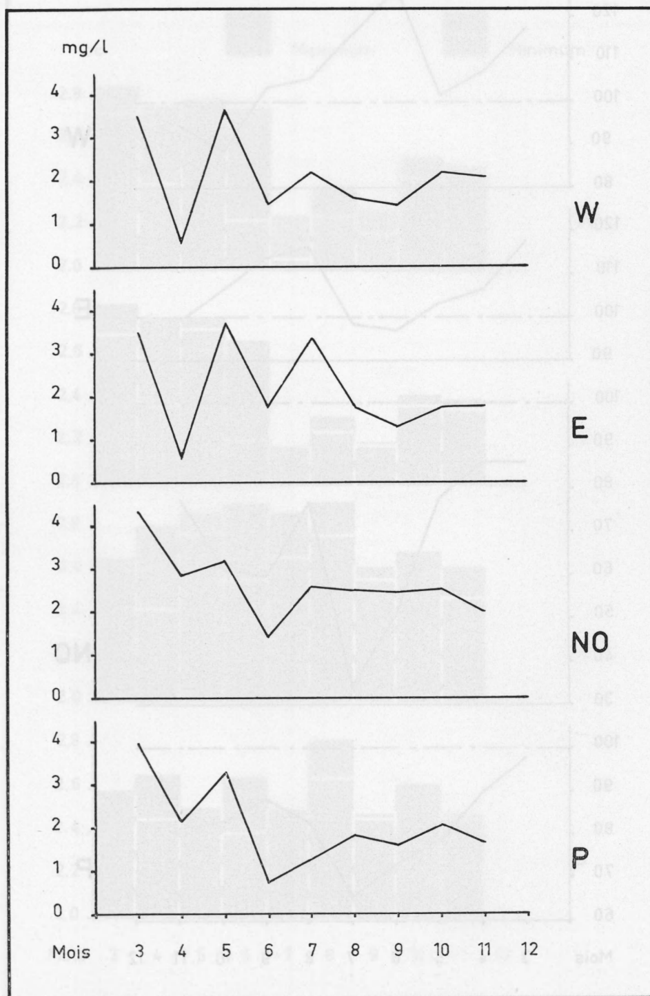
Fig. 7 — Nitrates NO 3 mg/litre — Moyennes mensuelles.
