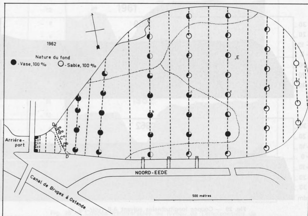
Fig. 30 — Répartition de la vase et du sable dans le bassin de chasse d'Ostende, 1962.
