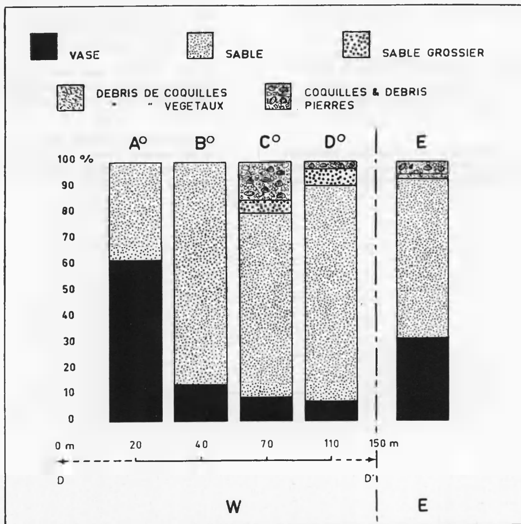
Fig. 32 — % des éléments des échantillons de fond prélevés en août 1961 : A°-D°, le long de l'emplacement de l'ancienne digue D-D' et E, à l'Est du bassin (voir fig. 28, 30).
