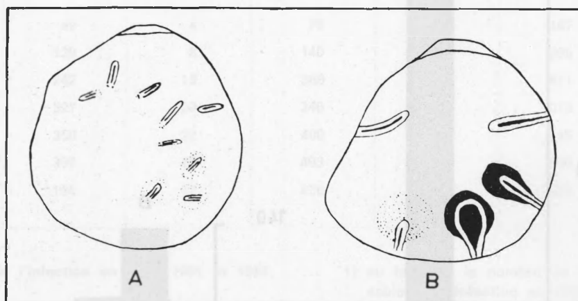
Fig. 25 — Vues intérieures de valves présentant les résultats de la présence de (A) Polydora ciliata (JOHNSTON) et de (B) Polydora hoplura CLAPAREDE. En noir : tubes, poches et dépôts vaseux provoqués par les vers ; en pointillé : zones de conchyoline sécrétée par l'huître. (d'après P. KORRINGA, 1951).
