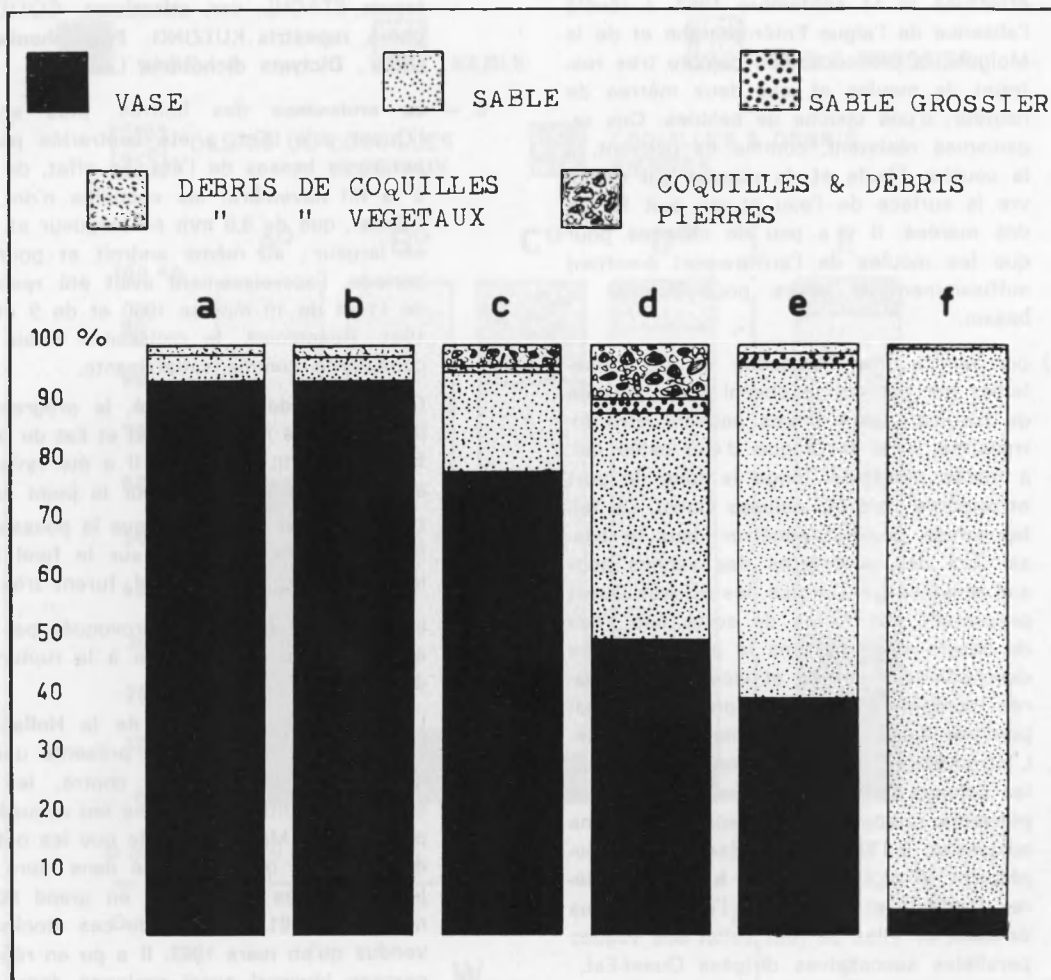
Fig. 31 — % des éléments des échantillons de fond prélevés en 1962 le long d'une ligne longitudinale a-f (voir fig. 1).
