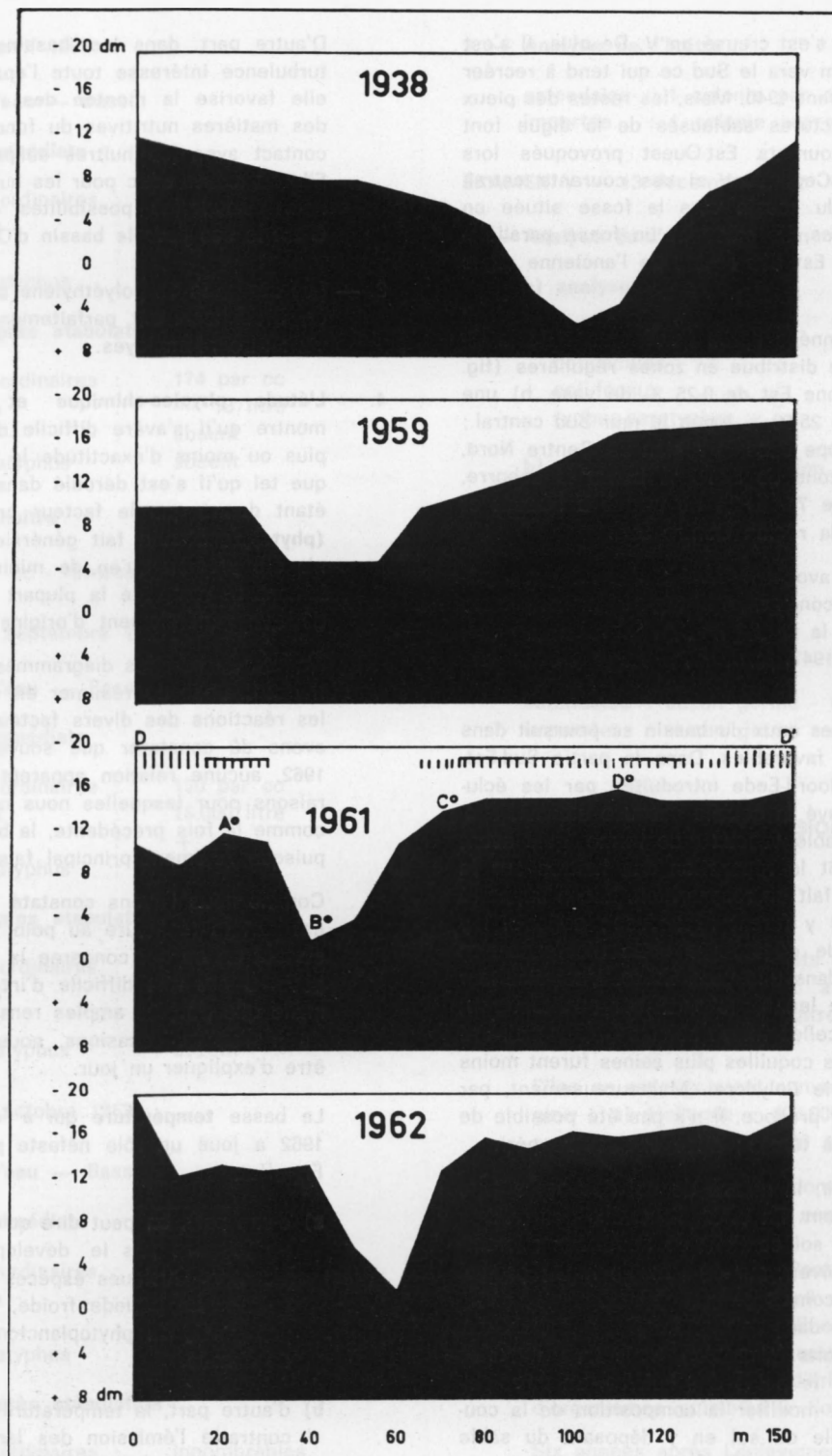
Fig. 28 — Coupes transversales au niveau de l'emplacement de l'ancienne digue, D-D' (voir fig. 30).
