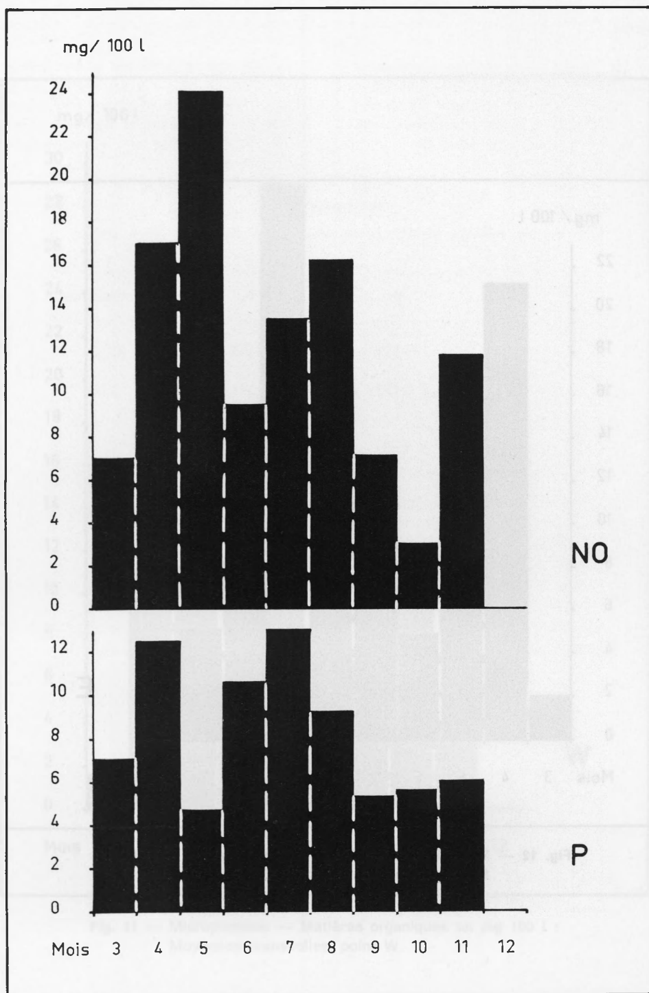
Fig. 13 — Microplancton — Matières organiques en mg/100 l : Moyennes mensuelles, points NO et P.
