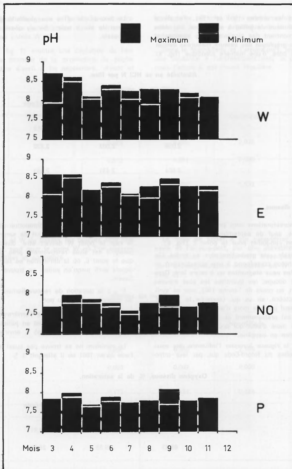
Fig. 4 — pH : Moyennes mensuelles — Maximum — minimum.
