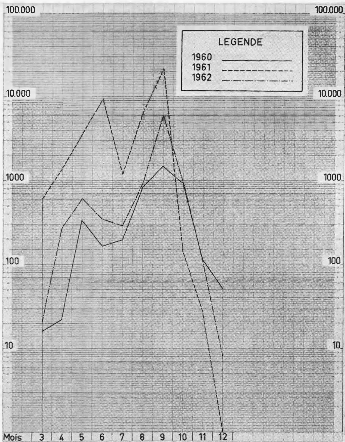
Fig. 23 — Nombre moyen de larves de Polydora par mois et pour 50 l d'eau en 1960, 1961 et 1962.
