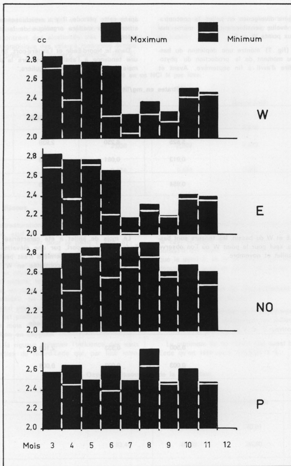
Fig. 5 — Alcalinité cc HCl N/litre : Moyennes mensuelles — Maximum — minimum.
