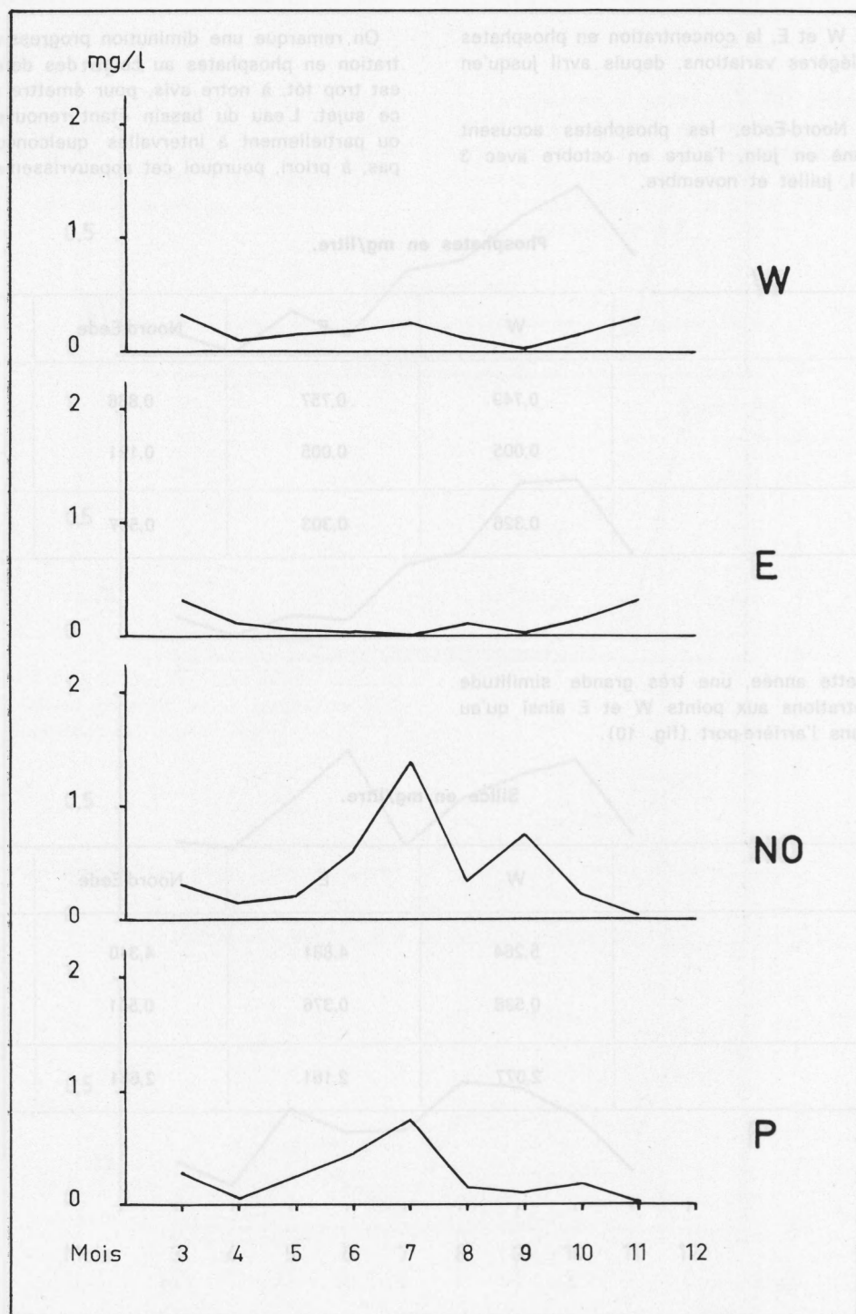
Fig. 8 — Nitrites NO 2 mg/litre — Moyennes mensuelles.
