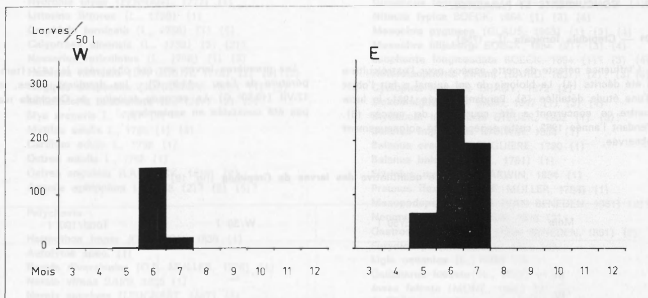
Fig. 19 — Nombre de larves de Crepidula fornicata L. par mois et pour 50 l d'eau, dans les biotopes W et E.
