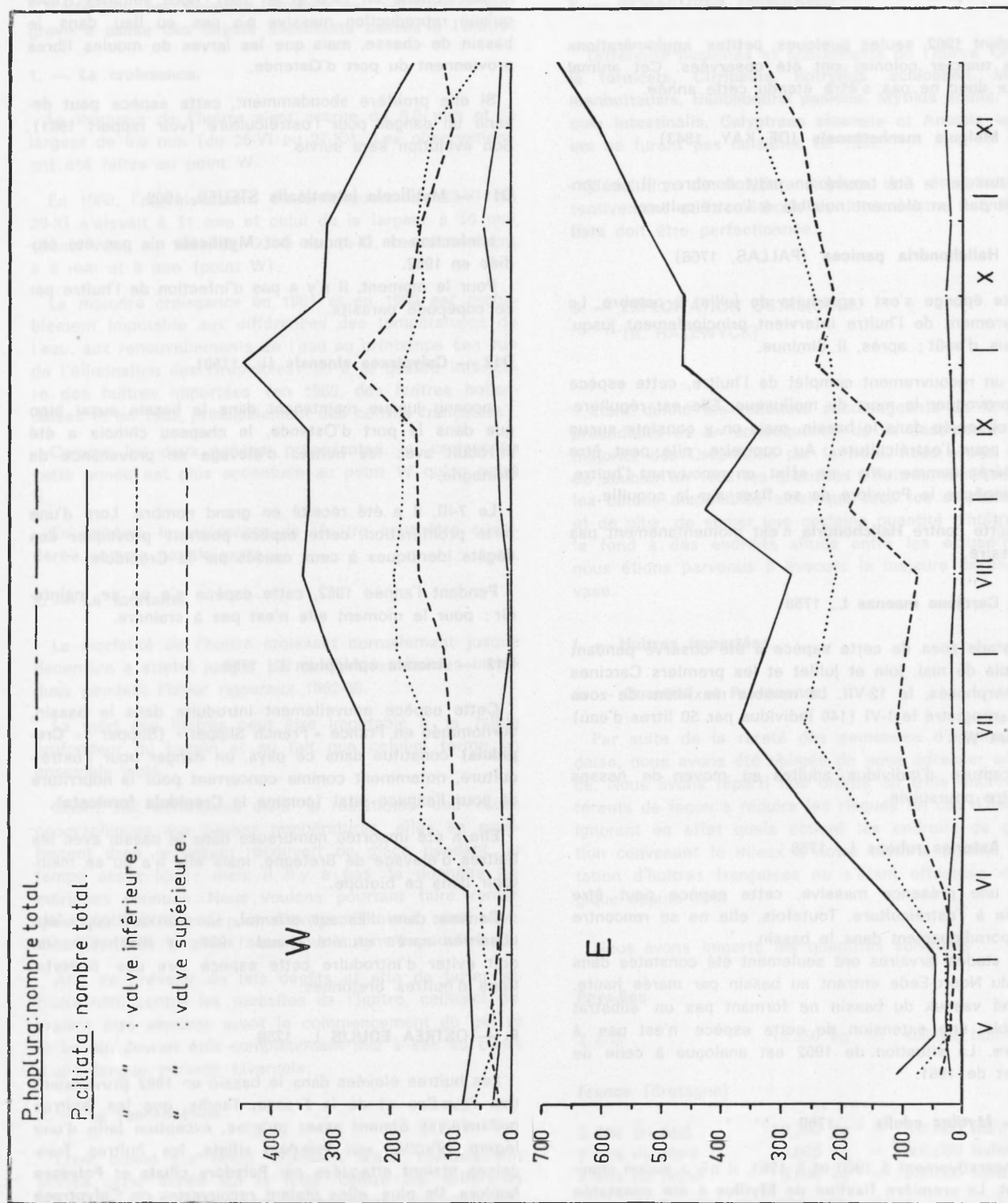
Fig. 27 — Nombre de galeries creusées par Polydora ciliata (JOHNSTON) et Polydora hoplura CLAPAREDE par 16 huitres dans les biotopes W et E.
