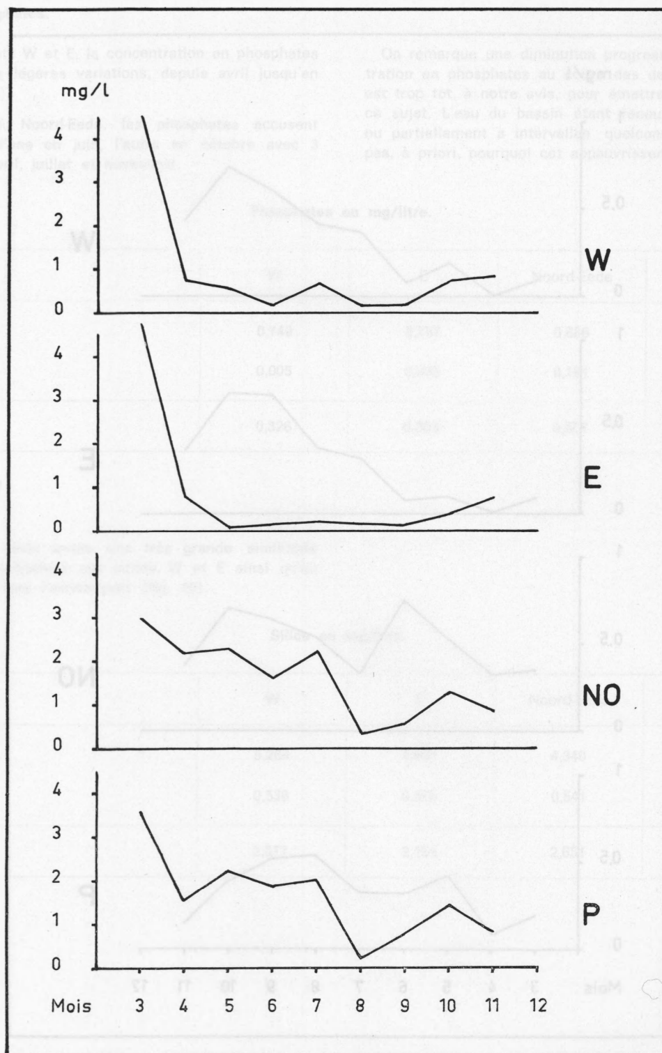
Fig. 10 — Silice \text{SiO}_2 mg/litre — Moyennes mensuelles.
