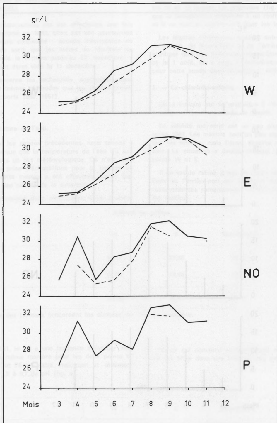
Fig. 3 — Salinité : Moyennes mensuelles ——— = Maximum - - - - = minimum.
