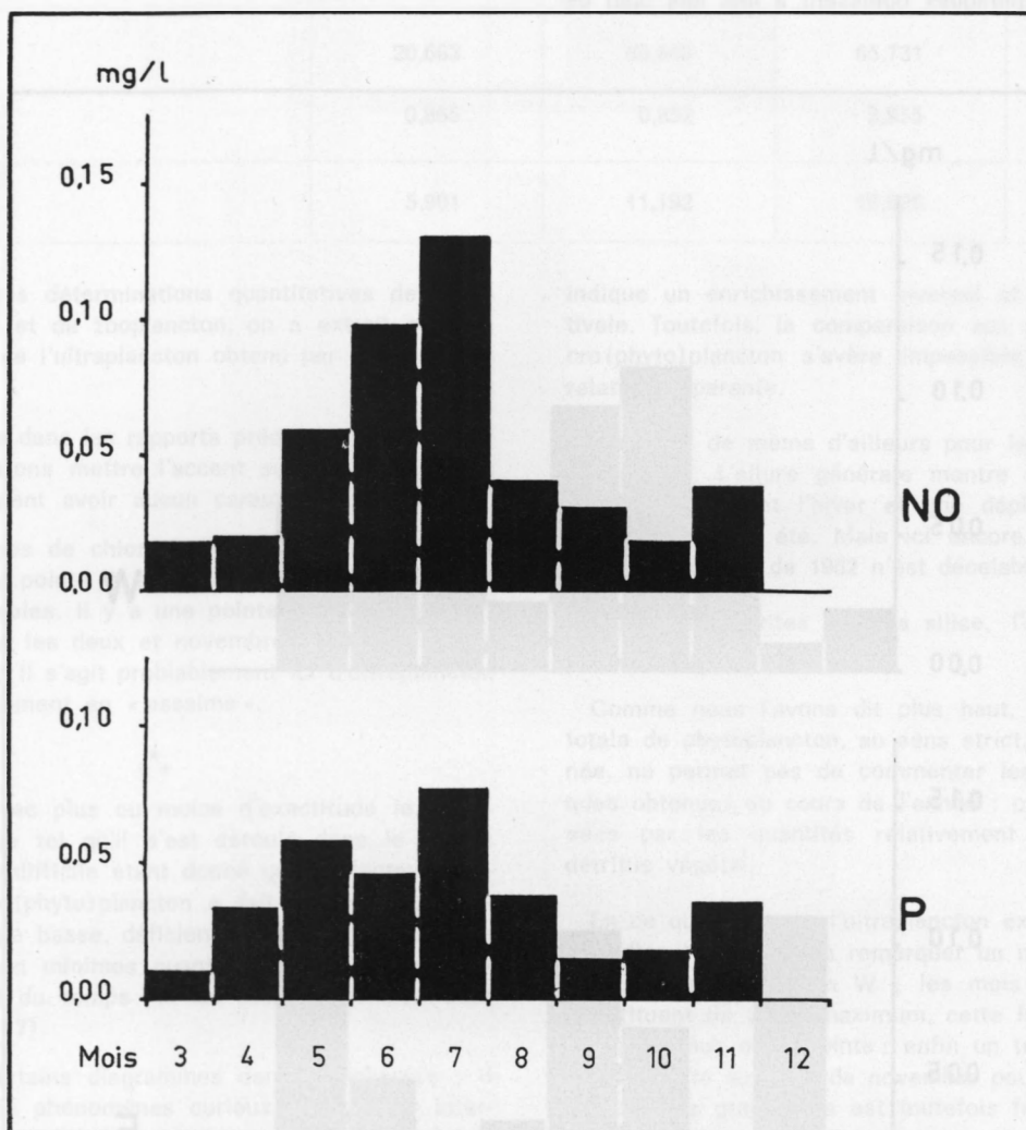
Fig. 16 — Chlorophylle en mg/litre — Moyennes mensuelles, points NO et P.
