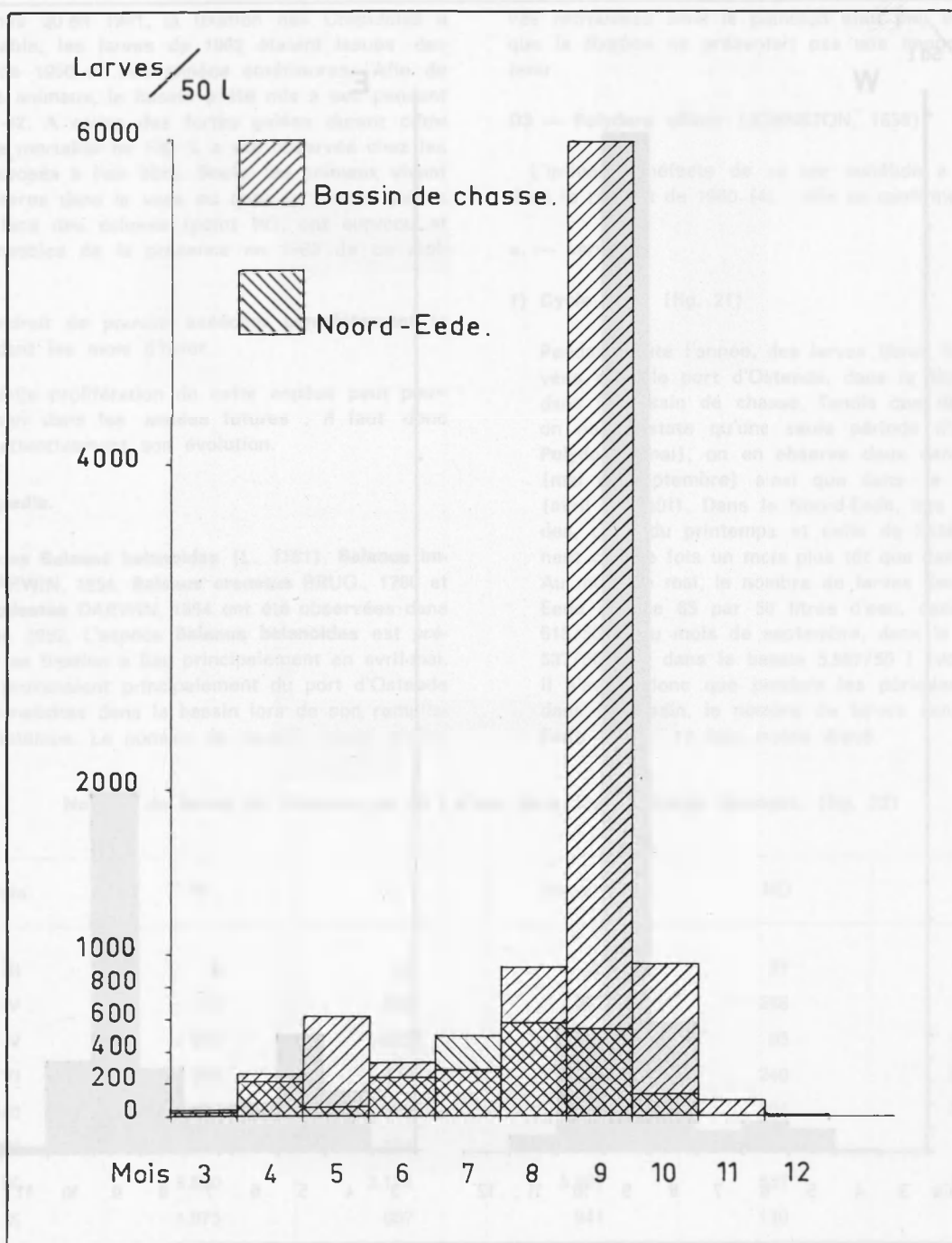
Fig. 22 — Nombre moyen de larves de Polydora par mois et pour 50 l d'eau, dans le bassin de chasse et dans le Noord-Eede.
