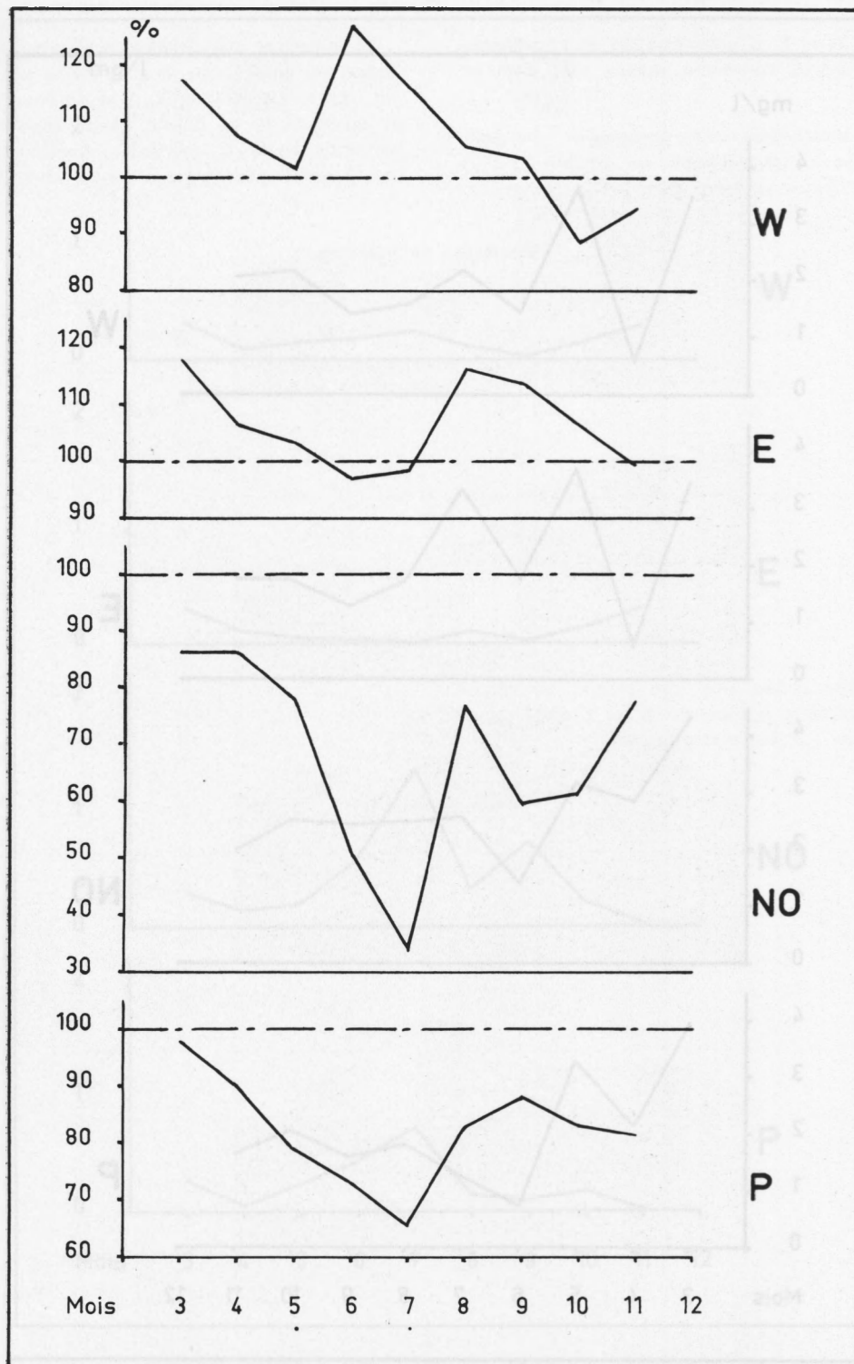
Fig. 6 — Oxygène % saturation — Moyennes mensuelles.
