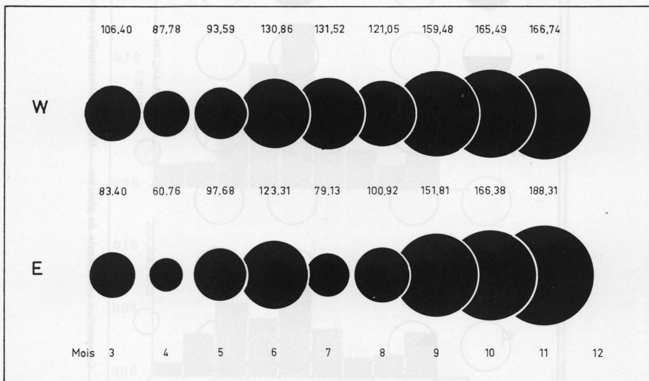
Fig. 18 — Index de qualité — Moyennes mensuelles, points W et E.
