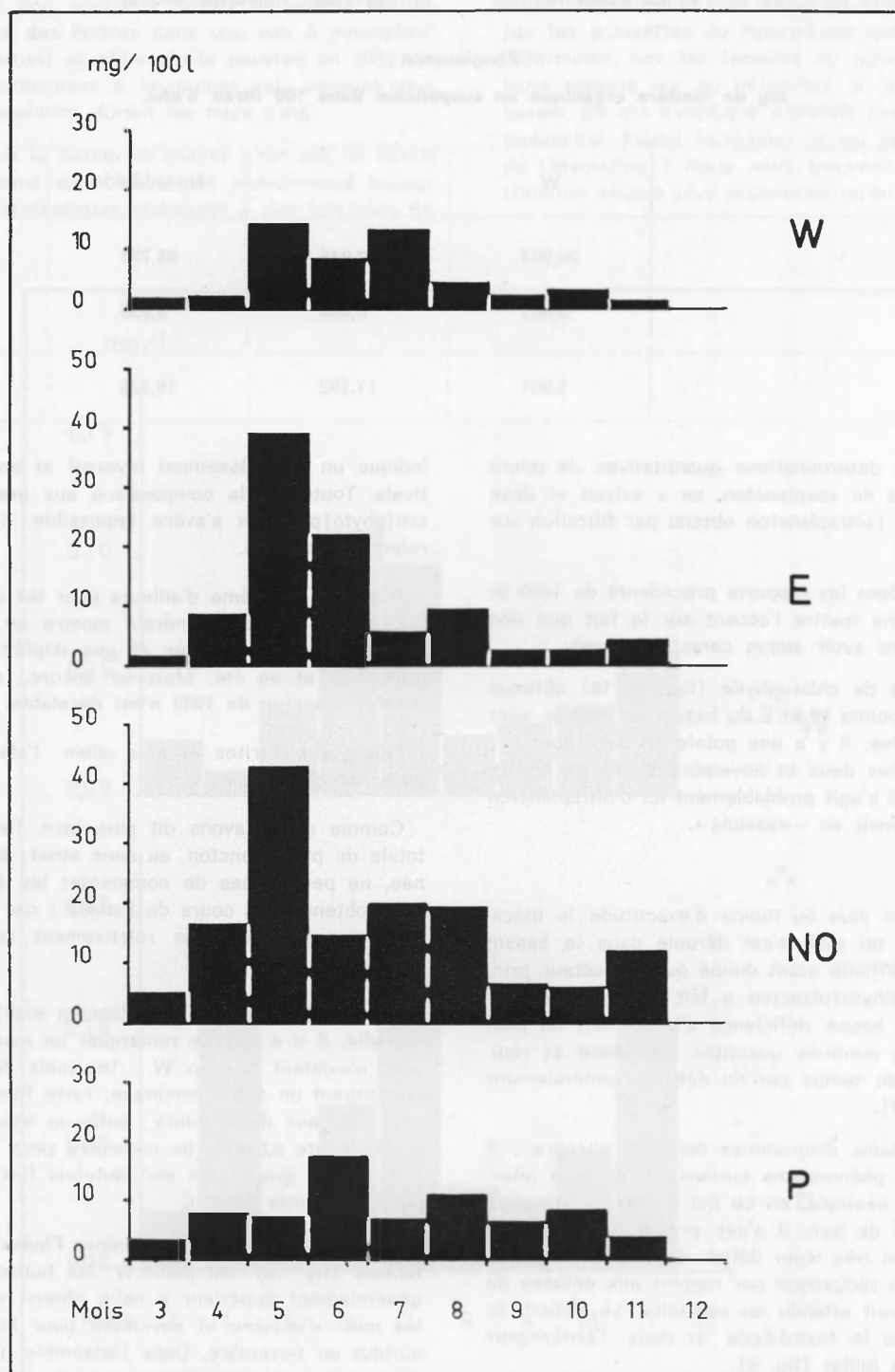
Fig. 14 — Zooplancton — Matières organiques en mg/100 l : Moyennes mensuelles.
