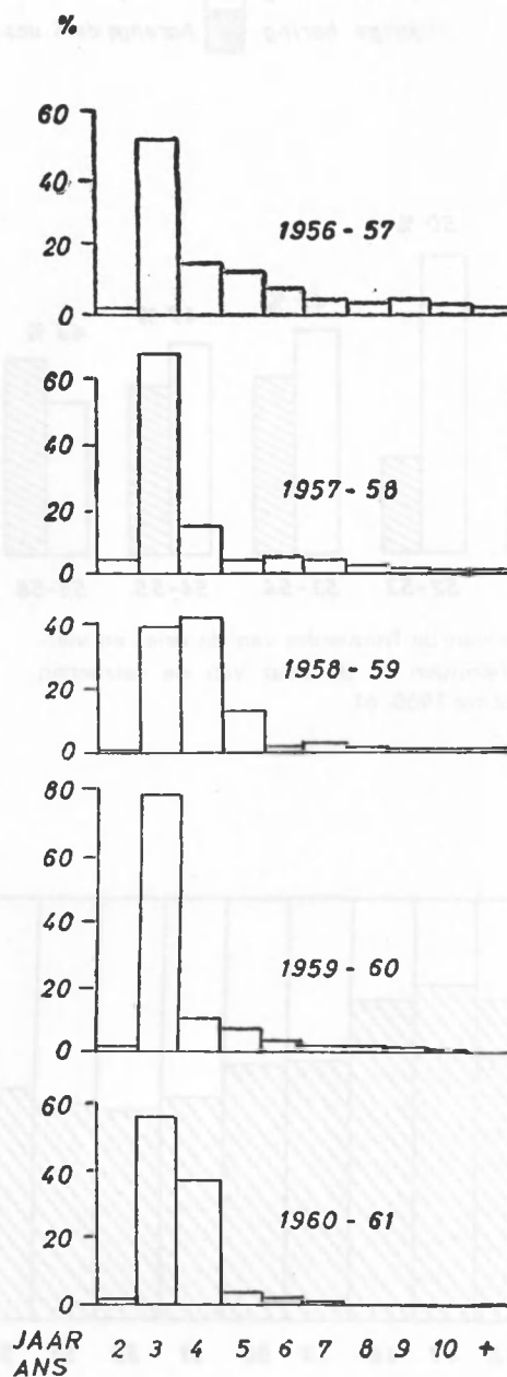
Fig. 1 — Escalier biologique des concentrations de harengs au cours de la période 1951-'52 à 1960-'61.
