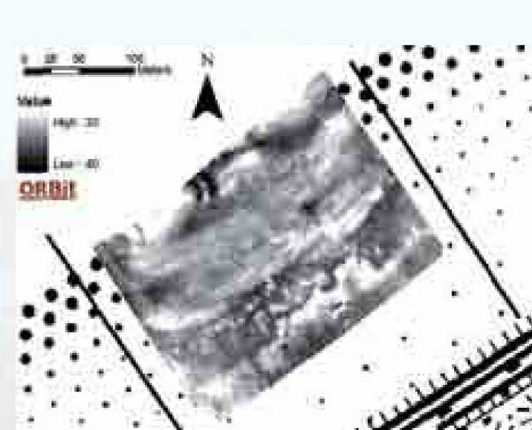
↑ De opgemeten zone tussen de golfbrekers en de variatie in schijnbare elektrische geleiding tot op een diepte van ongeveer 0,5 m. (BE). © Orbit/A2S
