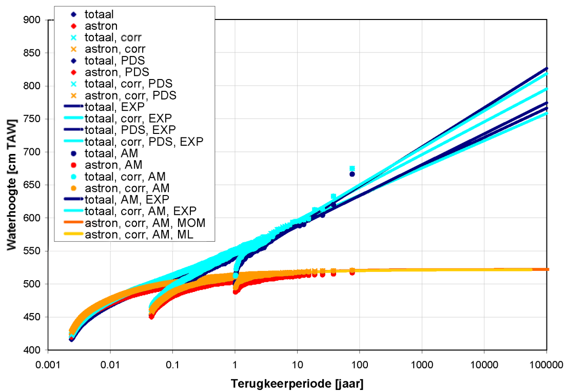
Figuur 4. Totale waterhoogte en astronomische component versus terugkeerperiode
