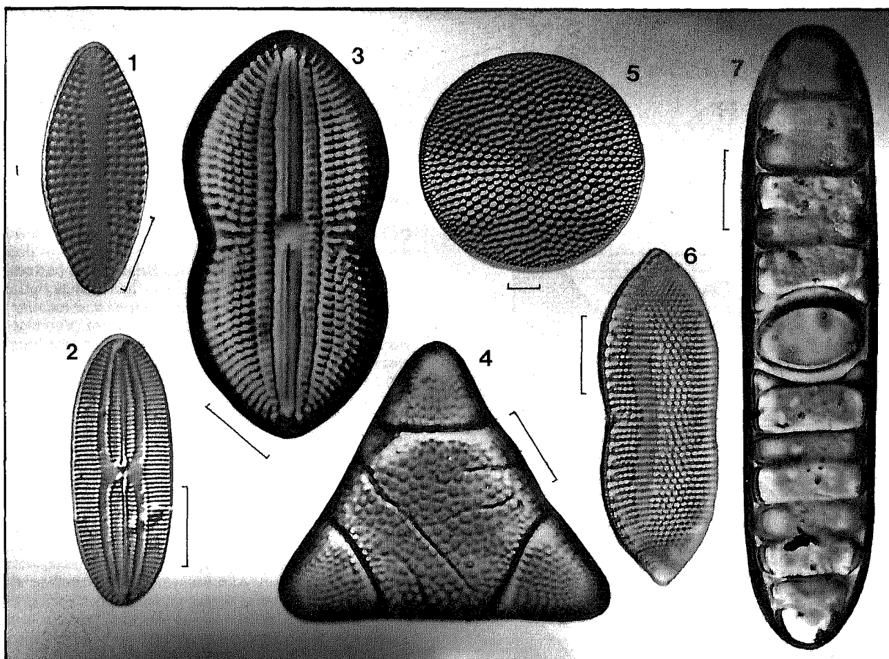
Afb. 6. Enkele mariene diatomeeën (L.M.). Marien-brak: 1. Delphineis surirella . 2. Navicula forcipata . Marien: 3. Diploneis bombus . 4. Biddulphia alternans . 5. Coscinodiscus apiculatus var. ambigua . 6. Nitzschia panduriformis . 7. Grammatophora serpentina . Herkomst: België, Holoceen.
