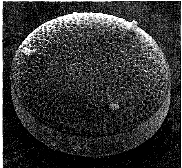
Afb. 2. De centrische diatomee Aulacodiscus argus (S.E.M.). Herkomst: België, Holoceen.
