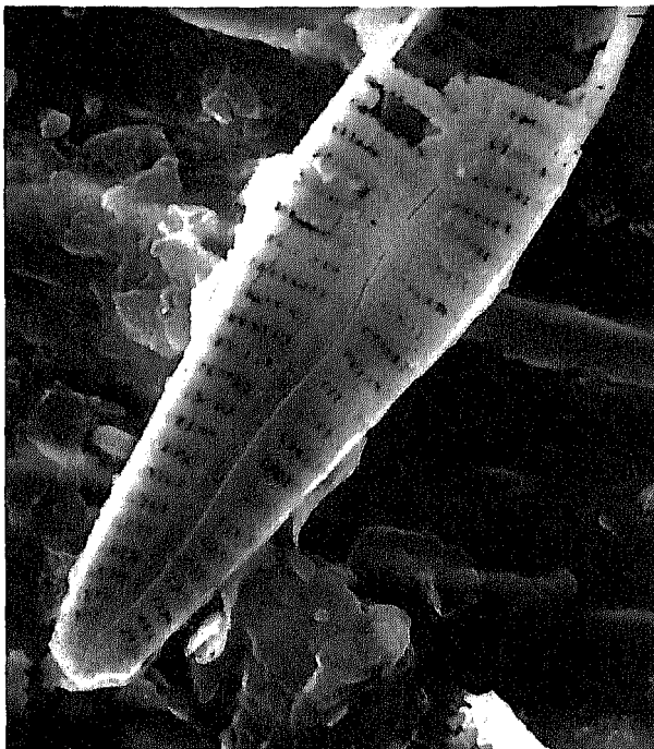
Afb. 1. Kiezelskelet van Gomphonema affine (S.E.M.). Een gedeelte van het bovenste schaal is weggebroken zodat de binnenzijde zichtbaar is. Herkomst: België, Holoceen. De maatstreep bij de figuren geeft steeds 10 micrometer weer.
