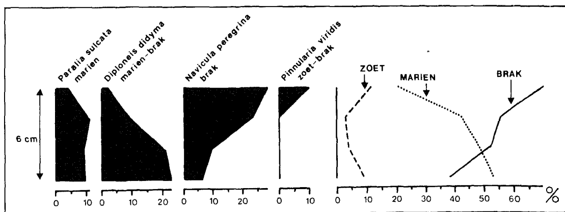
Afb. 10. Evolutie van de belangrijkste soorten evenals van het globale aandeel van zoetwater-, brakwater- en mariene diatomeeën in een kleig laagje uit een veenpakket uit de westelijke Belgische kustvlakte. De percentages berusten op tellingen van meer dan 500 schaaltes per niveau.
