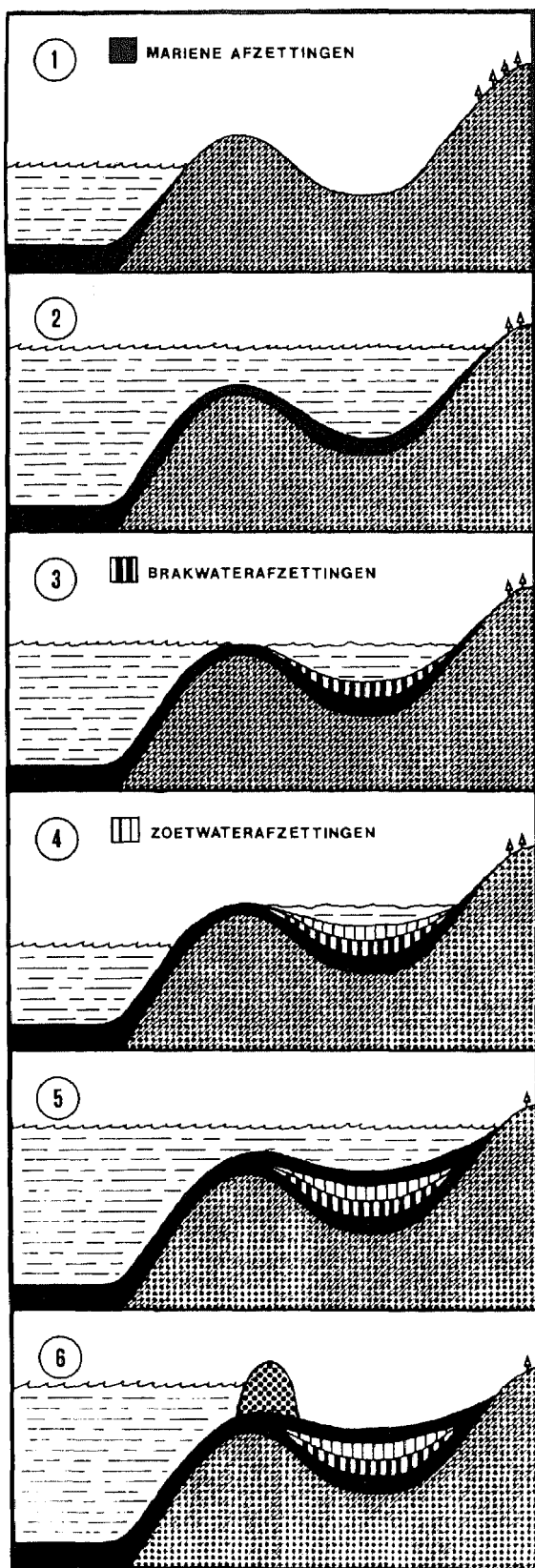
Afb. 8. Vereenvoudigde evolutie van een kustgebied bij een veranderlijke zeespiegel. Verklaring zie tekst (gedeeltelijk naar Kjemperud, 1981).
