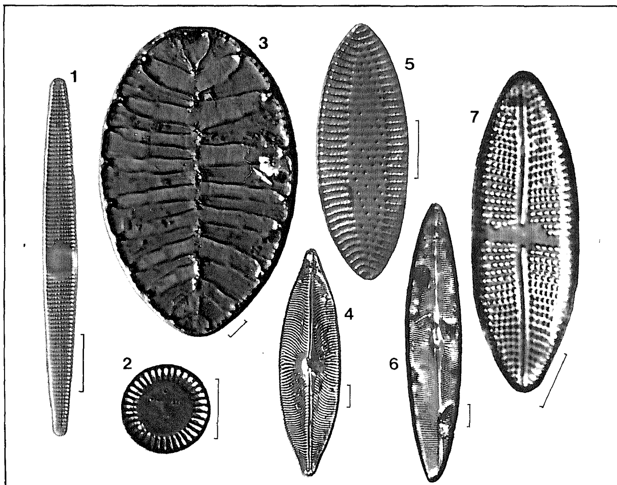
Afb. 5. Enkele brakwaterdiatomeeën (L.M.). Brak-zoet: 1. Fragilaria pulchella . 2. Cyclotella meneghiniana . Brak: 3. Surirella striatula . 4. Pinnuavis elegans . 5. Nitzschia navicularis . Brak-marien: 6. Scoliopleura tumida . 7. Achnantes brevipes . Herkomst: België, Holoceen.
