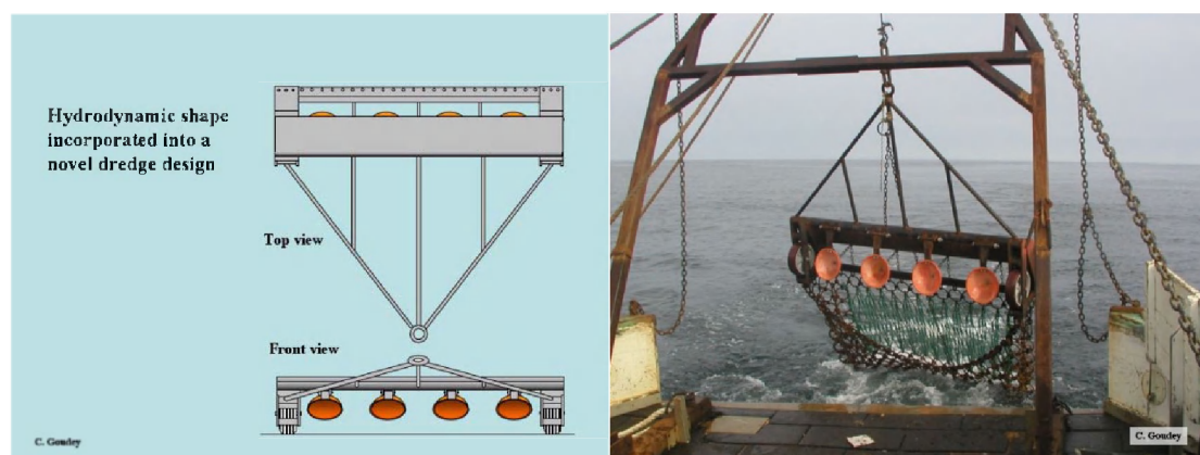
Figuur 1-4: Toepassing van bolcappen in een prototype schelpdierkor (bron: C. Goudey, M.I.T. Boston, USA)
