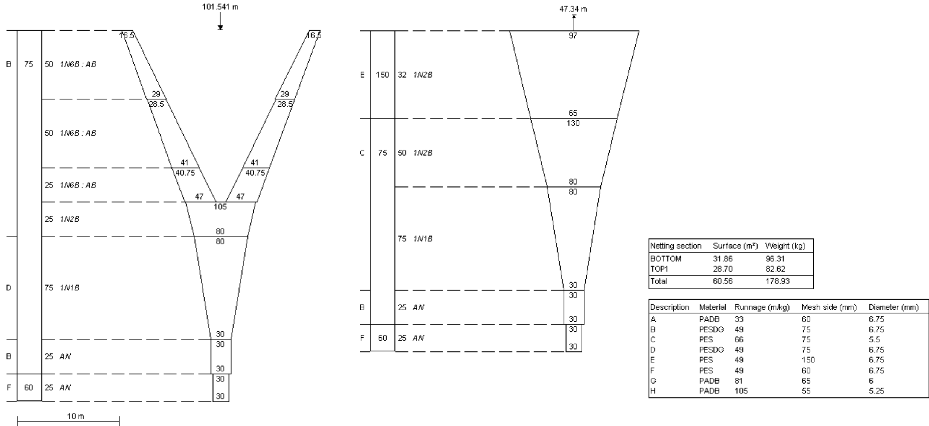
Figuur 9-1: Nettetekening in DynamiT™ van het originele boomkornet van de FD-281
