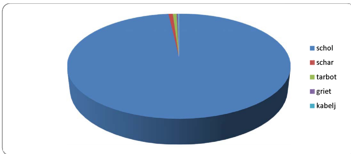
Figuur 4-32: Gemiddelde samenstelling van de aangevoerde vis (27 trekken).
