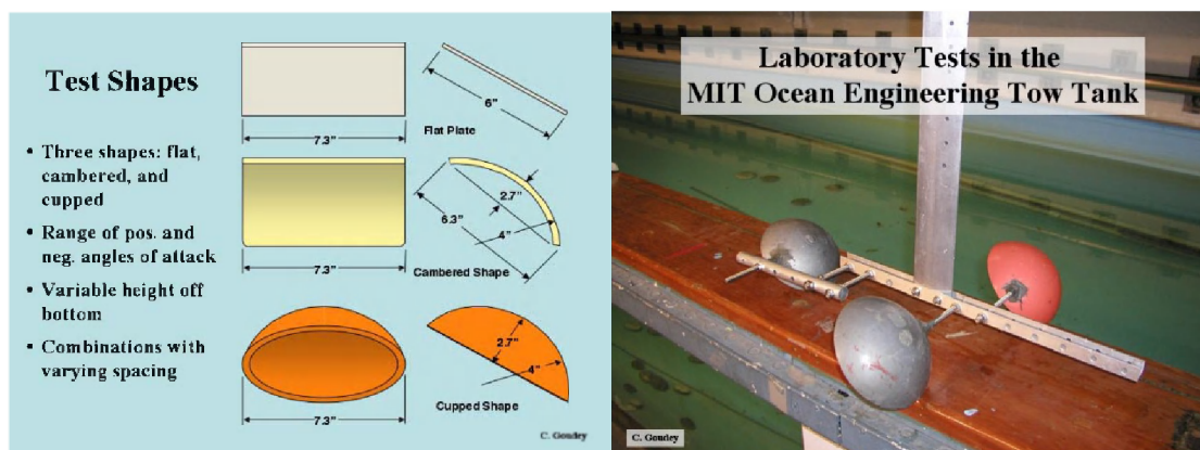
Figuur 1-3: Experimenten aan wervelwerking (bron: C. Goudey, M.I.T. Boston, USA)
