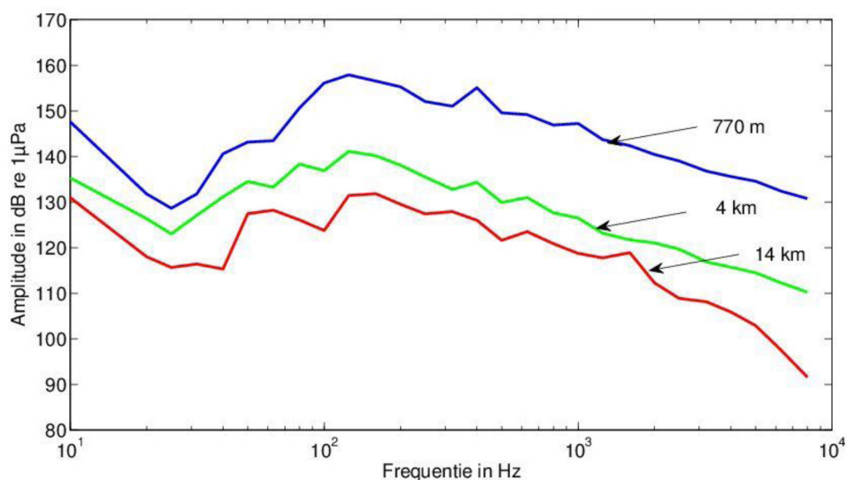
Figuur 3.7: Pieken in het onderwatergeluid (1/3 octaafband spectrum) gemeten op drie afstanden van de Blybank, tijdens het heien van de fundering voor een windturbine.
