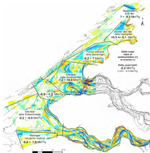
Figuur 3.3: Getallen per deelgebied in \text{Mm}^3/\text{jaar} voor erosie en sedimentatie gedurende de periode 1976/1980 tot 2004 voor het Zeeuwse Deltagebiet. De gekleurde gebieden tonen erosie/sedimentatie over de periode 1964 tot 2004 (naar Cleveringa, 2008).
