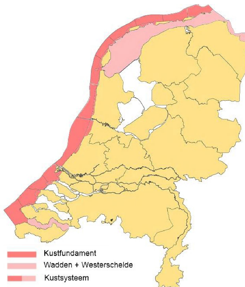
Figuur 1.1: Ligging van het Nederlandse kustfundament en van het Nederlandse kustsysteem. De duinen zijn onderdeel van zowel het kustfundament als van het kustsysteem
