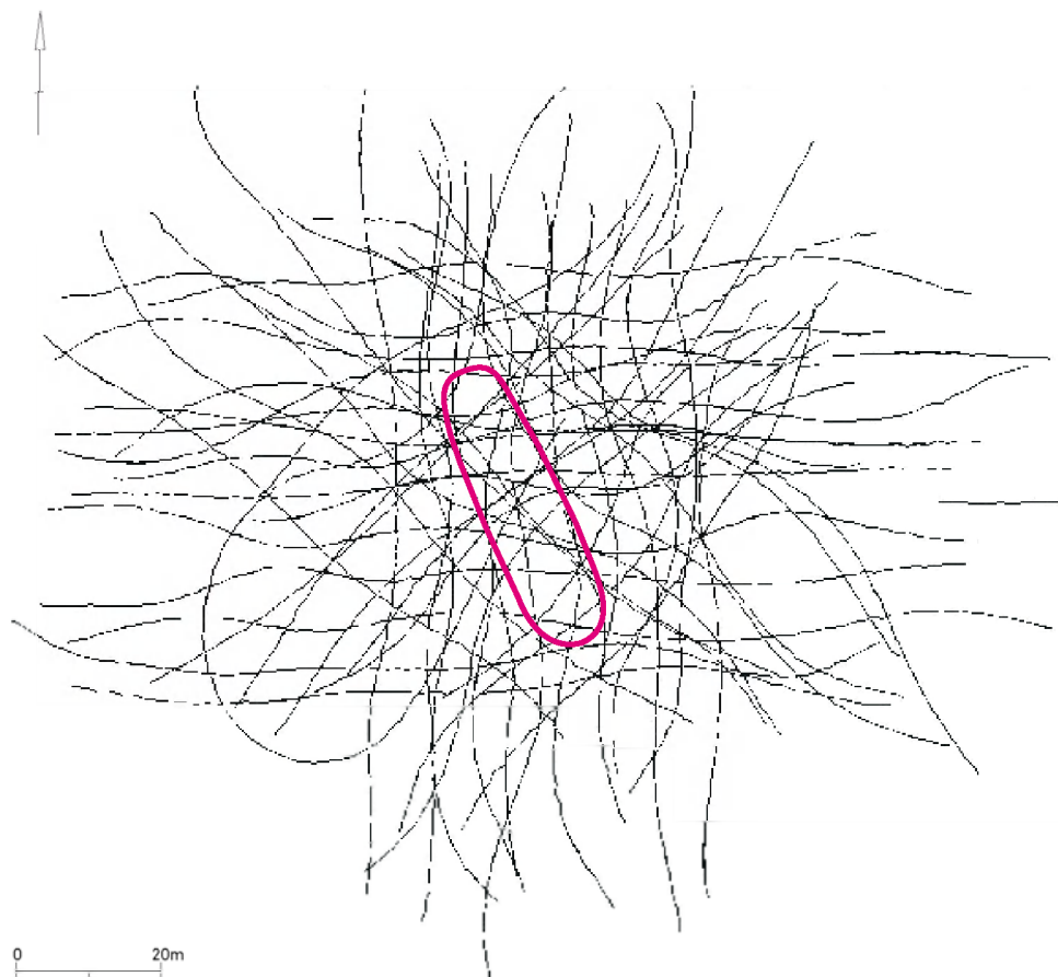
FIG. 10 Seismic network recorded over the wreck site of 't Vliegende Hart in 2010. The red ellipse marks the (supposed) location of the wreck. In total 49 profiles were recorded crossing the wreck at different angles. Seismisch netwerk opgenomen over het wrak van 't Vliegende Hart in 2010. De rode ellips markeert de (vermeende) locatie van het wrak. In totaal werden 49 profielen opgenomen die het wrak kruisen onder verschillende hoeken.
