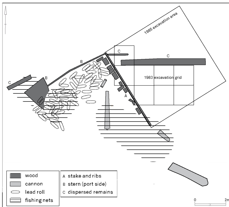
FIG. 5 Remains of t Vliegende Hart wreck site observed during diving investigations in 1983 (after Gawronski & Kist 1984). Structural fragments include a.o. wooden fragments of the stern (B) and hull (A). Nearby also several cannons and a large number of lead rolls were found, partly covered by fishing nets. The 1985 excavation area is also shown on the right (after Sills Consortium Recoveries Ltd 1985). Overblijfselen van het wrak van 't Vliegende Hart zoals blootgelegd tijdens het duikonderzoek in 1983 (naar Gawronski & Kist 1984). Houten fragmenten van de opbouw zijn o.a. afkomstig van de achtersteven (B) en de scheepsrump (A). Vlakbij werden ook een paar kanonnen en een groot aantal loden ballastrollen gevonden, gedeeltelijk bedekt door vissersnetten. Het opgravingsgebied uit 1985 is ook aangeduid rechts (naar Sills Consortium Recoveries Ltd 1985).
