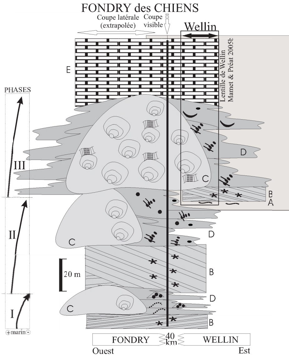
Figure 4 : Modèle sédimentaire de la lentille biohermale. Position interprétée des deux coupes, à gauche coupe du 'Fondry des Chiens' et interprétation des faciès latéraux avec deux lentilles non exposées, à droite coupe de Wellin (in Mamet & Prétat, 2005b). Les lettres A à E correspondent aux environnements majeurs (se reporter au texte) se succédant suivant les trois phases régressives I, II et III. Se reporter à la figure 3b pour la légende des symboles. Sedimentary model of the biohermal lens with interpreted position of two sections, on the left, the 'Fondry des Chiens' section with its two inferred and unexposed lateral biohermal lenses, on the right, the Wellin section (in Mamet & Prétat, 2005b). Bold A to E letters represent the major environments (see text) occurring through the succession of regressive phases I, II and III. Symbols legend to be found in figure 3b.
