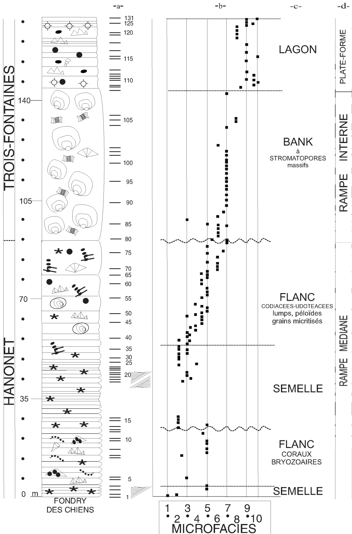
Figure 2 : Log stratigraphique de la coupe du 'Fondry des Chiens'. Colonne a = position des échantillons prélevés (pétrographie), Colonne b = séquence standard des microfaciès 1 à 10 (cf texte pour la description), Colonne c = environnements, Colonne d = système sédimentaire. Se reporter à la figure 3b pour la légende des symboles. Stratigraphic log of 'Fondry des Chiens' section. Column a = position of the studied sample (petrography), Column b = standard sequence of microfacies 1 to 10 (see text for description), Column c = environments, Column d = sedimentary systems. Symbols legend to be found in Fig. 3b.
