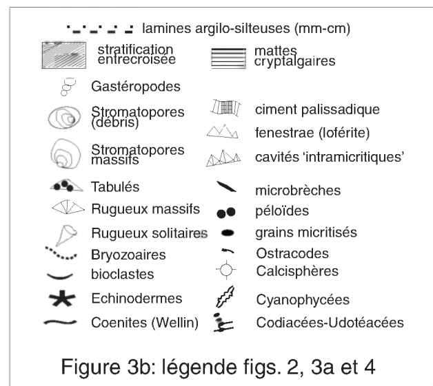
Figure 3b : Légende des figures- legend of figures.
