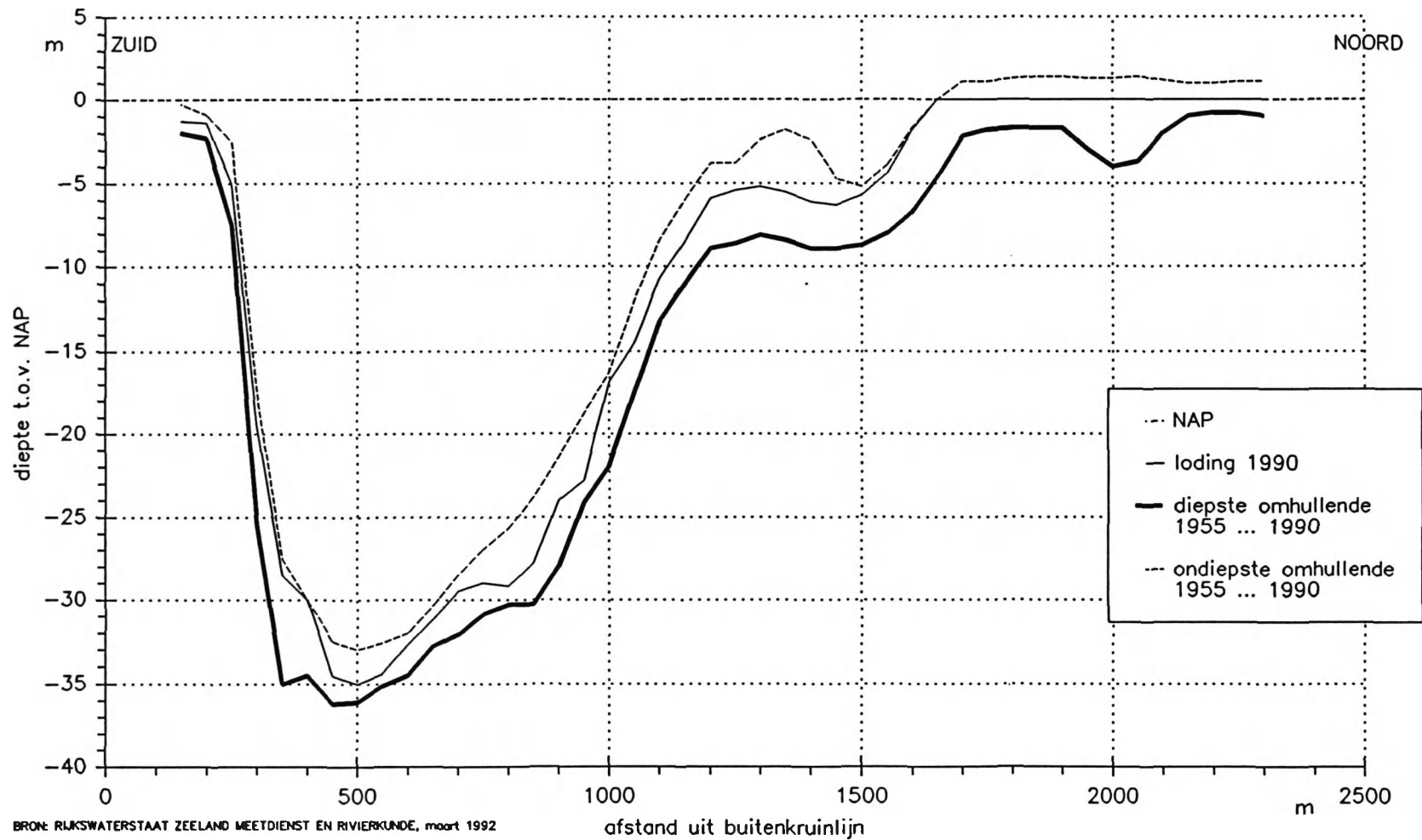
WOV-tracé 3, boortunnel; omhullenden van de ladingen uit 1955 ... 1990 in de Pas van Terneuzen
