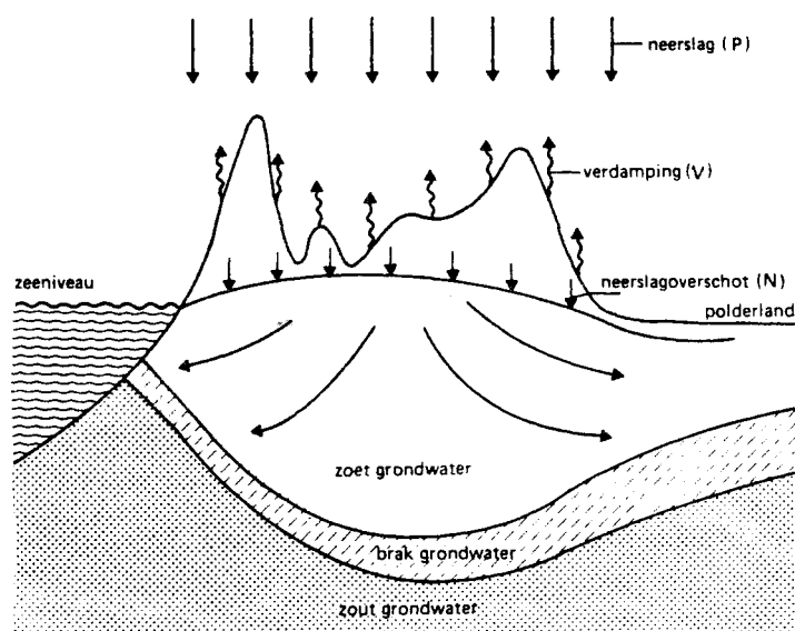
Fig. II.1. Geschematiseerd grondwaterstromingsmodel van het duinmassief (de horizontale schaal werd sterk samengedrongen) (naar Bakker, 1981).
