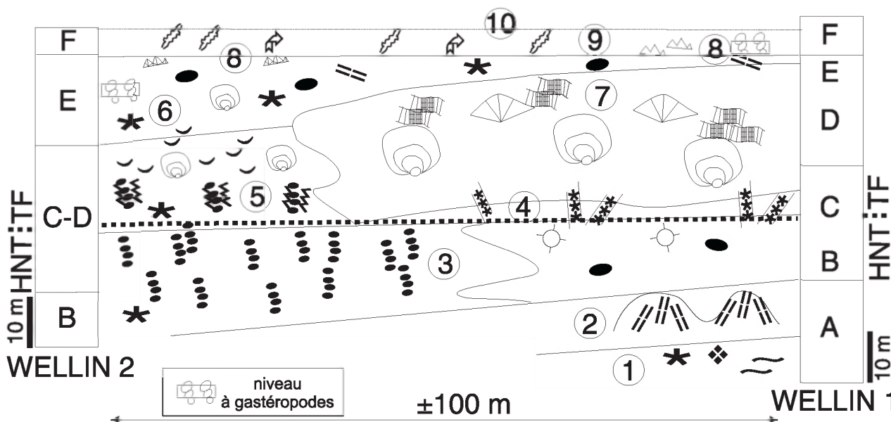
Figure 6 : Diagramme de corrélation lithostratigraphique des deux coupes. Les lettres majuscules correspondent aux environnements mentionnés aux figures 2 et 3. Les chiffres encadrés sont les 10 microfaciès de la figure 4a. Abréviations : HNT = Formation de Hanonet, TF = Formation de Trois-Fontaines. La limite entre ces deux formations est placée arbitrairement à la base de la semelle et de ses faciès latéraux. Se reporter à la figure 4b pour la légende des symboles.
