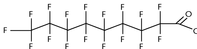
PFOA
