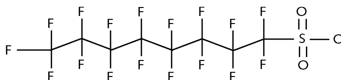
PFOS
