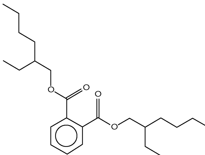
Figuur 1. DEHP
