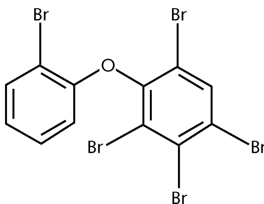
Figuur 2. Pentabroomdifenylether
