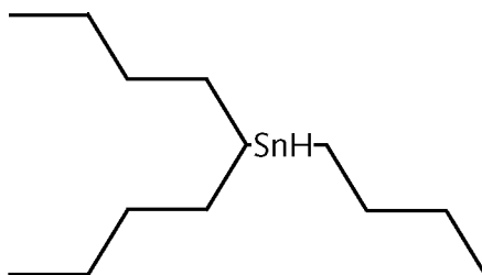
Figuur 3. Tributyltin
