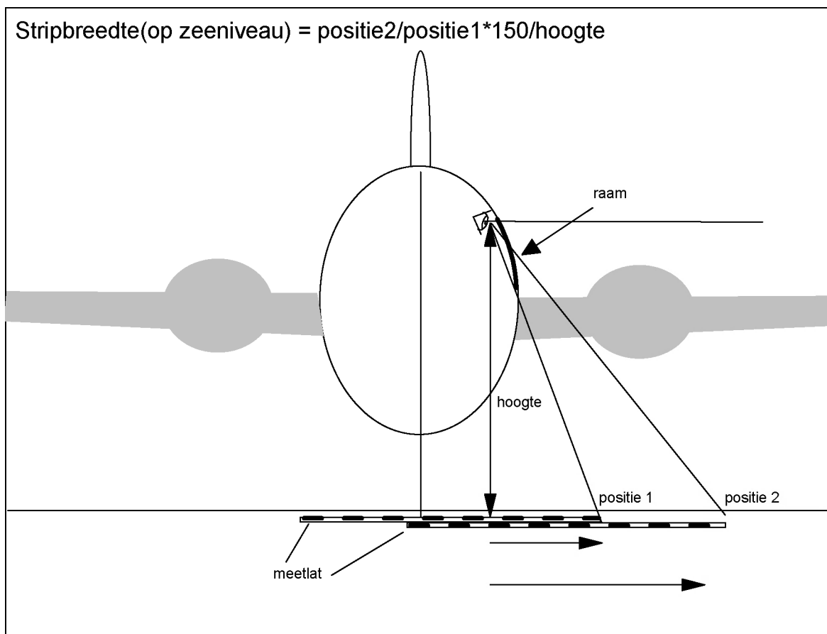
Figuur 12c. metingen aan stripbreedte in een hangar
