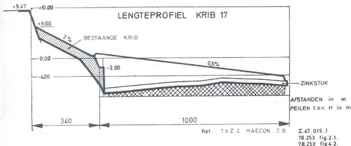
Figuur 4.1 : Ontwerp uit 1978 van strekdam voor oostkust [R17]
