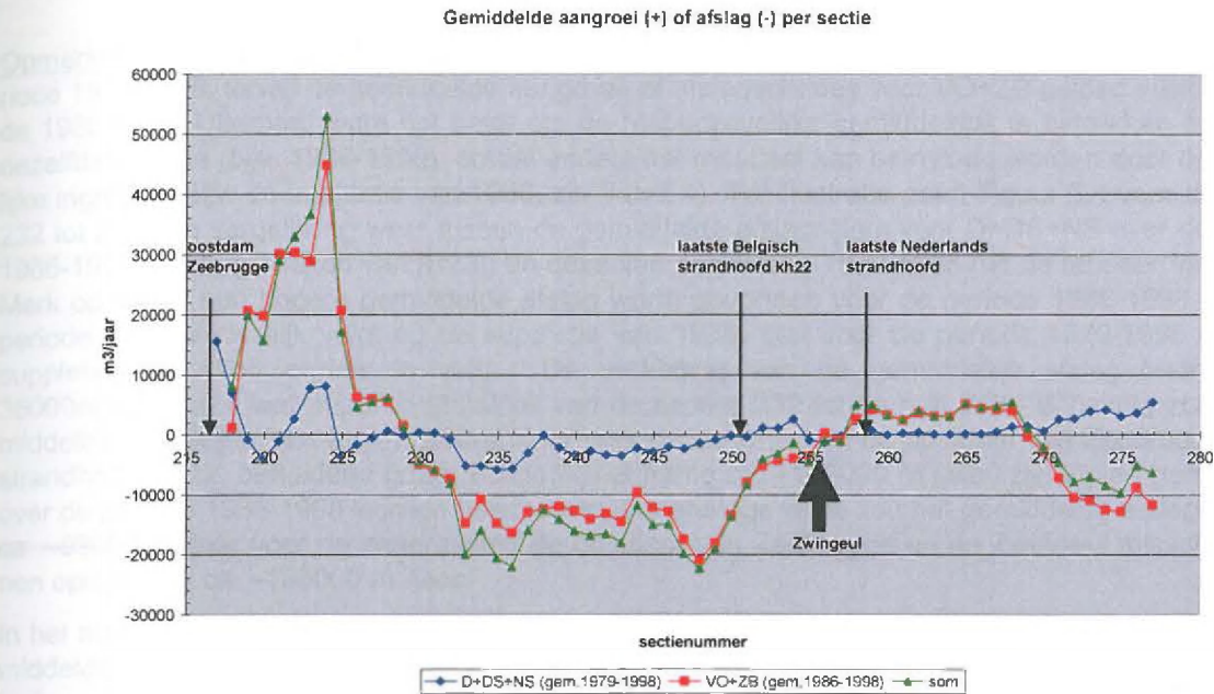
Figuur 3.3: Gemiddelde jaarlijkse aangroei- of afslagvolumes per kustsectie (bron: [R23] en [R22])
