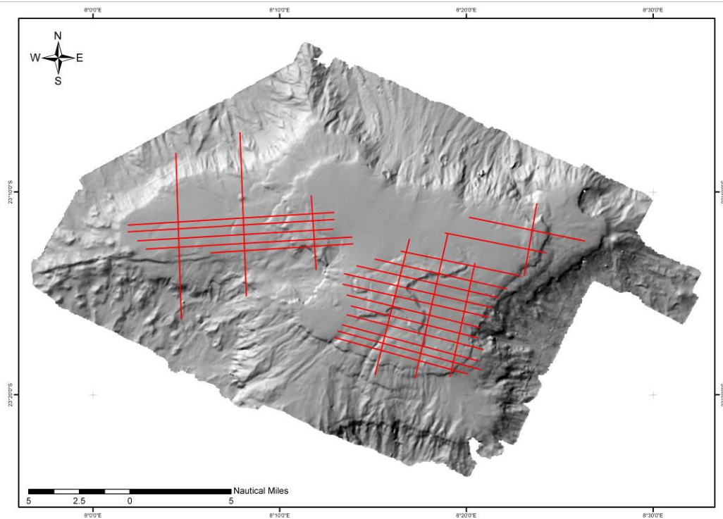
Figura 6.2: Diseño de líneas de navegación para prospección sísmica de la zona del Monte de Ewing con la sonda paramétrica TOPAS / Navigation lines design for seismic exploration of the Ewing Seamount using parametric sounding (TOPAS).
