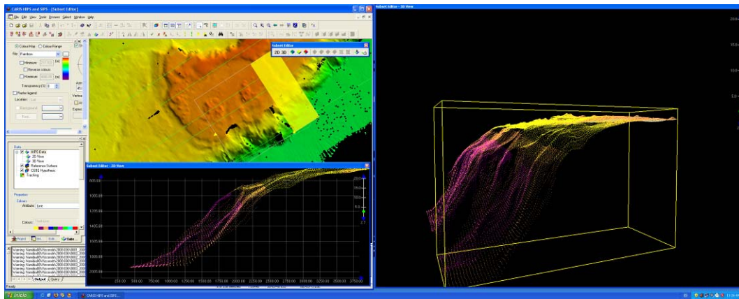
Figura 2.3: Pantalla de trabajo del modulo “Subset Editor” con vistas en 2D y 3D con las sondas pertenecientes al área seleccionada para limpiar / Work screen of the Subset Editor module with 2D and 3D views with the sound to be cleaned.
