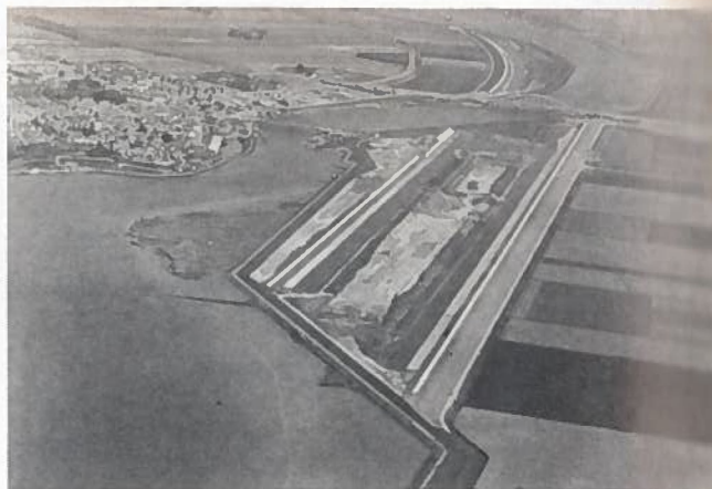
Figuur 63. Overzicht van de uitgevoerde werken vanuit het zuiden.
