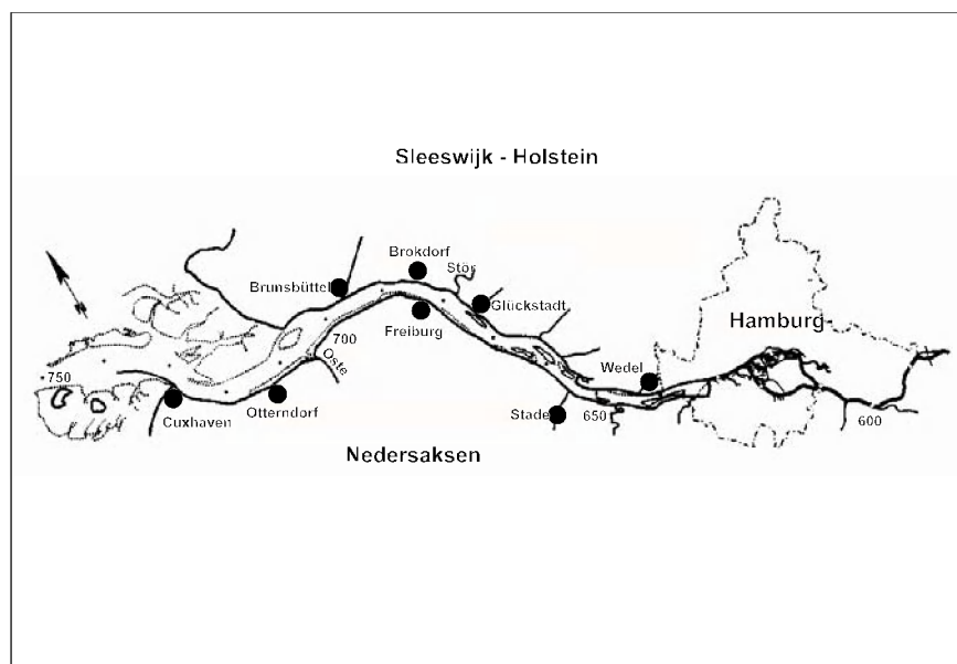
..... Figuur 3 Het Elbe-estuarium in Noord- Duitsland.
