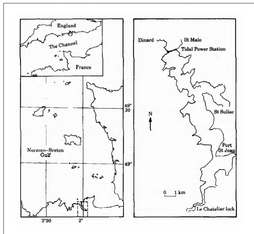
Figuur 4 Het estuarium van La Rance in Frankrijk
