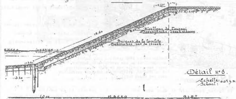
Doorsnede van de dijk te Heist 1860-1890
