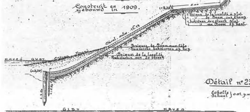
Doorsnede van de zeedijk in het Zoute voltooid in 1909.
