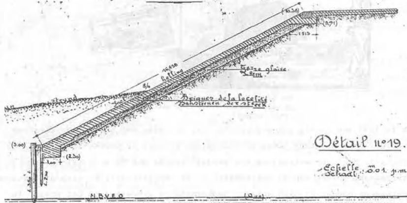
Doorsnede van de dijk te Knokke uit 1894
