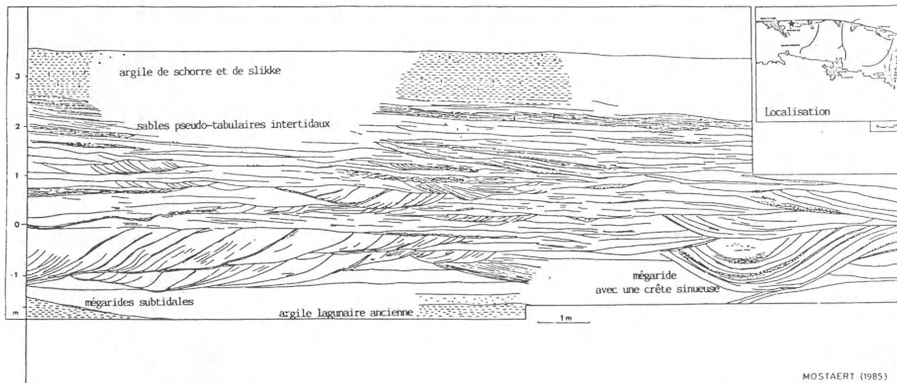
Fig. 4c : Séquence typique d'un remplissage d'un chenal de marée à Bredene, avec une couverture de sédiments de slikke et de schorre.
