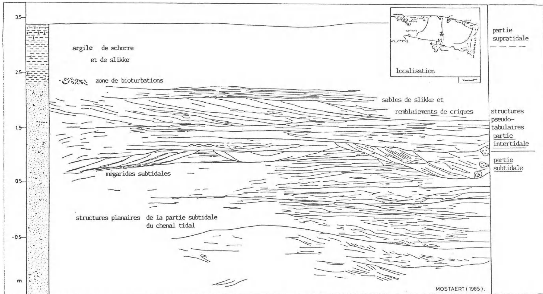
Fig. 4b : Séquence typique d'un remplissage d'un chenal de marée au Nord de Bruges, avec une couverture de sédiments intertidaux de slikke et de schorre.
