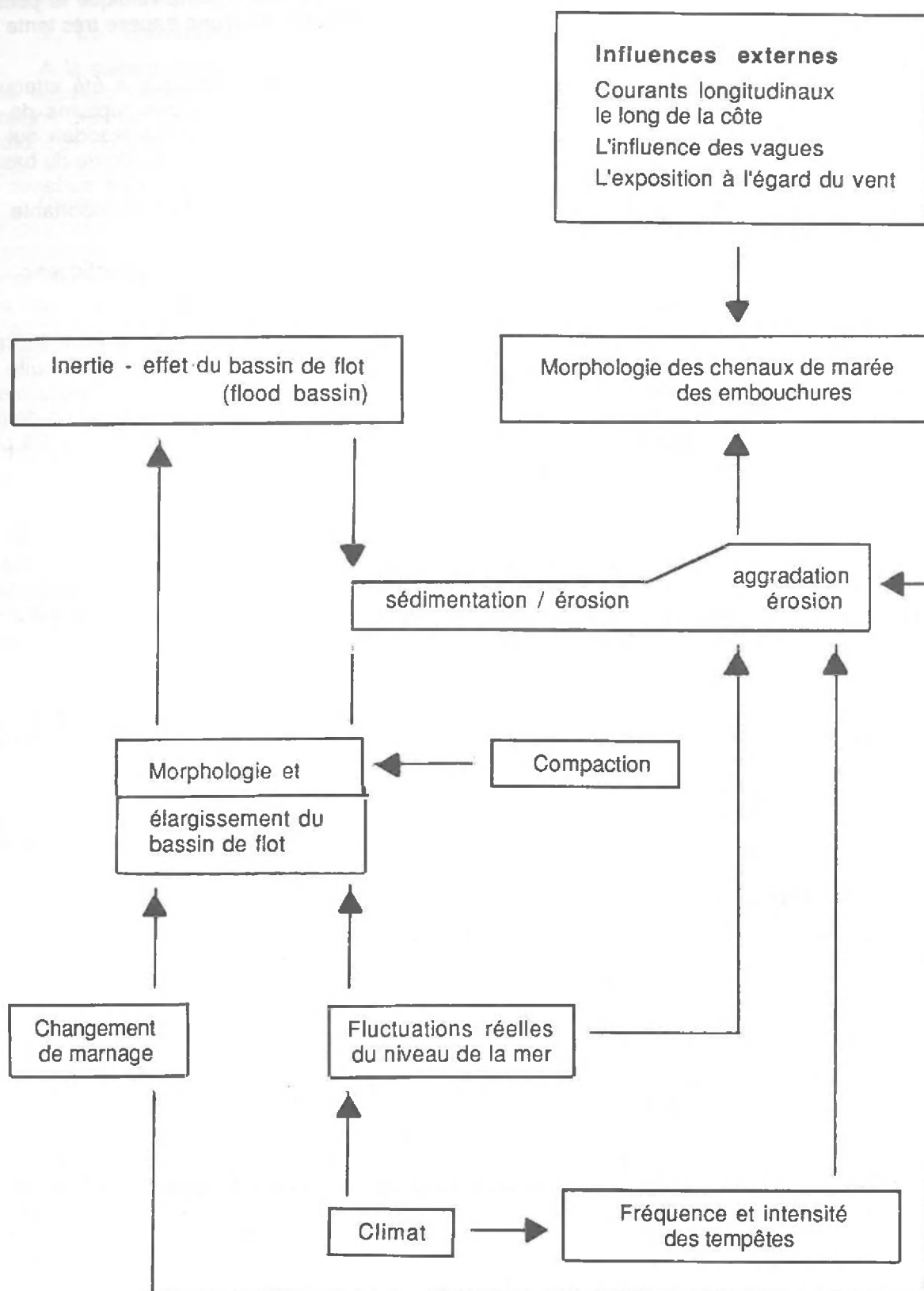
Fig. 6 : Interaction des facteurs qui influencent les niveaux de la mer dans la zone infra - littorale.
