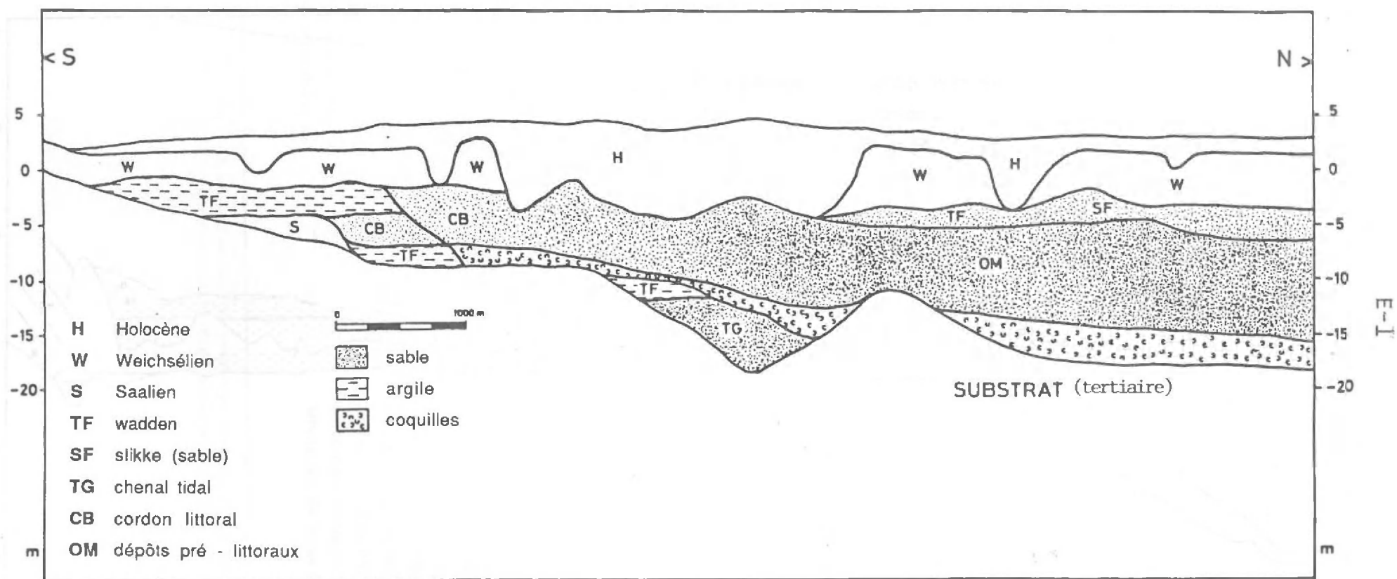
Fig. 3a : Les séquences éémiennees
