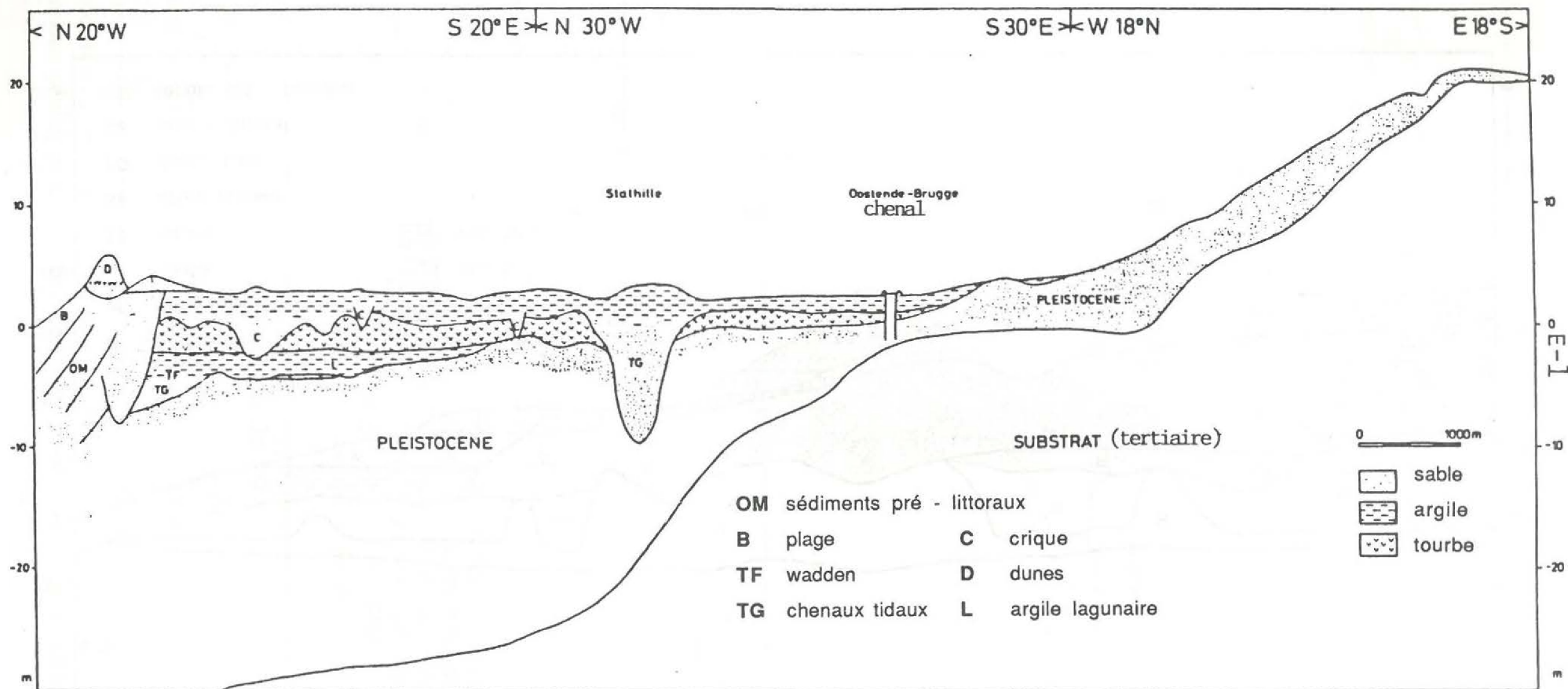
Fig. 3b : Les séquences holocènes
