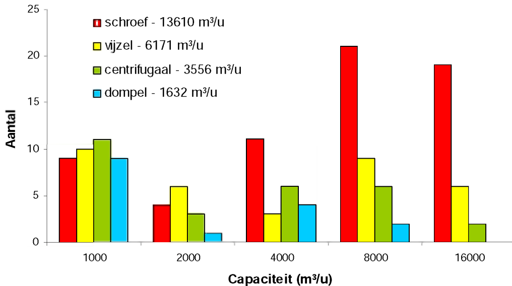
Figuur 5. Aantal pompgemalen per capaciteitsklasse (m³/u) en type pompemaal. In de legende wordt de gemiddelde capaciteit per type gegeven.
