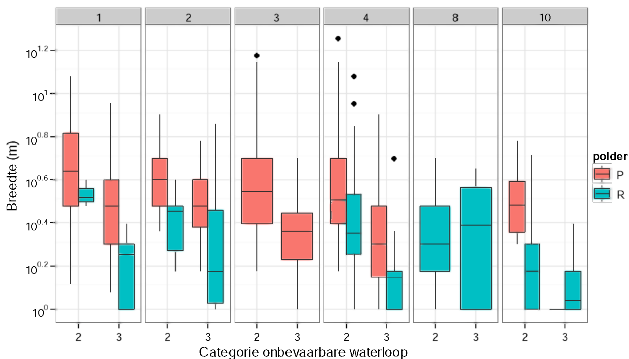
Figuur 2. Boxplots van de breedte van waterloopsegmenten per categorie (onbevaarbaar 2 en 3) en per bekken (1 = IJzer, 2 = Brugse polders, 3 = Gentse kanalen, 4 = Beneden-Schelde, 8 = Dijle, 10 = Nete).
