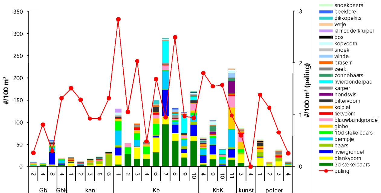
Figuur 10. Aantal vissen per 100 m² in de verschillende waterlooptypes van de rivierbekkens. De densiteit van paling wordt op de rechtse y-as weergegeven. Alleen de waterlooptypes die in de bemalingsgebieden voorkomen worden weergegeven.
