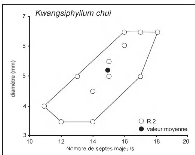
Figure 4-54: Diagramme de distribution du diamètre externe (en mm) en fonction du nombre de septes majeurs chez Kwangsiphyllum chui .
