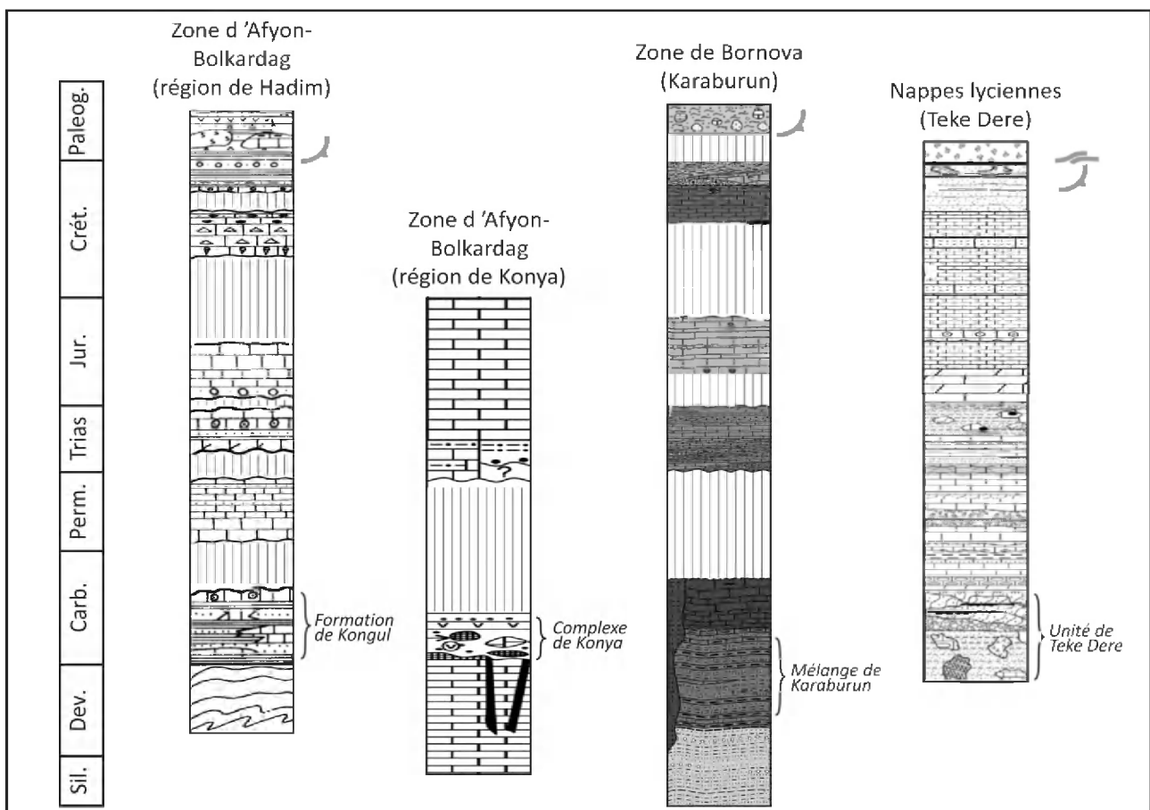
Figure 2-3: Colonne lithostratigraphique synthétique des Anatolides (Nappes Lyciennes, Zone de Tavşanlı, Afyon-Bolkardağ et Bornova). Modifié d'Özgül (1997: Hadım), de Robertson & Ustaömer (2009: Konya), de Çakmakoglu & Bilgin (2006: Karaburun) et Vachard & Moix (2011: Teke Dere). Légende en Figure 2-4.
