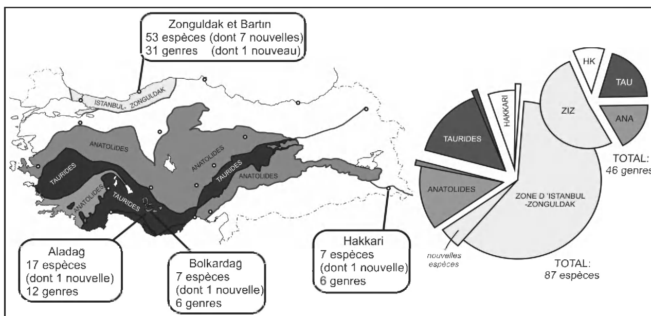
Figure 6-1: Synthèse graphique de la diversité des coraux tétracoralliaires au Carbonifère inférieur dans les quatre zones de Turquie traitées dans cette étude.
