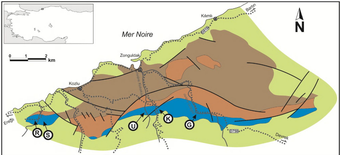
Figure 3-3: Carte géologique schématique de la région de Zonguldak dans le Nord-ouest de la Turquie. Modifié de Okan & Höşgör (2007). Légende: G : coupe de Gökgöl, K : coupe de Kokaksu, R : coupe de Kisla, S : carrière Sayılı, U : coupe d'Ulutam. La légende des couleur se trouve à la Figure 3-12).
