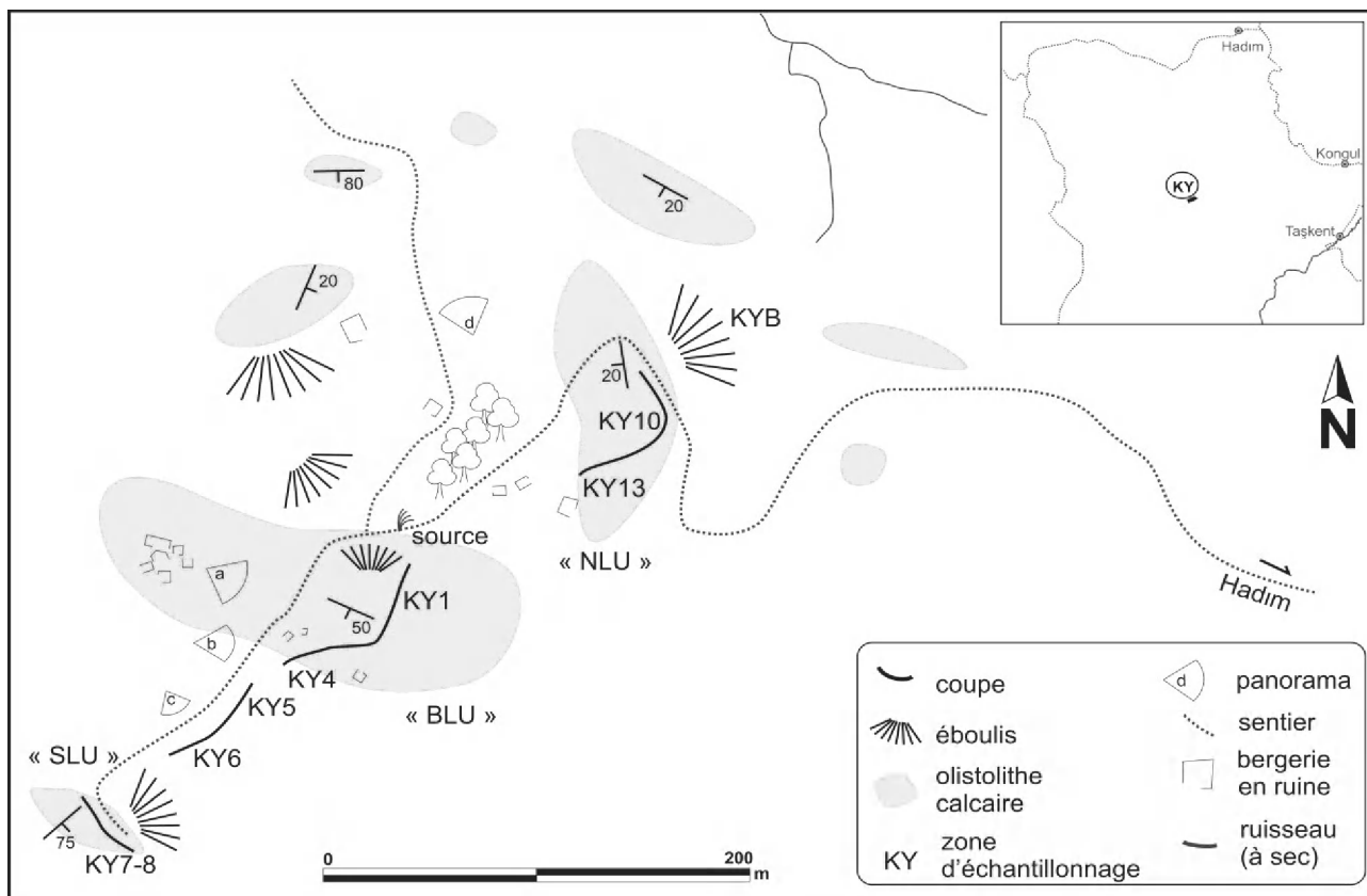
Figure 3-24: Carte de localisation de la coupe de Kongul Yayla dans les Anatolides centrales. Les panoramas font référence aux prises de vue des photographies présentées à la Figure 3-27.
