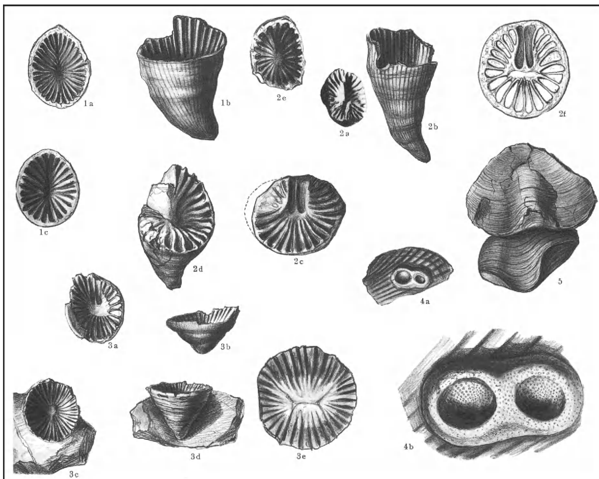
Figure 4-9: Coraux solitaires du Tournaisien de Yerköprü (Taurides orientales), Planche 4 de Frech (1916) reproduite à l'échelle 1/2. Les figures 1 et 2 sont potentiellement des Zaphrentites parallela .
