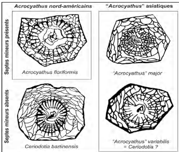
Figure 4-41: Comparaison des morphologies des polypiérites chez Ceriodotia , Acrocyathus (sens stricto, formes nord-américaines) et " Acrocyathus " asiatiques dont certaines espèces pourraient être classées dans le genre Ceriodotia . Explications dans le texte. Acrocyathus floriformis redessiné de Sando (1962, pl. 5, fig. 1), " Acrocyathus " major redessiné de Wu & Zhao (1989, pl. 33, fig. 1a), " Acrocyathus " variabilis redessiné de Wu & Zhao (1989, pl. 35, fig. 5).
