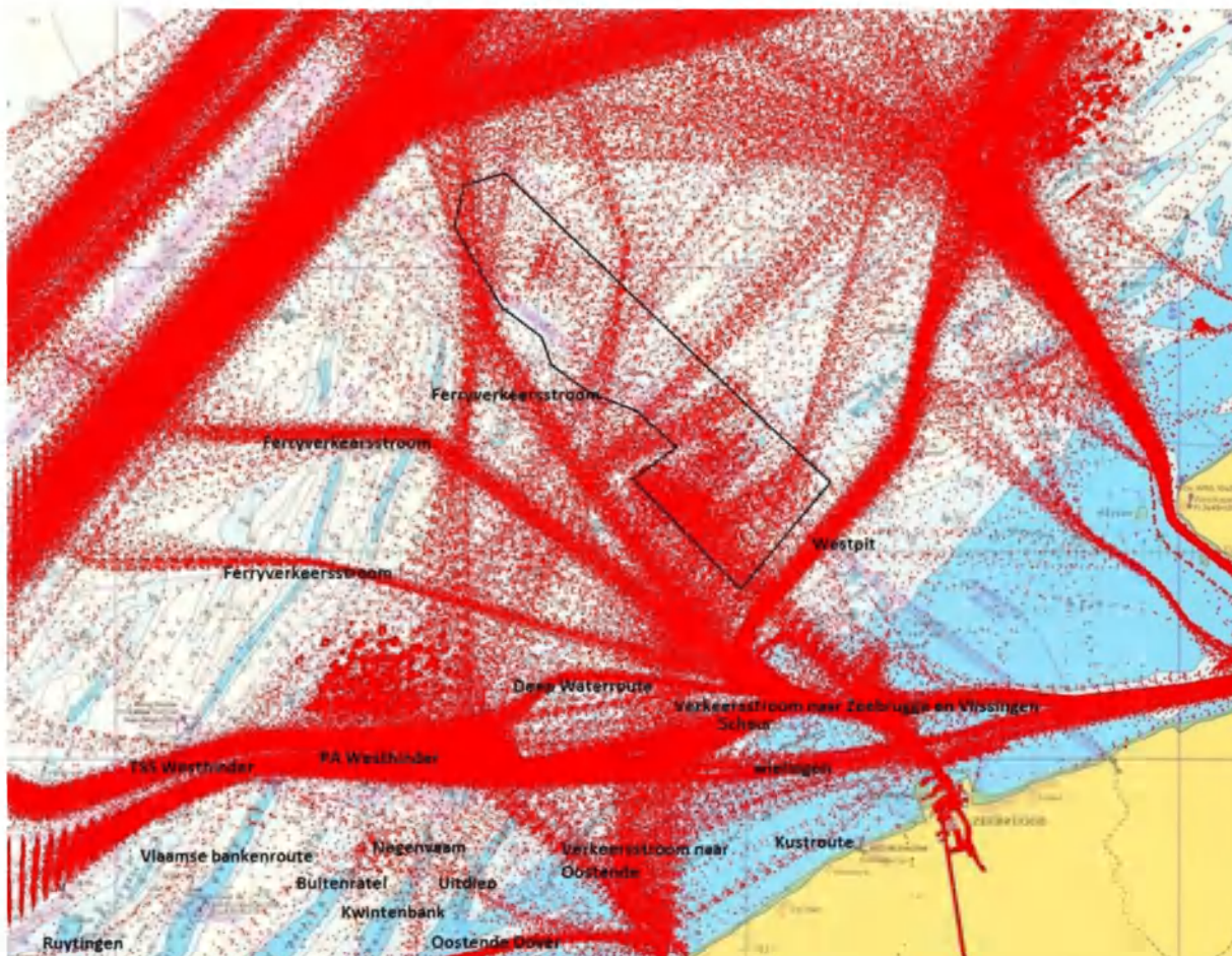
Figuur 25: AIS-gegevens Scheepvaart, periode juni 2012 [Bron: AIS DATA, Beheer- en Exploitatie Team Schelderadarketen].
