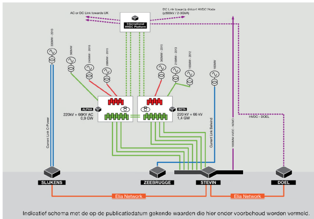
Figuur 42: Indicatief schema met de op de publicatiedatum gekende elektriciteitswaarden [Bron : Brochure Elia, Hoogspanningsnet in de Noordzee. Een toekomstvisie].
