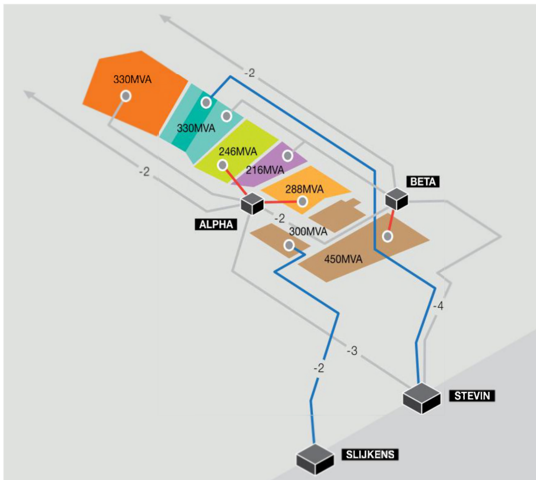
Figuur 43: Indicatief schema met de op de publicatiedatum gekende elektriciteitswaarden van de windmolenparken [Bron : Brochure Elia, Hoogspanningsnet in de Noordzee. Een toekomstvisie].
