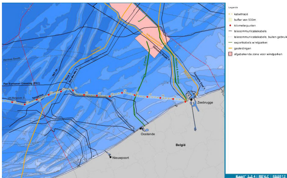
Figuren 40 en 41: Onderzoek naar Nemo-kabel [Bron: Elia, 2012].
