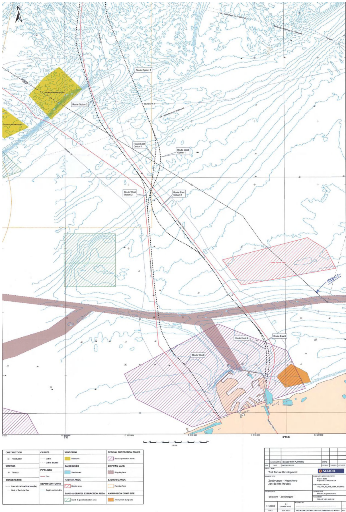
Figuur 45: Onderzoek nieuwe pijpleiding tussen Noorwegen en Zeebrugge: mogelijke tracés (de mogelijke tracés worden in zwarte stippellijn weergegeven) [Bron: Fluxys]
