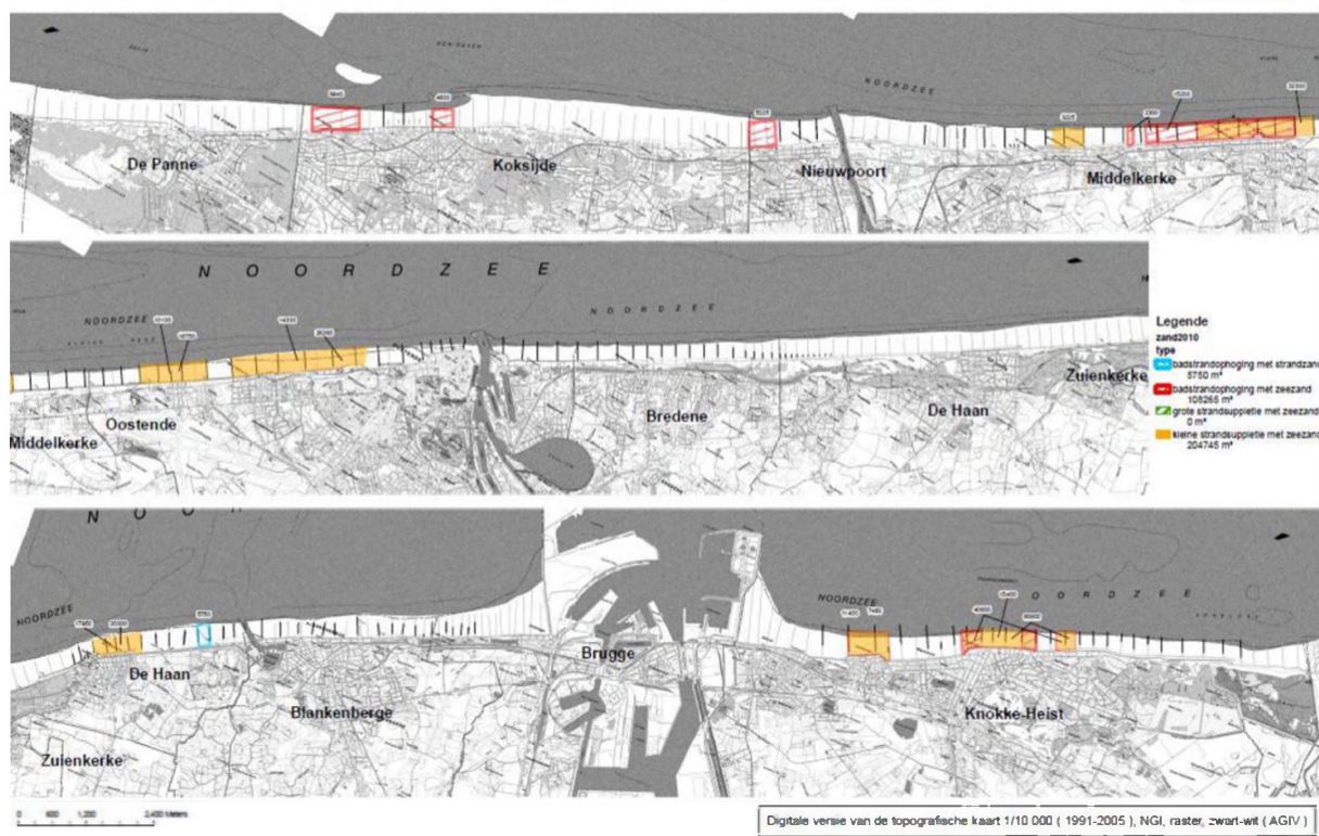
Figuur 20: Hoeveelheid gewonnen zand voor kustverdediging en strandsuppletie in 2010 [Bron: Afdeling Kust in: Belgische Staat, 2012. Socio-economische analyse van het gebruik van de Belgische mariene wateren en de aan de aantasting van het mariene milieu verbonden kosten. Kaderrichtlijn Mariene Strategie – Art 8, lid 1c. Federale Overheidsdienst Volksgezondheid, Veiligheid van de Voedselketen en Leefmilieu, Brussel, België, 137 pp, blz. 76 f //
