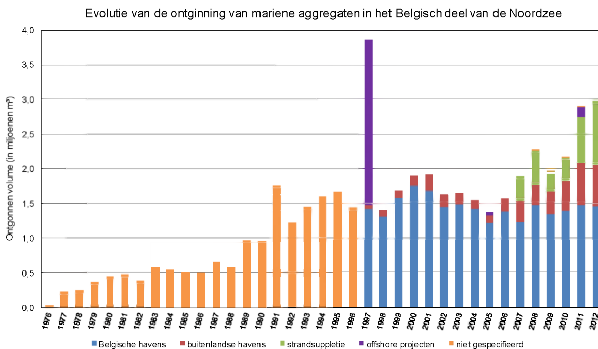
Figuur 30: Aggregaatextractie in het BNZ (1976-2012) [Bron: FOD Economie, januari 2013 (niet-gepubliceerd)]
