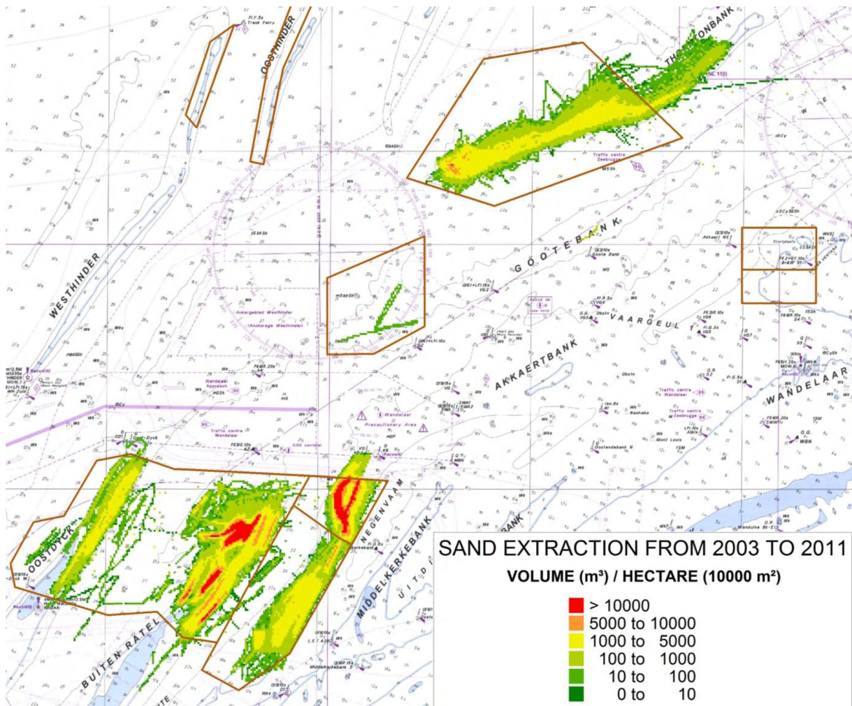
Figuur 31: Ontgonnen volumes in de periode 2003-2011 [Bron: FOD Economie, januari 2013 (niet gepubliceerd)]
