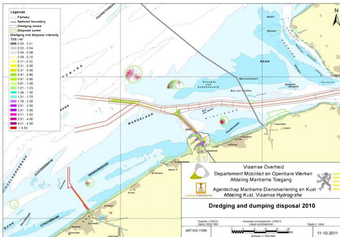
Figuur 28: Bagger- en stortintensiteit in 2010 [Bron: Vlaamse Overheid, Departement Mobiliteit en Openbare Werken, Afdeling Maritieme Toegang, 11-10-2011; Belgische Staat, 2012. Initiële Beoordeling voor de Belgische mariene wateren. Kaderrichtlijn Mariene Strategie – Art 8 lid 1a & 1b. BMM, Federale Overheidsdienst Volksgezondheid, Veiligheid van de Voedselketen en Leefmilieu, Brussel, België, 81 pp., 52].
