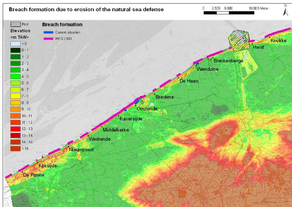
Figuur 53: Locatie van bresvorming door erosie van strand en duinen voor een gemiddelde herhalingstijd van 1 keer op de 17 000 jaar vergeleken bij het huidige zeeklimaat en bij een worst case scenario tegen 2100
