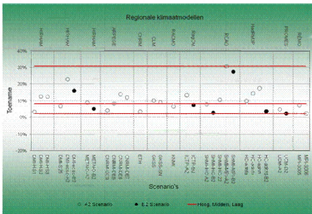
Figuur 7: Percentage neerslagtoename tijdens het winterseizoen voor uitzonderlijke neerslag
