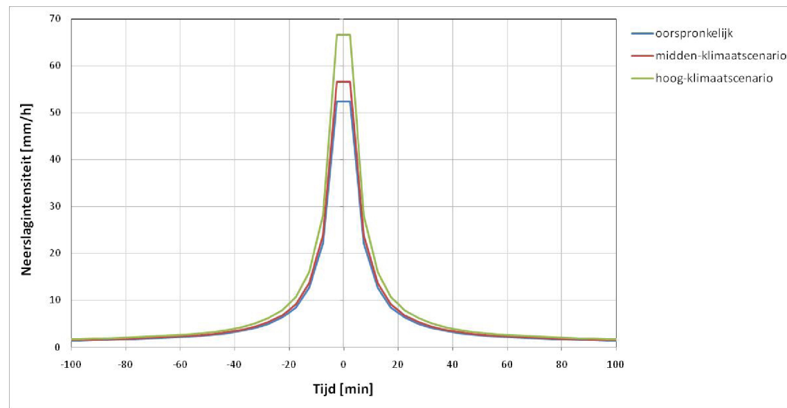
Figuur 34: Aanpassing composietbui bij het hoog- en midden-klimaatscenario voor een terugkeerperiode van 2 jaar (Vlaanderen, scenarioperiode 2071-2100 vergeleken met de controleperiode 1961-1990)
