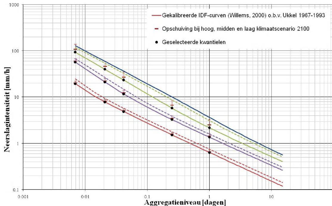
Figuur 33: Opschuiving van de neerslagintensiteiten bij het hoog-, midden- en laag-klimaatscenario voor verschillende aggregatieniveaus en vergelijking met de huidige IDF-verbanden voor verschillende terugkeerperioden
