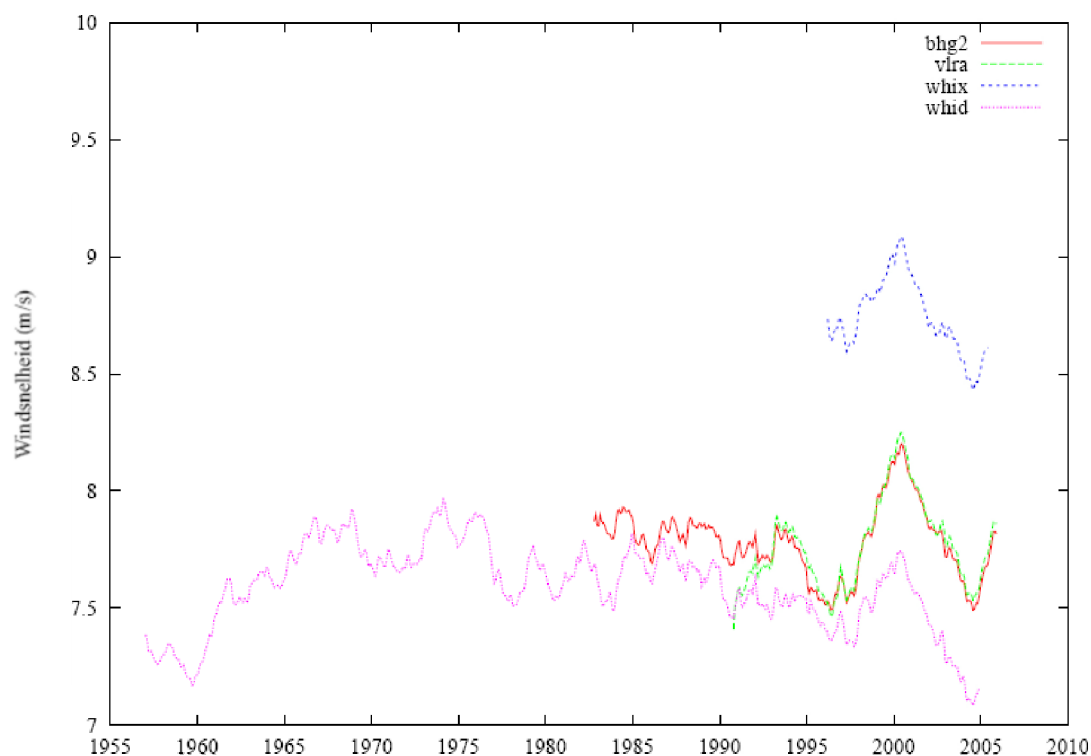
Figuur 29: Langetermijntrend over 48 maanden van de maandelijks gemeten gemiddelde windsnelheid in Brouwershavense Gat 2 (bhg2), Vlakte van de Raan (vlra) en Westhinder (whix) en van de maandelijks gemiddelde windsnelheden van de meteorologische voorspellingen van DNMI in Westhinder (whid)
