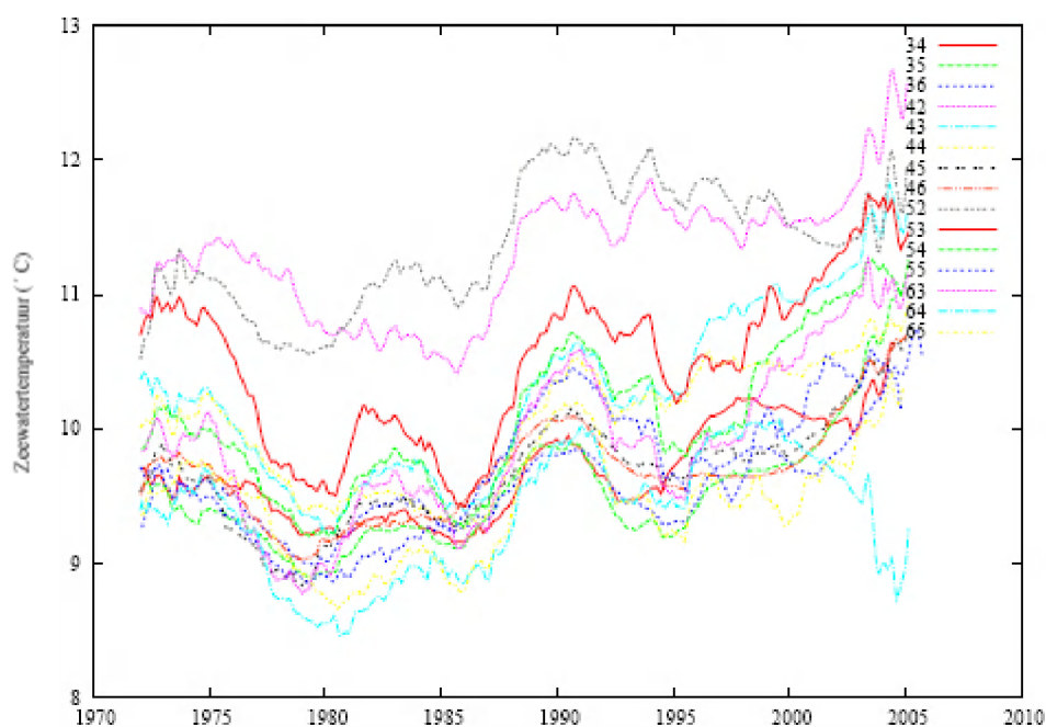
Figuur 27: Langetermijntrend over 48 maanden van de maandelijks gemeten gemiddelde zeewatertemperatuur in de verschillende subgebieden van de Noordzee, berekend met de gegevens, verkregen van de World Ocean Data Base
