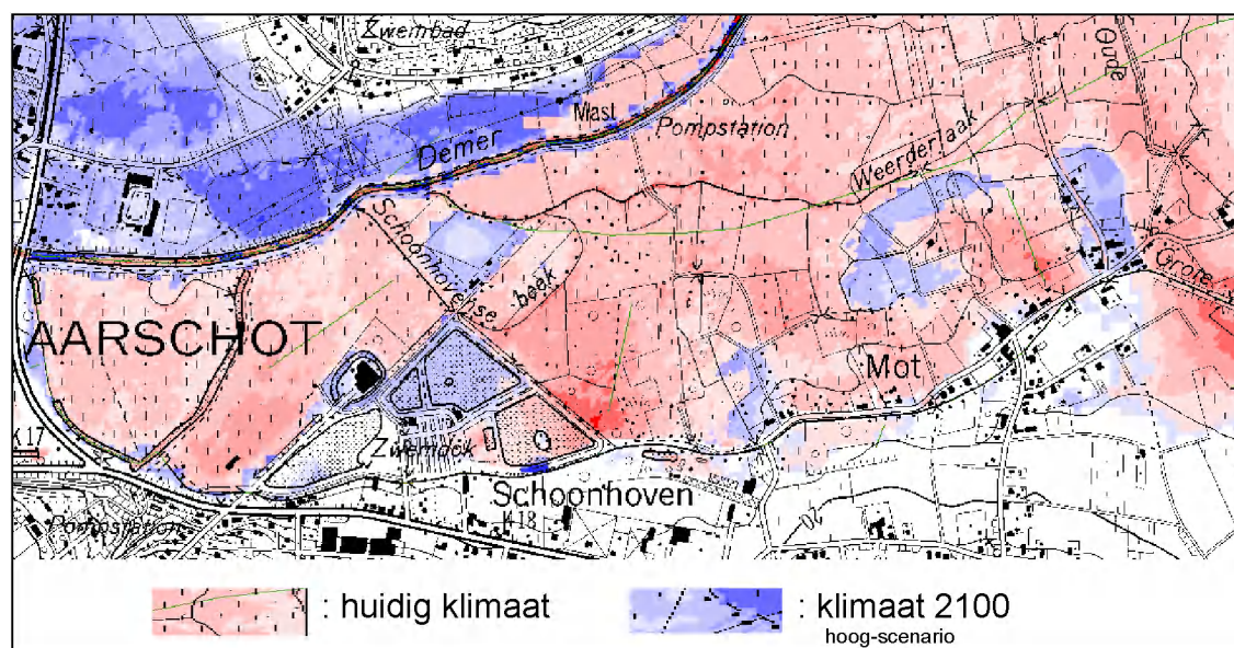
Figuur 32: Lokaal overstroomingsgebied met een gemiddelde herhalingsjijd van 1 keer op de 100 jaar, voor en na het hoog CCI-HYDR klimaatscenario (referentieperiode 1961-1990 tot de scenarioperiode 2071-2100)
