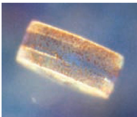
■ Het schijfvormige glazen huisje van het kiezelwier Coscinodiscus , met binnenin talrijke goudbruine bladgroenkorrels of chloroplasten (PAE)
