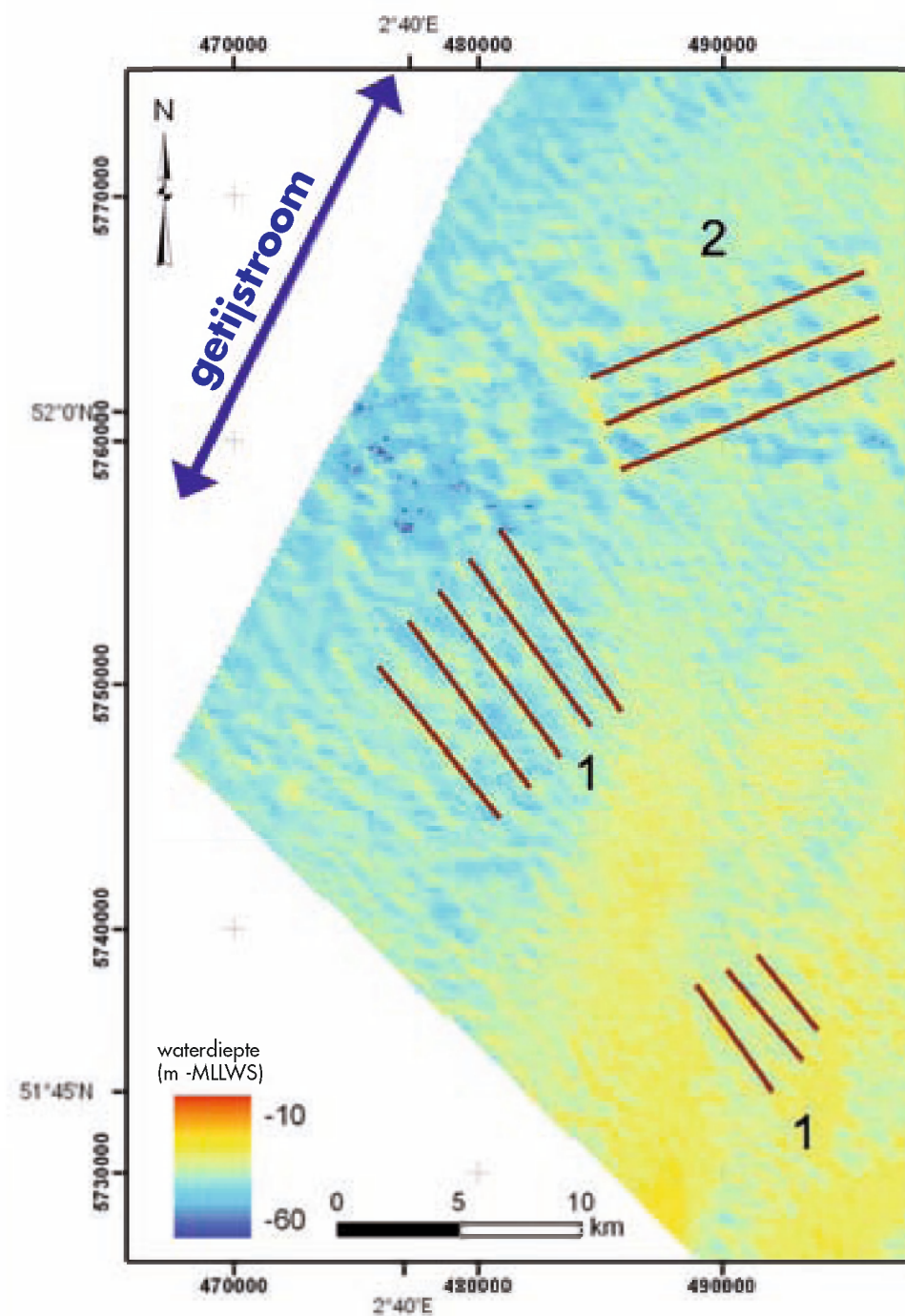
Op deze diepte kaart van een deel van de Noordzee zijn lange bodemgolven (bruine lijnen) te herkennen. Ze komen hier zowel voor met een oriëntatie van 65° in tegenwijzerszin t.o.v. de getijstroom (1) als 30° in wijzerszin (2) (figuur gebruikt met permissie van T. van Dijk – Deltares).
