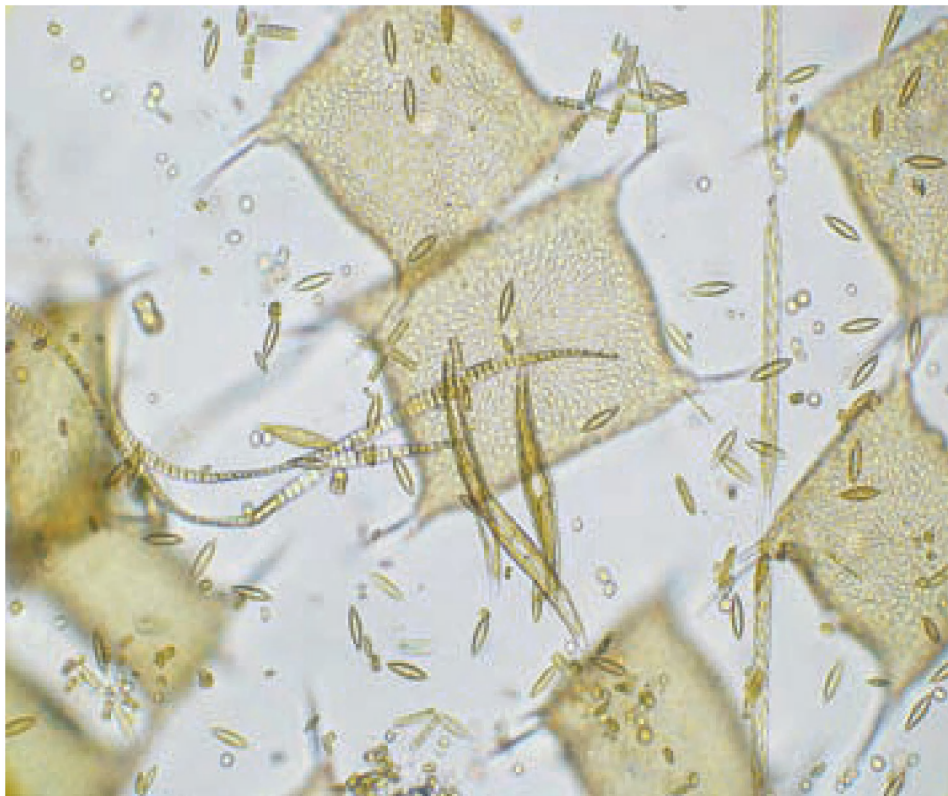
■ Vormenrijkdom van kiezelwieren zoals te vinden voor de Belgische kust (PAE)
