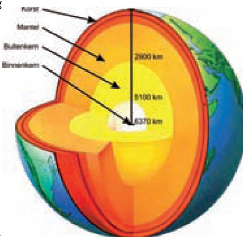
■ Van binnen naar buiten bestaat de aarde uit een vaste binnenkern, een vloeibare buitenkern, een plastische mantel van visceus gesteente en een vaste, hierop drijvende korst (Wikipedia)
