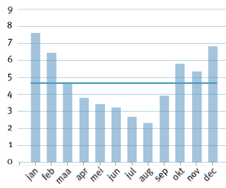
■ Westhinder 1990 - 2004 — Gemiddelde Westhinder (4,64 kW/m) ■ Maandelijks variatie van het beschikbaar golfvermogen ter hoogte van de Westhinder (1990-2004)(AWW)
