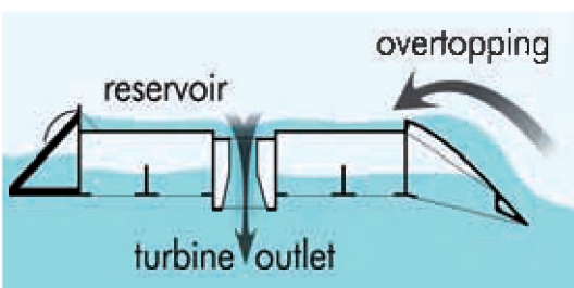
■ Weringsprincipe van de Wave Dragon (copyright: Wave Dragon)
