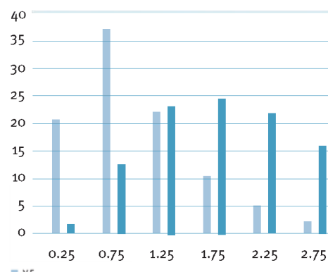
■ V.F. ■ Bijdrage tot het jaarlijks gemiddeld golfvermogen ■ Voorkomingsfrequentie (V.F.) en bijdrage tot het gemiddeld jaarlijks beschikbaar golfvermogen van verschillende golfhoogtes ter hoogte van de Westhinder (1990-2004)(AWW)
