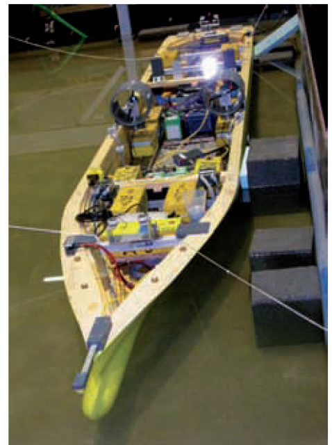
■ Ontwerp van nieuwe sluizen voor het Panama kanaal: Schaalmodelstudie (schaal 1:80) in het Waterbouwkundig Laboratorium te Borgerhout in opdracht van de Autoridad del Canal de Panamá. Zicht op het ontwerpschip (met een capaciteit van 12.000 twintig-voet-containers) met instrumentatie (WL)
