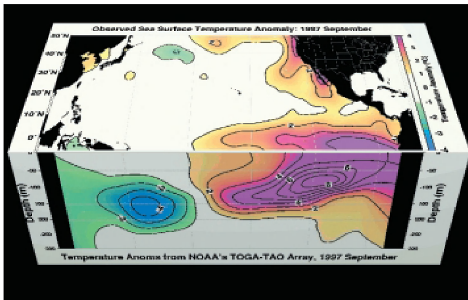
Bij een El Niño warmt het oppervlaktewater van de oostelijke Stille Oceaan tijdelijk op, met verstrekkende en wereldomvattende gevolgen voor klimaat, mens en ecosysteem (NOAA)
