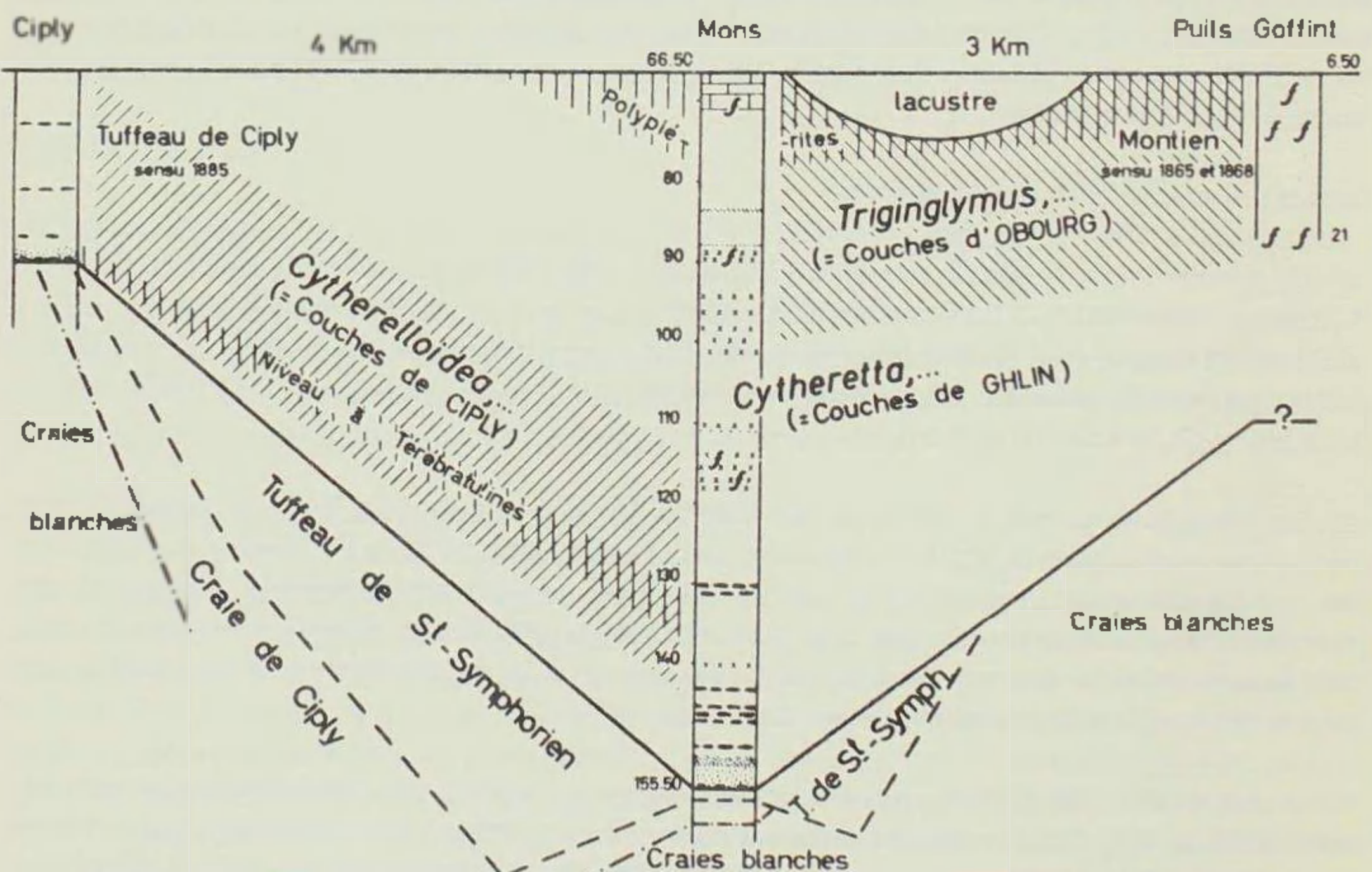
FIGURE 1 - Diagramme comparatif montrant les relations entre le Calcaire grossier de Mons (puits Goffint), le Tuffeau de Ciplly (craie de Ciplly). La superposition est démontrée à Mons dans la partie axiale du bassin. (Reproduction du diagramme figuré dès 1957, complété par la nomenclature en couches de Ciplly, Couches de Ghlin, Couches d'Obourg.)
