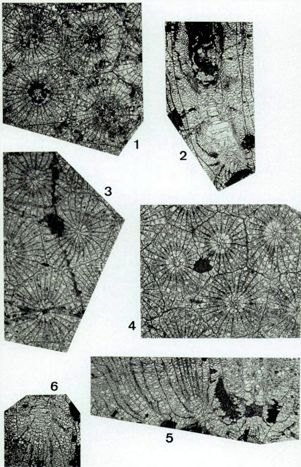
M. COEN-AUBERT. — Représentants des genres Phillipsastrea D'ORBIGNY, A., 1849, Billingsastraea GRABAU, A. W., 1917 et Iowaphyllum STUMM E. C., 1949 du Frasnien du Massif de la Vesdre et de la bordure orientale du Bassin de Dinant.
