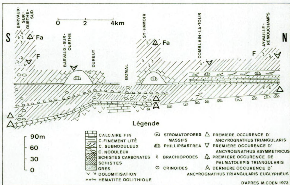
Fig. 4. — Variations faciales de la partie supérieure du Frasnien le long de la bordure orientale du Bassin de Dinant
