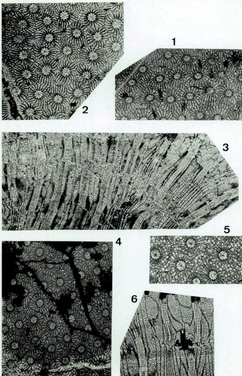
M. COEN-AUBERT. — Représentants des genres Phillipsastrea D'ORBIGNY, A., 1849, Billingsastrea GRABAU, A. W., 1917 et lowapophyllum STUMM E. C., 1949 du Frasnien du Massif de la Vesdre et de la bordure orientale du Bassin de Dinant.
