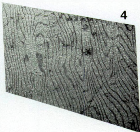
M. COEN-AUBERT. — Représentants des genres Phillipsastrea D'ORBIGNY, A., 1849, Billingsastraea GRABAU, A. W., 1917 et Iowaphyllum STUMM E. C., 1949 du Frasnien du Massif de la Vesdre et de la bordure orientale du Bassin de Dinant.
